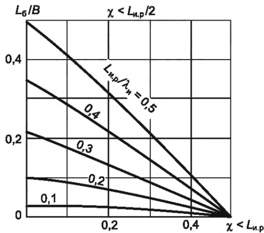
Рисунок 10.6 — Графики относительного поперечного размыва выпуклого берега в зависимости от расстояния проектного створа до вершины излучины при различных темпах смещения излучины
