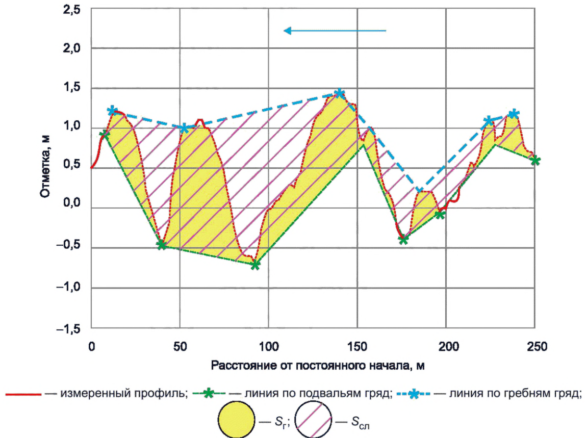
Рисунок 13.3 — Схема расчета среднего коэффициента формы гряд \bar{m}_r
