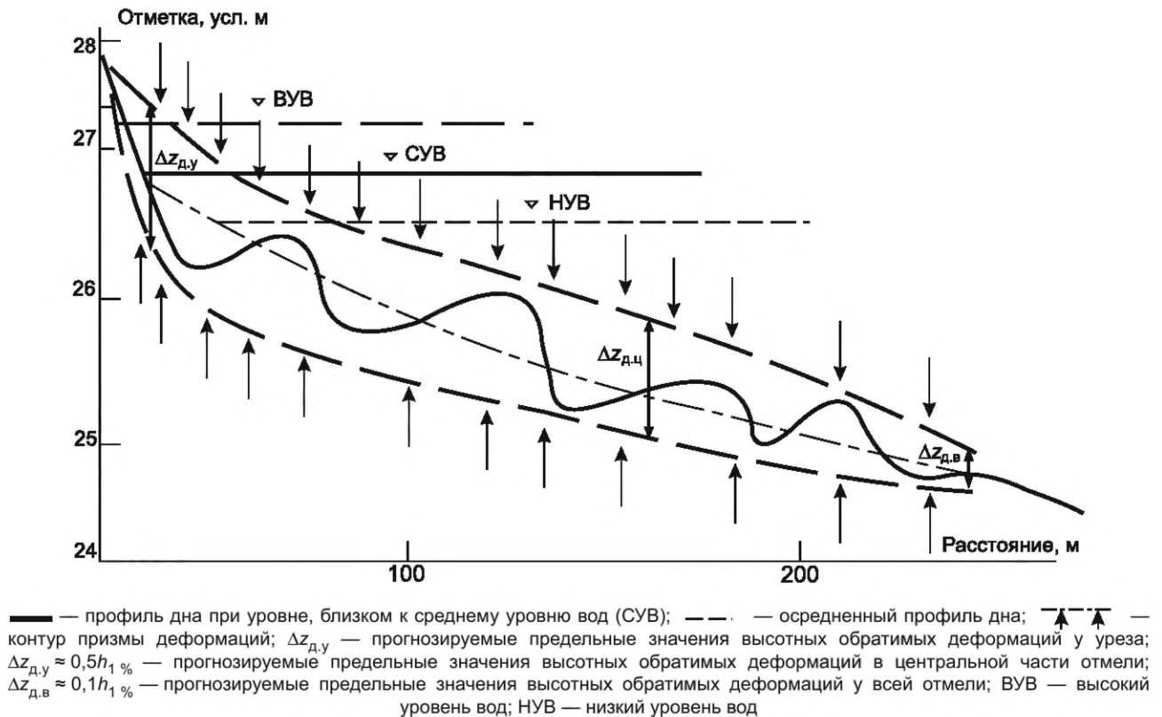
Рисунок 14.5 — Построение контура высотных деформаций дна береговой отмели (вертикальные стрелки) по осредненному профилю створа перехода МН по рассчитанным значениям деформаций в различных частях отмели
