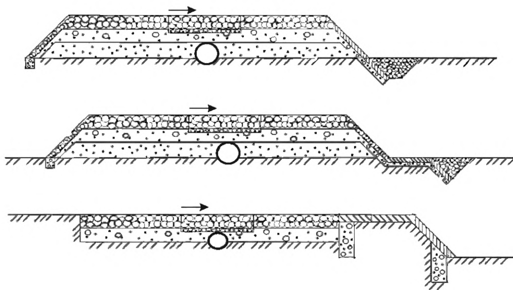
Рисунок 15.1 — Принципиальные схемы площадного крепления речного дна над МТ в пределах речных русел
