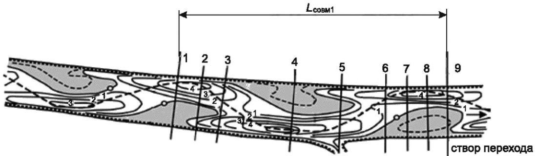
Рисунок 10.1 — Схема расположения совмещаемых поперечников при побочневом типе руслового процесса
