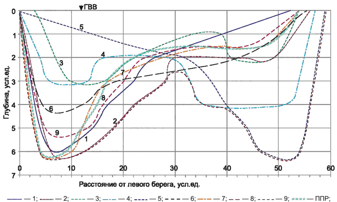
Рисунок 10.1 — Схема расположения совмещаемых поперечников при побочневом типе руслового процесса
