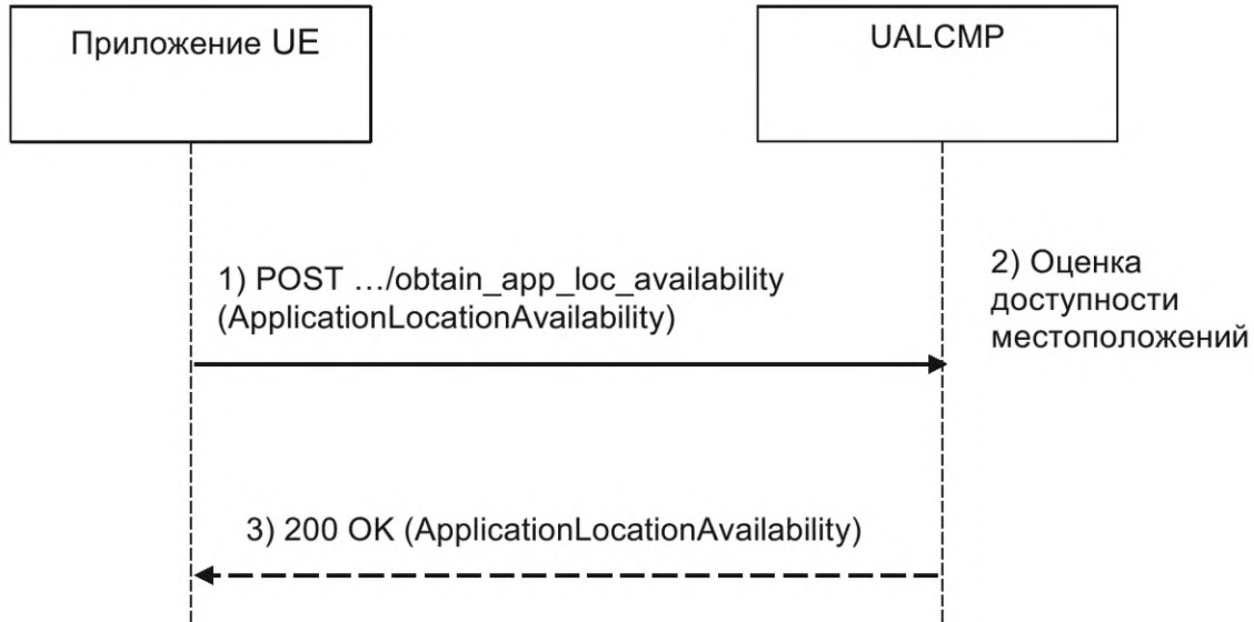
Рисунок 6 — Процесс предоставления точки M×2 в системе MEC
