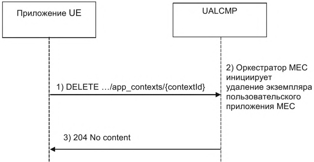
Рисунок 3 — Процесс удаления экземпляра пользовательского приложения MEC
