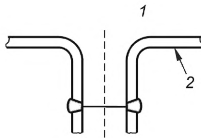
Рисунок D.19 — Типовое двустороннее стыковое сварное соединение
