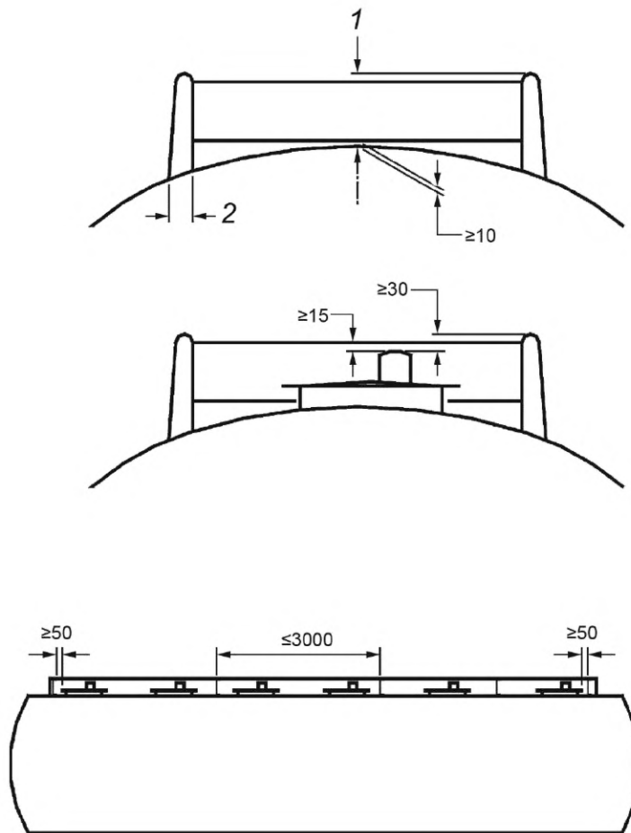
1 — высота продольного защитного элемента над верхней частью корпуса (измеряют по верхней части осевой линии корпуса); 2 — ширина продольного защитного элемента (измеряют у его основания) — не менее одной трети высоты
