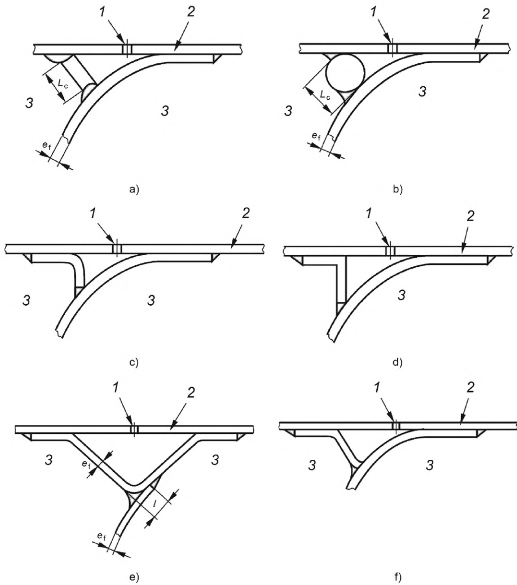
Рисунок D.11 — Типовые усиленные соединения
