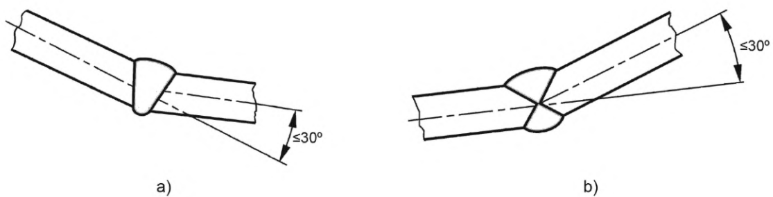
Рисунок D.9 — Типовые угловые сварные соединения
