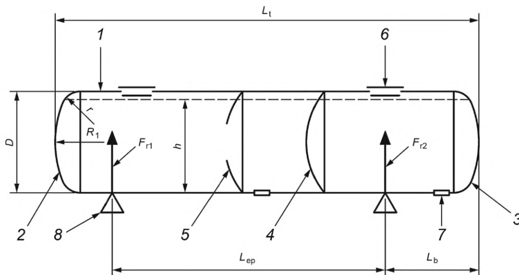
1 — стенка корпуса; 2 — переднее днище; 3 — заднее днище; 4 — перегородка; 5 — волногасящая переборка; 6 — верхнее отверстие; 7 — нижнее отверстие; 8 — опоры
