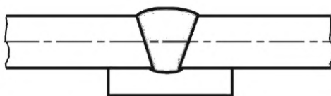
Рисунок D.5 — Типовое стыковое сварное соединение с подкладкой
