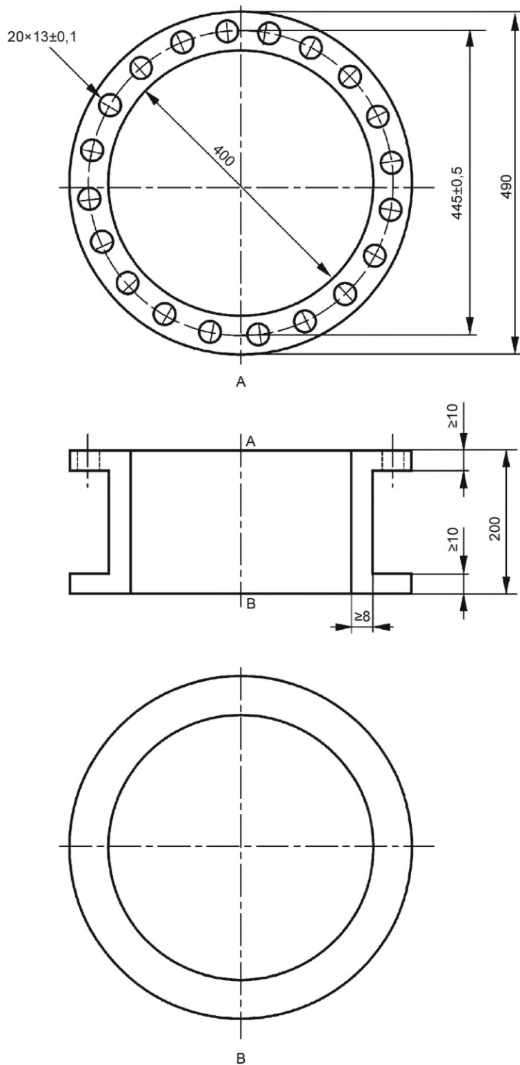
Рисунок В.1 — Опорное приспособление для установки испытуемого образца
