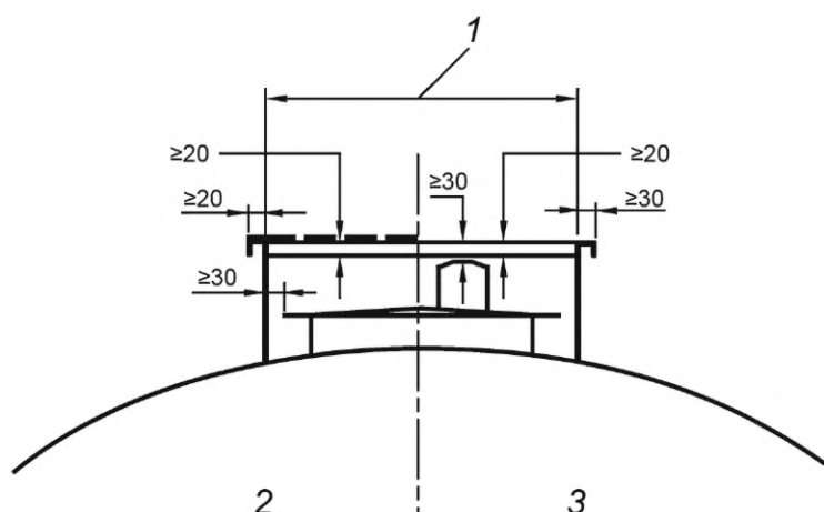
1 — ширина, диаметр не более 900 мм, длина (если прямоугольный) не более 1 500 мм; 2 — лоток для сбора жидкостей с крышкой; 3 — лоток для сбора жидкостей без крышки
