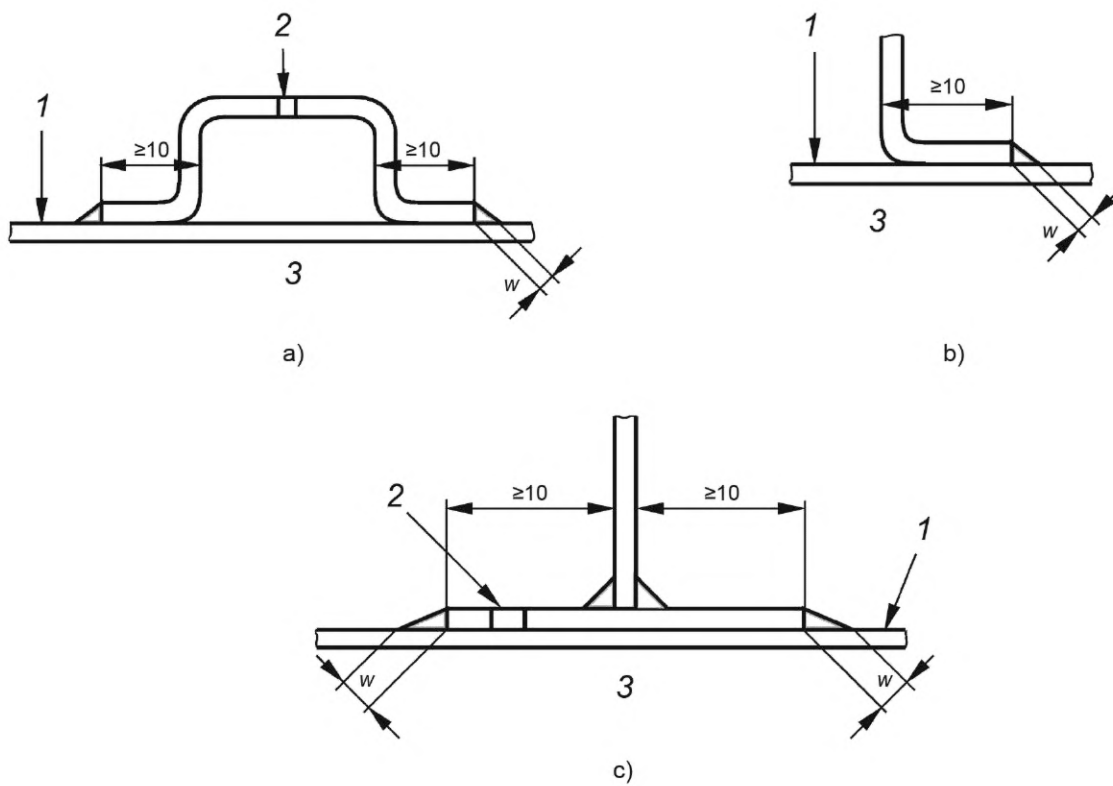
Рисунок D.15 — Типовые примеры соединений пластин днища с корпусом
