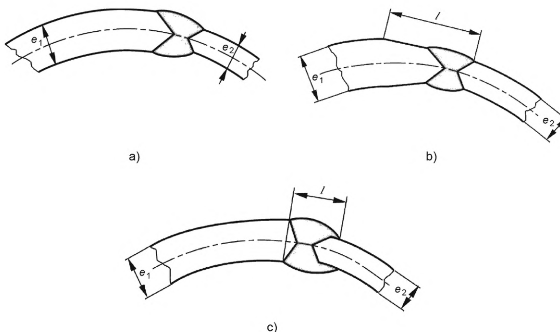
Рисунок D.3 — Типовые примеры стыковых сварных соединений с пластинами разной толщины
