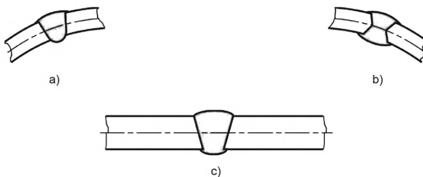
Рисунок D.2 — Типовые примеры стыковых сварных соединений с пластинами одинаковой толщины
