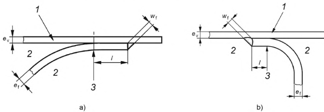
Рисунок D.11 — Типовые усиленные соединения
