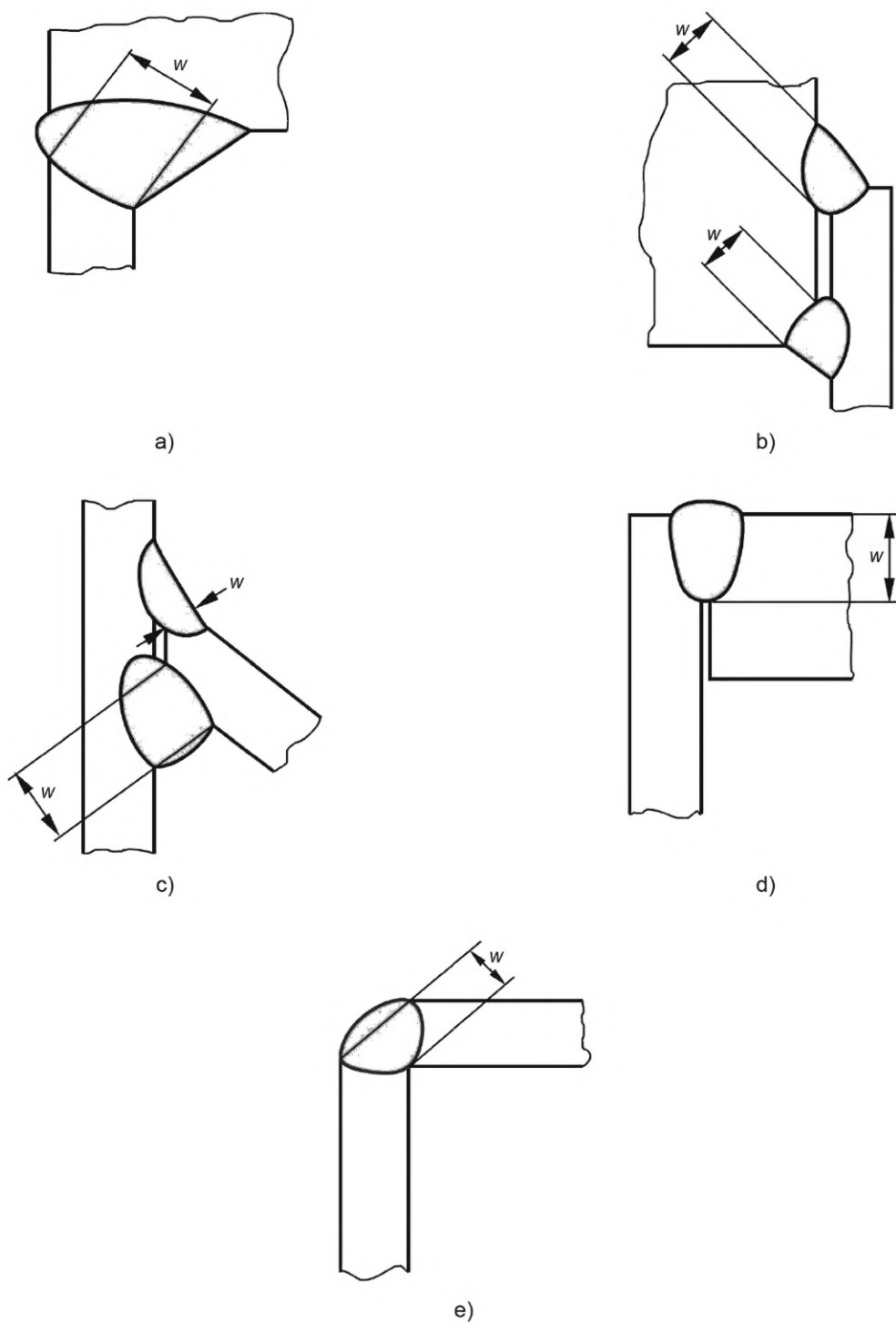
Рисунок D.1 — Типовые примеры эффективной глубины угловых сварных швов
