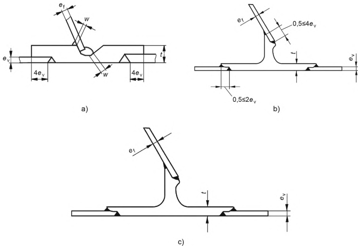
Рисунок D.14 — Типовые соединения перегородок
