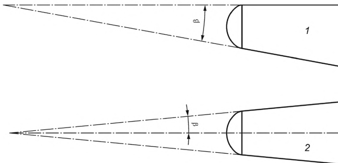
1 — клиновидный участок; 2 — конусообразный участок
