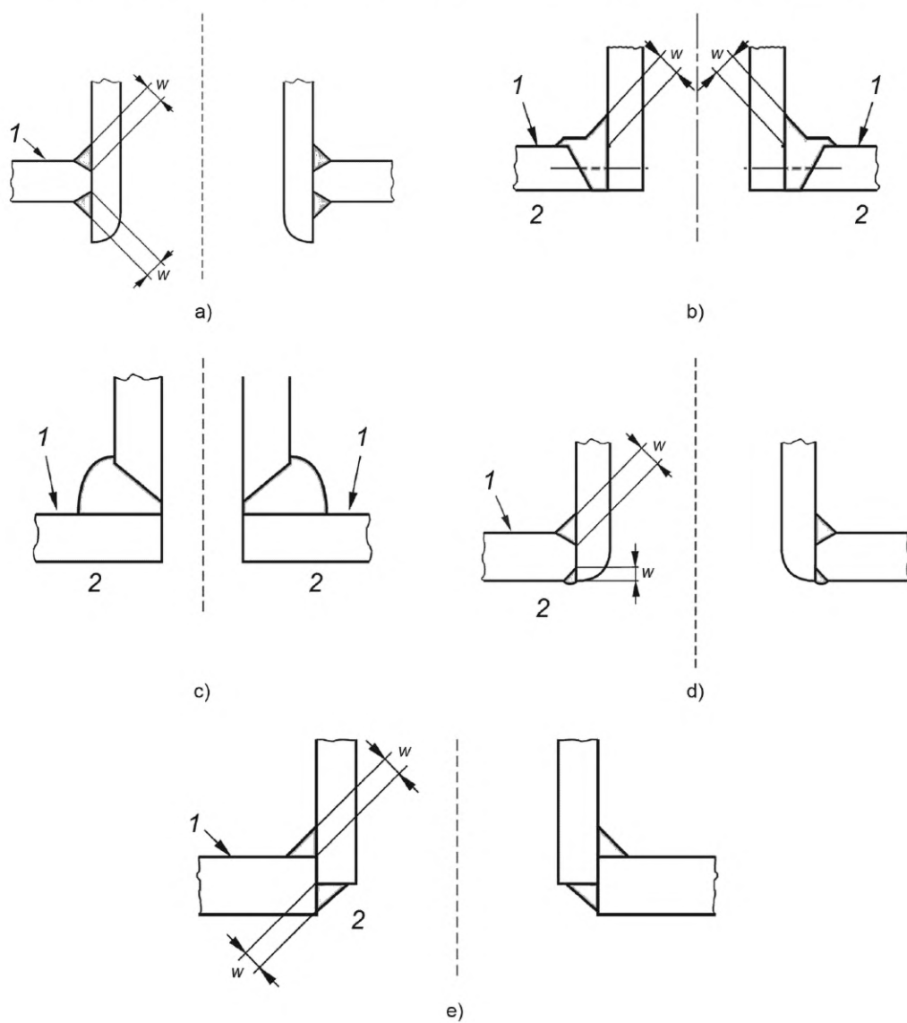
Рисунок D.17 — Типовые соединения непоглощающих усилительных элементов
