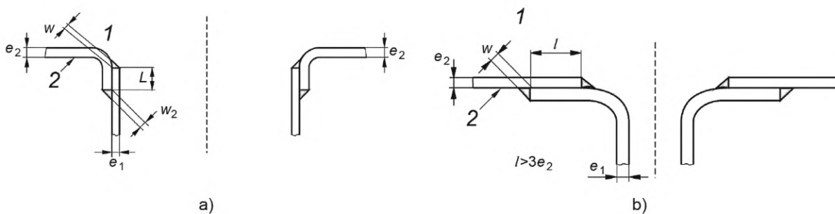
Рисунок D.19 — Типовое двустороннее стыковое сварное соединение
