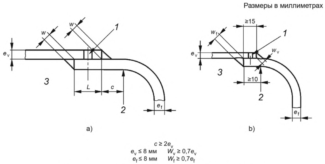
Рисунок D.7 — Типовые нахлесточные сварные соединения днища с корпусом
