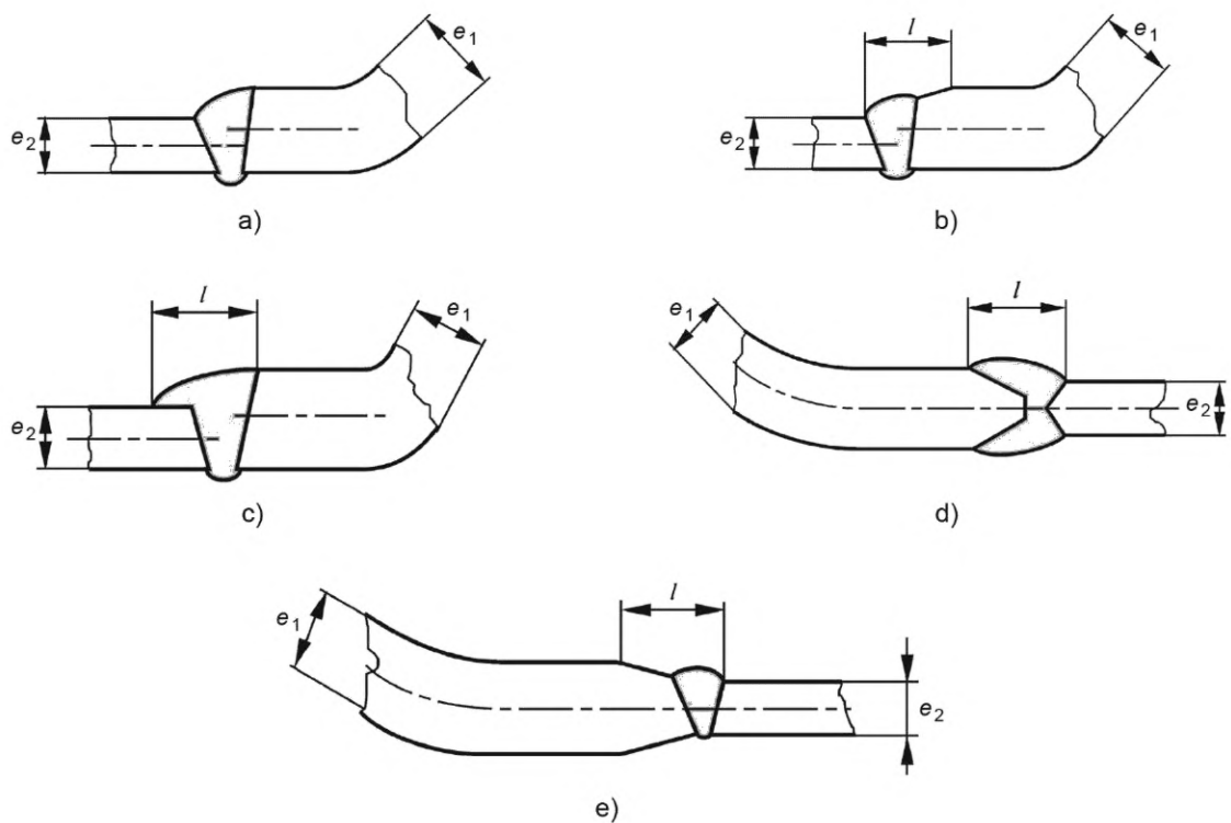
Рисунок D.4 — Типовые примеры стыковых сварных соединений корпуса с днищем
