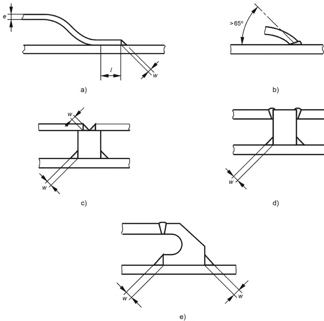
Рисунок D.23 — Типовые крепежные соединения нагревательных каналов с корпусами
