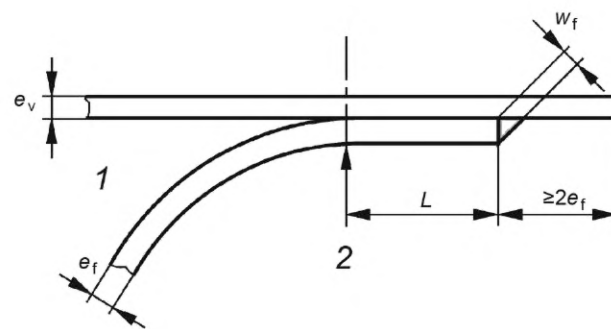
Рисунок D.7 — Типовые нахлесточные сварные соединения днища с корпусом
