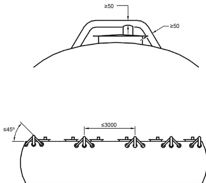
Рисунок 4 — Типовое расположение рабочего оборудования, защищенного дугами безопасности
