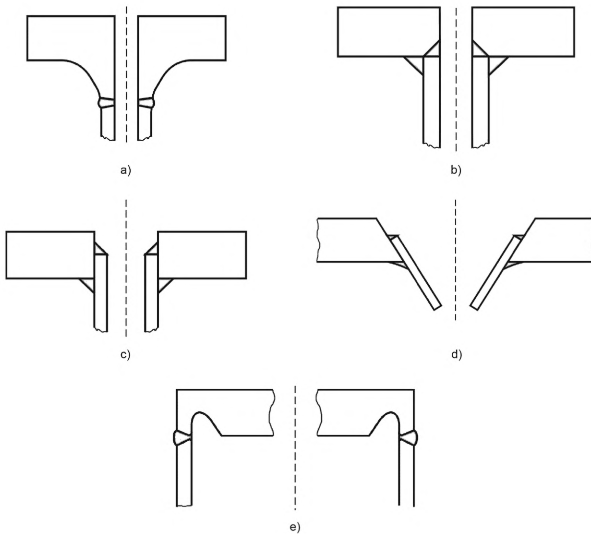
Рисунок D.22 — Типовые крепежные соединения фланцев с патрубками
