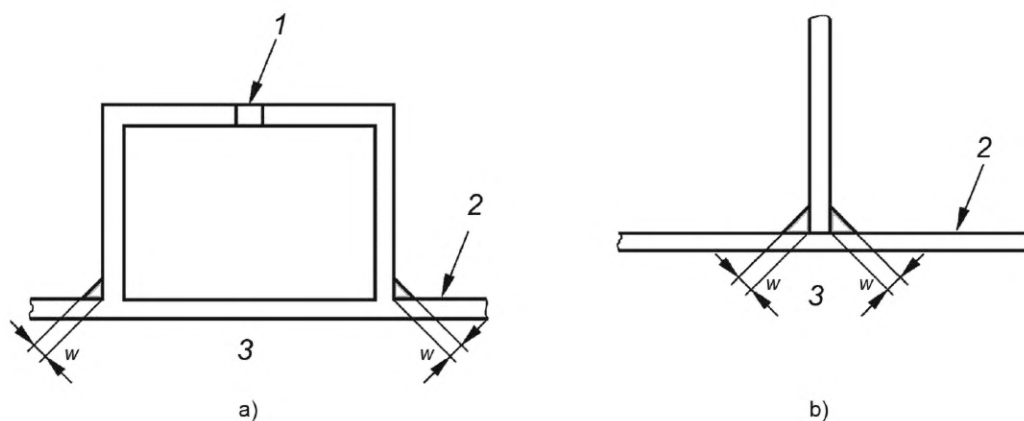
Рисунок D.17 — Типовые соединения непоглощающих усилительных элементов
