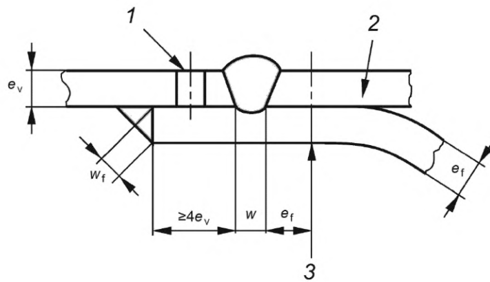
Рисунок D.13 — Типовое сварное соединение с двусторонним швом
