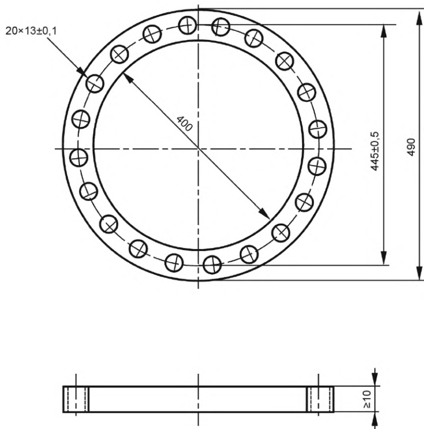
Рисунок В.2 — Зажимное кольцо
