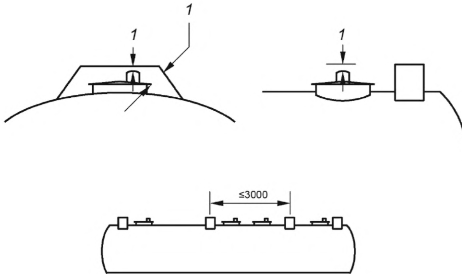
Рисунок 5 — Типовое расположение рабочего оборудования, защищенного поперечными элементами коробчатого сечения
