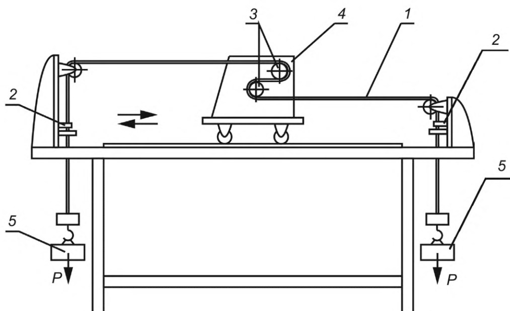
1 — испытываемый образец; 2 — ограничивающие зажимы; 3 — сменные ролики; 4 — каретка; 5 — грузы
