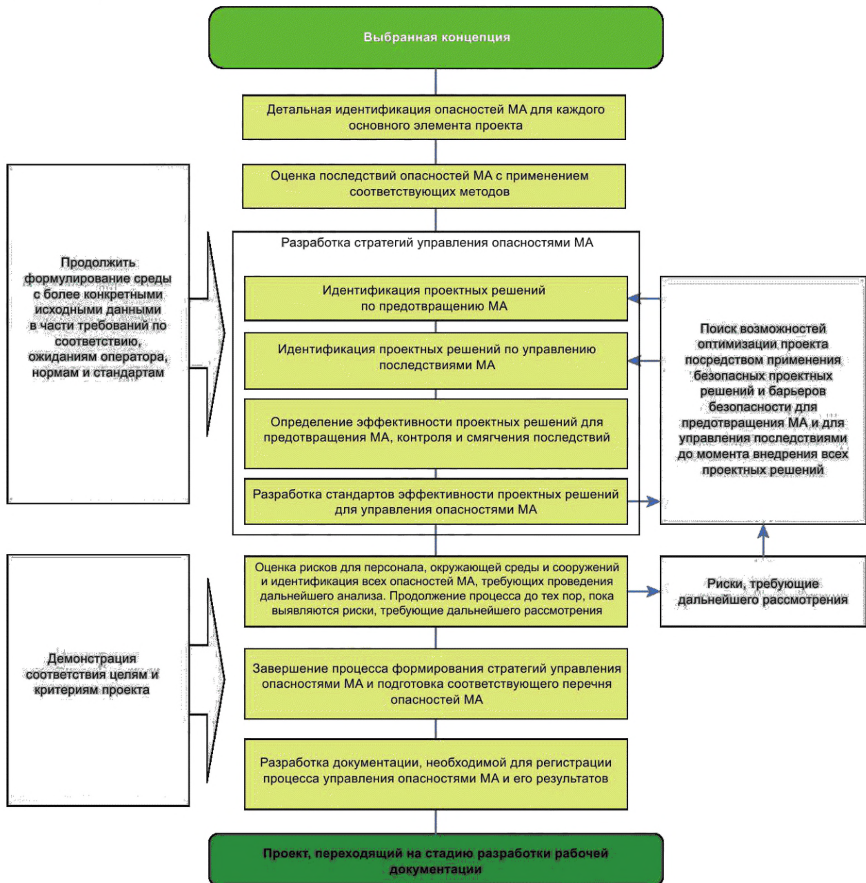
Рисунок 3 — Блок-схема процесса управления опасностями МА на стадии разработки предпроектной и проектной документации
