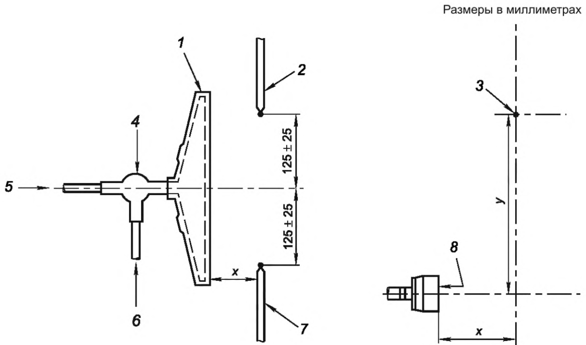
1 — горелка; 2 — термопара А; 3 — кончик термопары; 4 — смеситель Вентури; 5 — подача воздуха; 6 — подача пропана; 7 — термопара В; 8 — фронтальная поверхность рабочей части горелки
