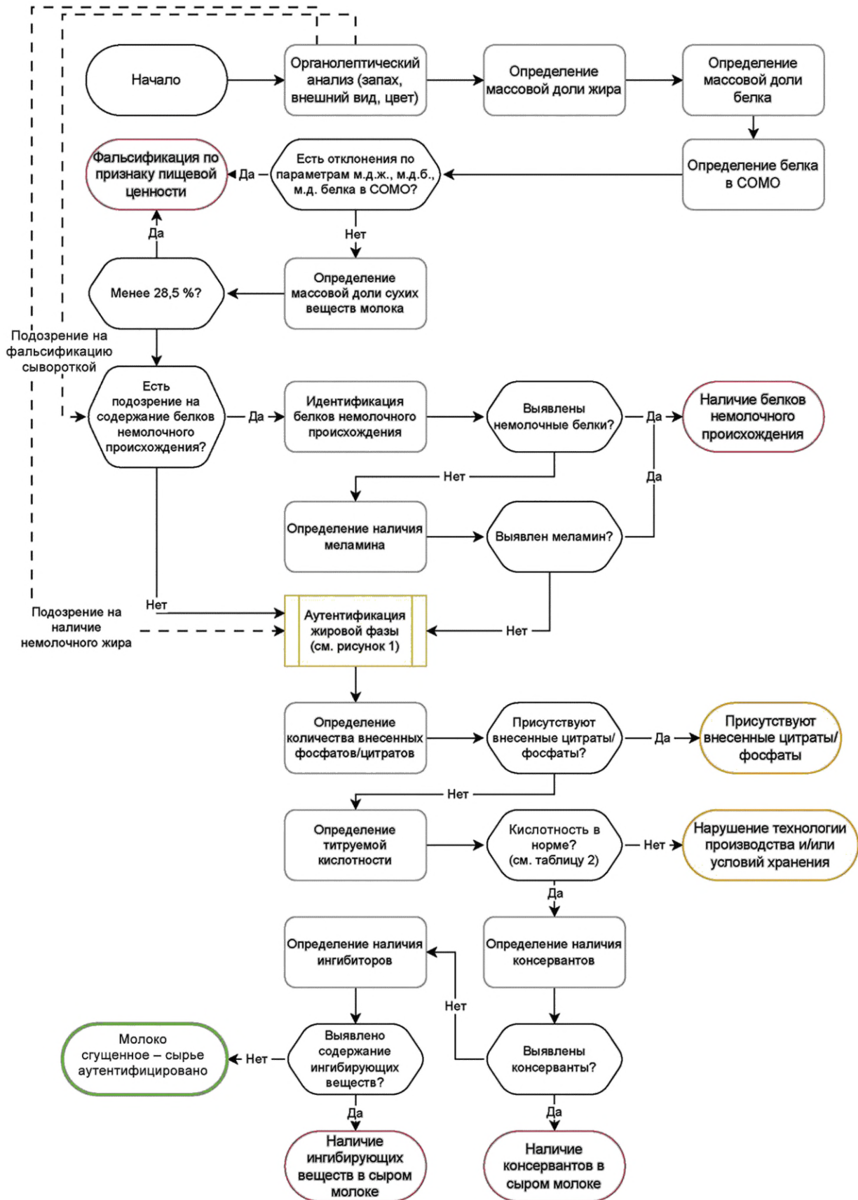
Рисунок 4 — Схема алгоритма аутентификации молока сгущенного — сырьё
