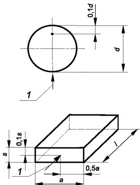
1 — направление измерения разности хода; d — диаметр заготовки; a — ширина заготовки; s — толщина заготовки; l — длина заготовки
