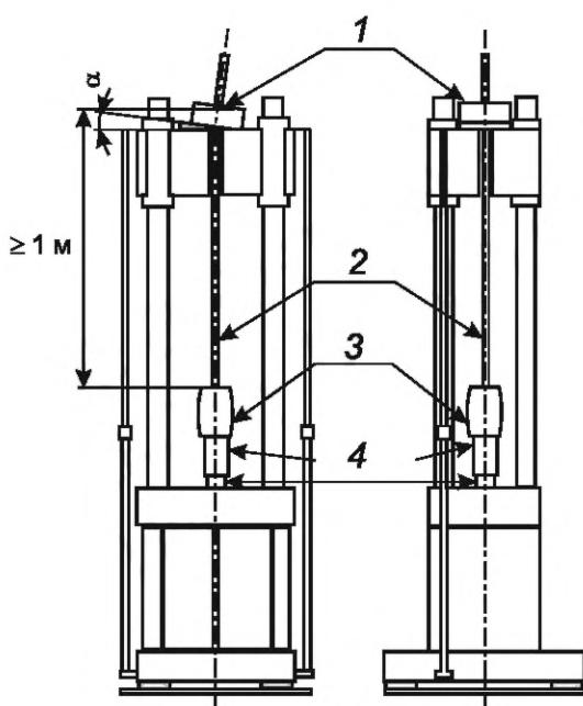
1 — обойма; 2 — прядь; 3 — захват; 4 — датчик усилия
