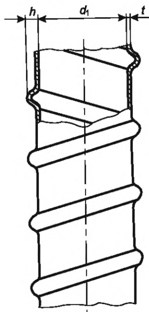
Рисунок И.1 — Геометрические параметры каналообразователя
