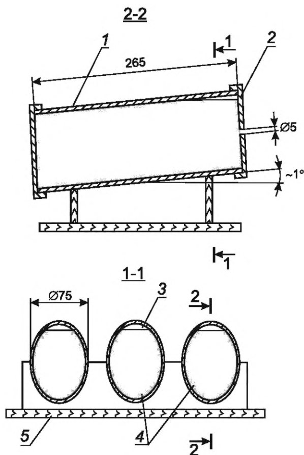
Рисунок К.2 — Схема испытания на оседание
