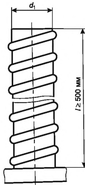
Рисунок И.2 — Образец для определения относительного объема гофрированной части
