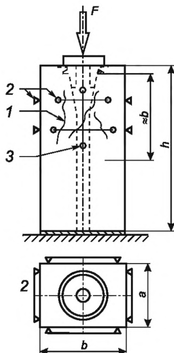
1 — трещина; 2 — база измерения поперечной относительной деформации; 3 — база измерения продольной относительной деформации
