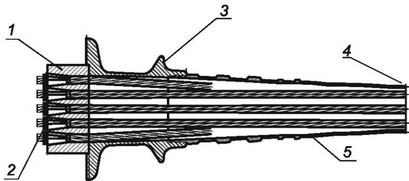
Рисунок 5.4 — Эскиз варианта анкера с опорным стаканом и клиновыми зажимами
