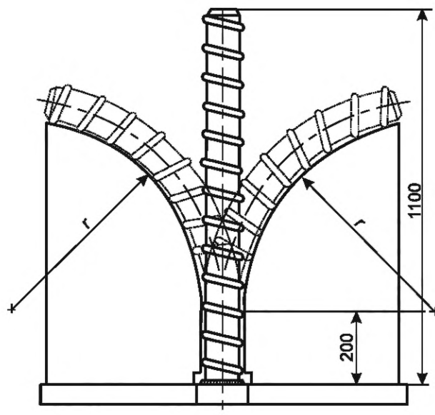
Рисунок И.5 — Схема стенда для проверки гибкости
