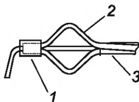
1 — втулка; 2 — каркас из проволок пряди; 3 — прядь
