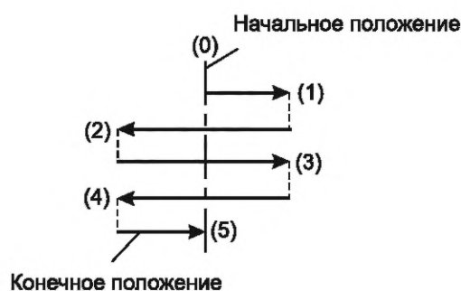
Рисунок И.6 — Порядок отгиба каналобразователя
