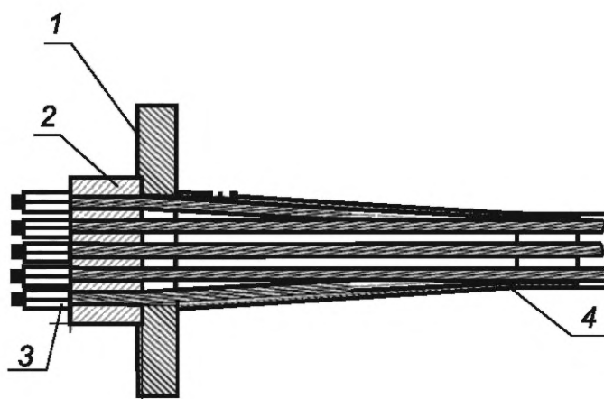
Рисунок 5.5 — Эскиз варианта анкера с опорной плитой и обжимными муфтами
