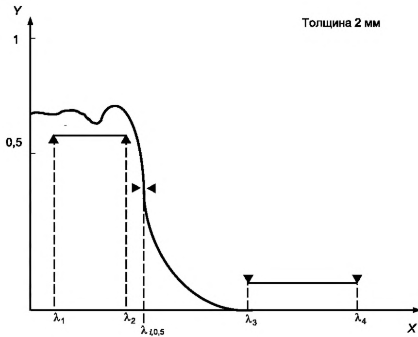
Рисунок 6 — Графическое представление спектральной характеристики коротковолново-пропускающего фильтра SP
