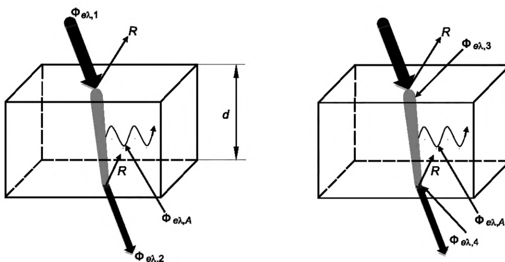
R — отражение от поверхности; d — толщина оптического фильтра объемного поглощения
