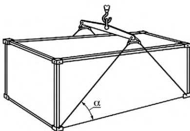
Рисунок 11 — Зацепка грузового контейнера линейной поперечной траверсой за нижние угловые фитинги
