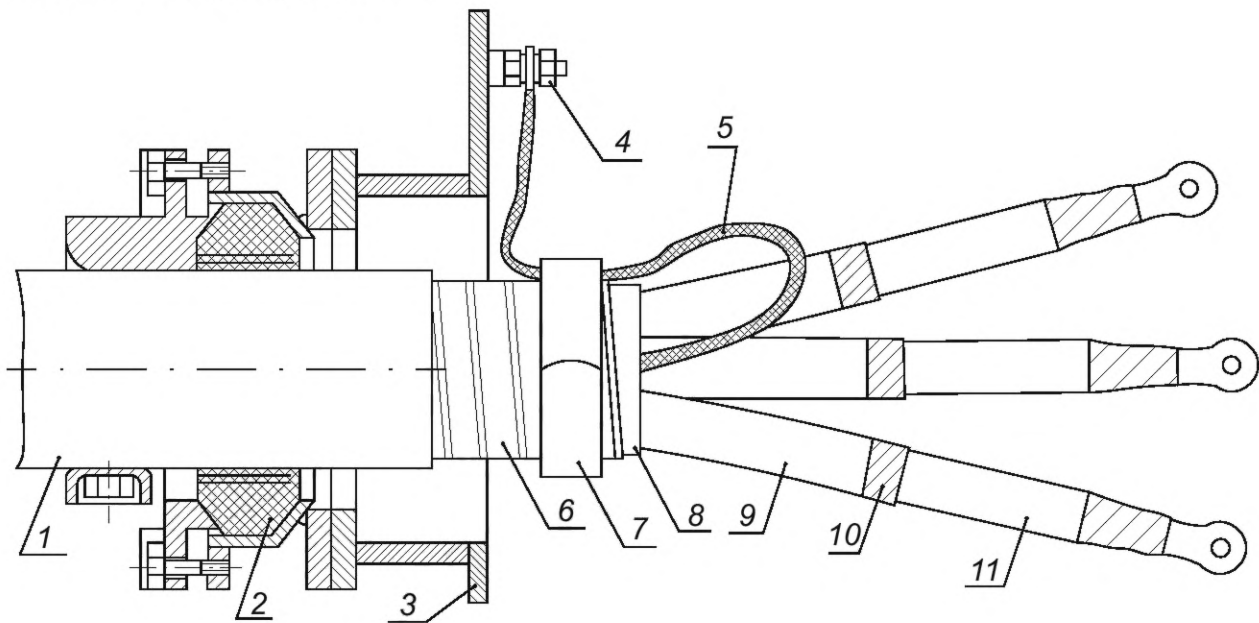
1 — наружная оболочка кабеля; 2 — уплотнительное кольцо; 3 — корпус; 4 — внутренний заземляющий зажим; 5 — жила заземления; 6 — броня кабеля; 7 — кольцо постоянного давления; 8 — внутренняя оболочка; 9 — экраны основных токопроводящих жил из медной ленты; 10 — ленточный бандаж экрана; 11 — изоляция жилы
