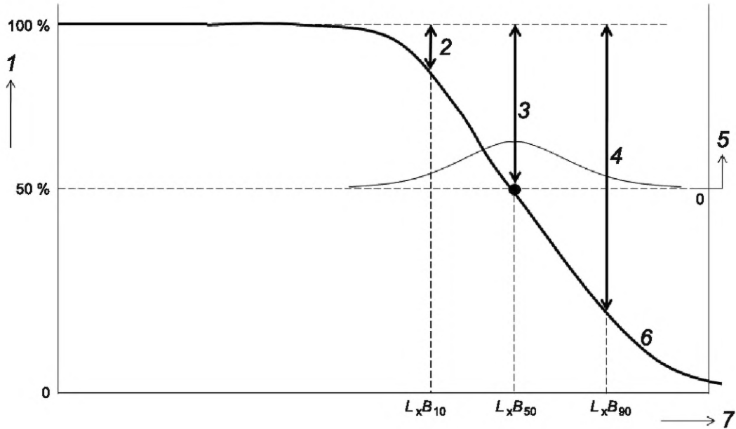
1 — R(t) ; 2 — 10 % отказов; 3 — 50 % отказов; 4 — 90 % отказов; 5 — pdf_x ; 6 — R_{\text{постепенное}} за L_x ; 7 — время работы t , ч
