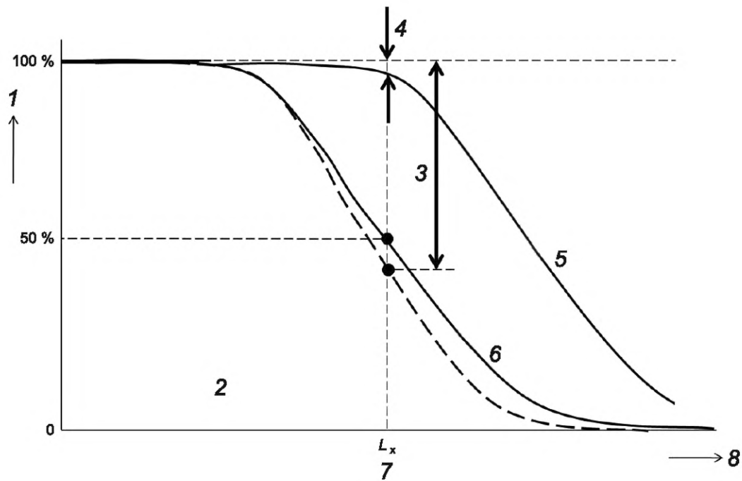
1 — R(t) ; 2 — R_{\text{общее}} = R_{\text{постепенное}_x}(t) \cdot R_{\text{внезапное}}(t) ; 3 — CFV; 4 — AFV; 5 — R_{\text{внезапное}}(t) ; 6 — R_{\text{постепенное}_x}(t) ; 7 — средний ресурс; 8 — время работы t , ч
