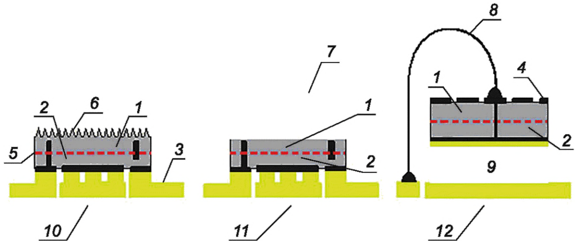
а) Тонкопленочный перевернутый СД кристалл
