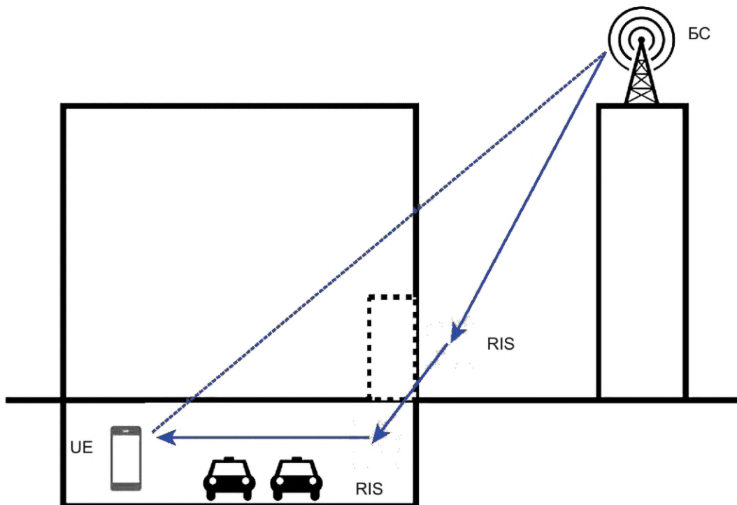
Рисунок 8 — Использование RIS для улучшения покрытия в сценарии, когда БС, расположенная на улице, обслуживает UE, которое находится в помещении
