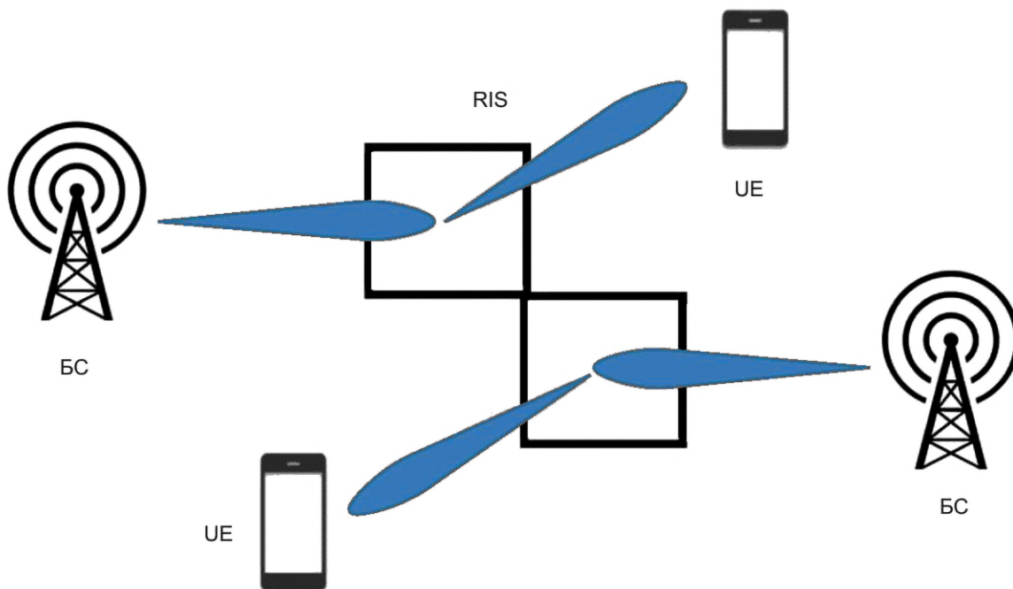
Рисунок 10 — Пример множественного доступа к радиосети с RIS
