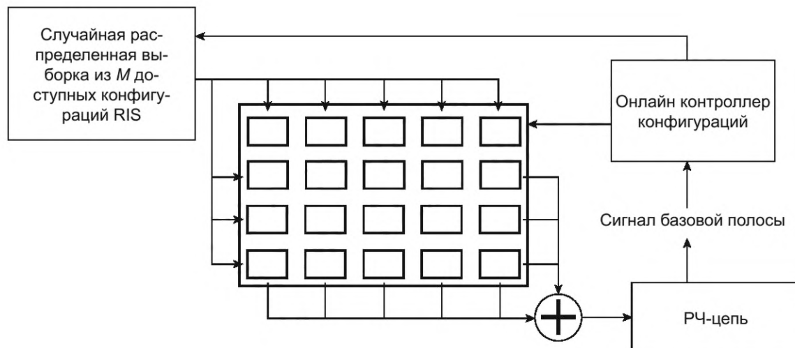
Рисунок 3 — Структурная схема аппаратной архитектуры RIS, включающая в себя одну активную РЧ-цепь приема, обеспечивающую обнаружение принимаемого сигнала в базовой полосе частот
