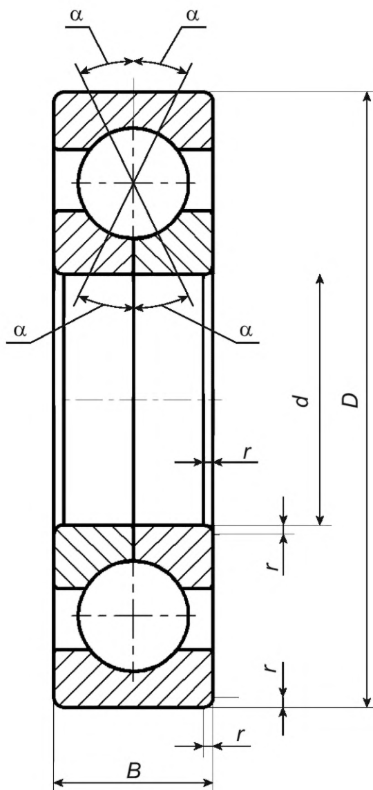
Рисунок 3 — Конструктивные исполнения 17, 59
