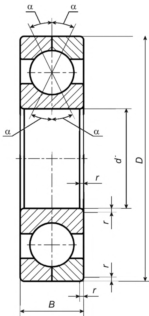
Рисунок 1 — Конструктивное исполнение 11
