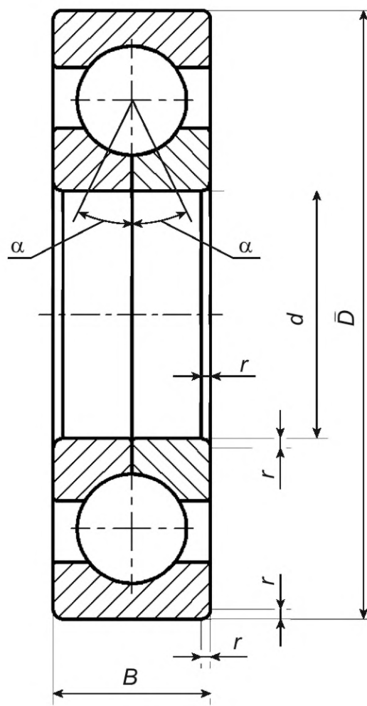
Рисунок 2 — Конструктивное исполнение 12
