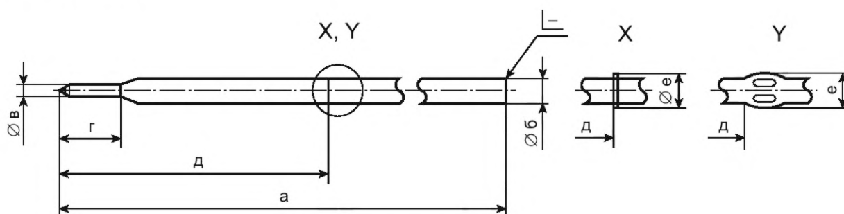
Рисунок 1 — Типы стержней A_1 , A_2 и В
