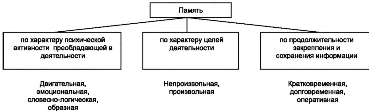
Рисунок 1 — Виды памяти
