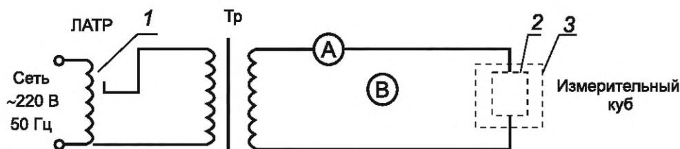
1 — лабораторный регулируемый трансформатор (ЛАТР); 2 — электрод; 3 — измерительный куб
