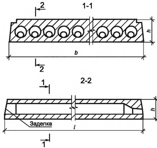
Рисунок 2 — Сечения плиты типа 4ПК
