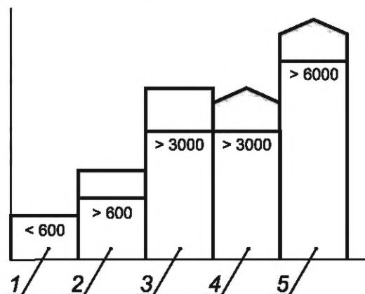
1 — не требуются ограждающие стены; 2 — необходимы ограждающие стены, соответствующие росту пользователя; 3 — необходимы ограждающие стены в 1,25 раза выше роста пользователя; 4 — необходима несъемная крыша; 5 — необходимы ограждающие стены и крыша
