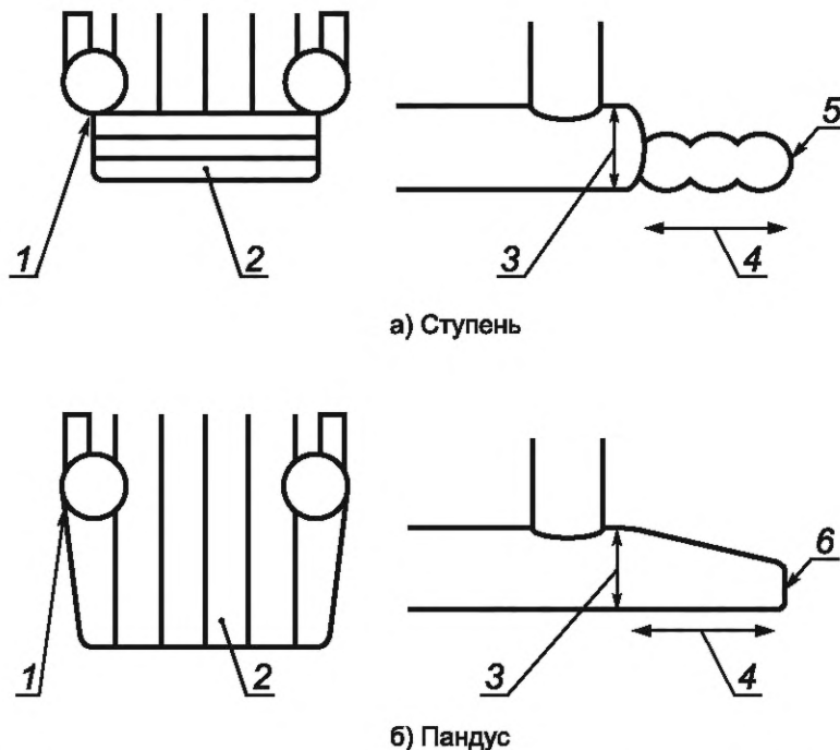
Рисунок 6 — Ступень и пандус
