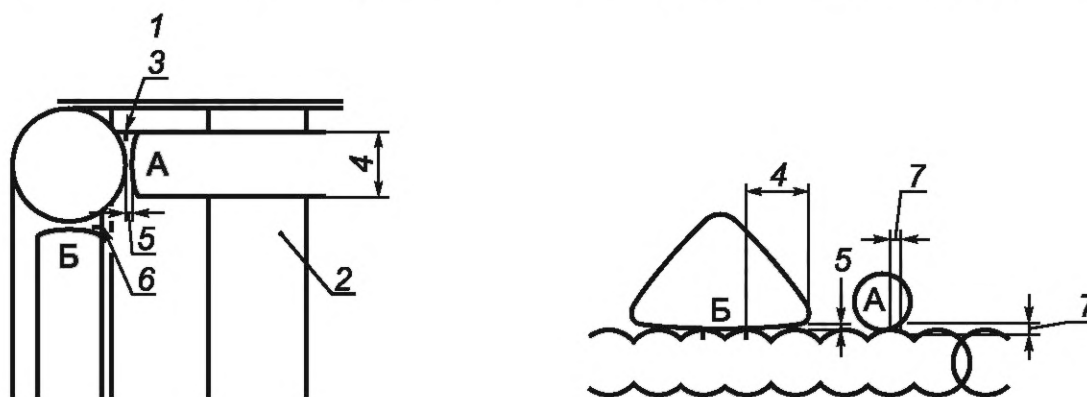
а) Позиция А, образующая место застревания, позиция Б, не образующая места застревания
