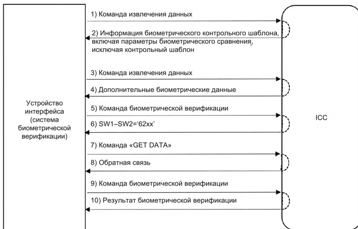
Рисунок 1 — Схема процедуры биометрического сравнения на идентификационной карте с механизмом распределения
