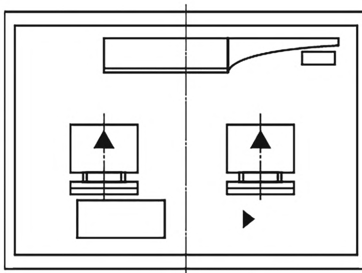
Рисунок И.5 — Размещение точек измерения параметров при проведении испытаний по определению показателей эффективности системы обеспечения микроклимата в операторской СПС
