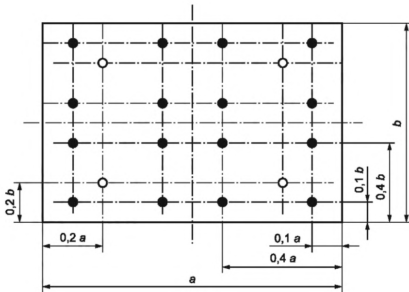
Рисунок М.3 — Координаты точек измерения скоростей в воздуховодах прямоугольного сечения
