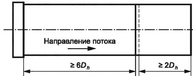
Рисунок М.1 — Схема выбора мерного сечения
