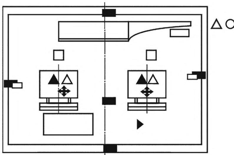
Рисунок Б.11 — Размещение точек измерения параметров микроклимата для холодного периода года в операторской СПС
