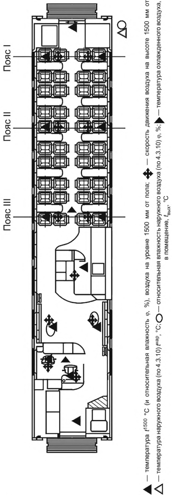
Рисунок Б.3 — Размещение точек измерения параметров микроклимата для теплого периода года в прицепном вагоне МВПС (вагон-ресторан)
