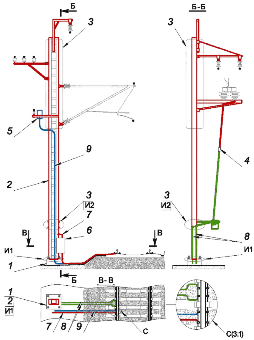
д) Металлическая консольная опора с разъединителем
