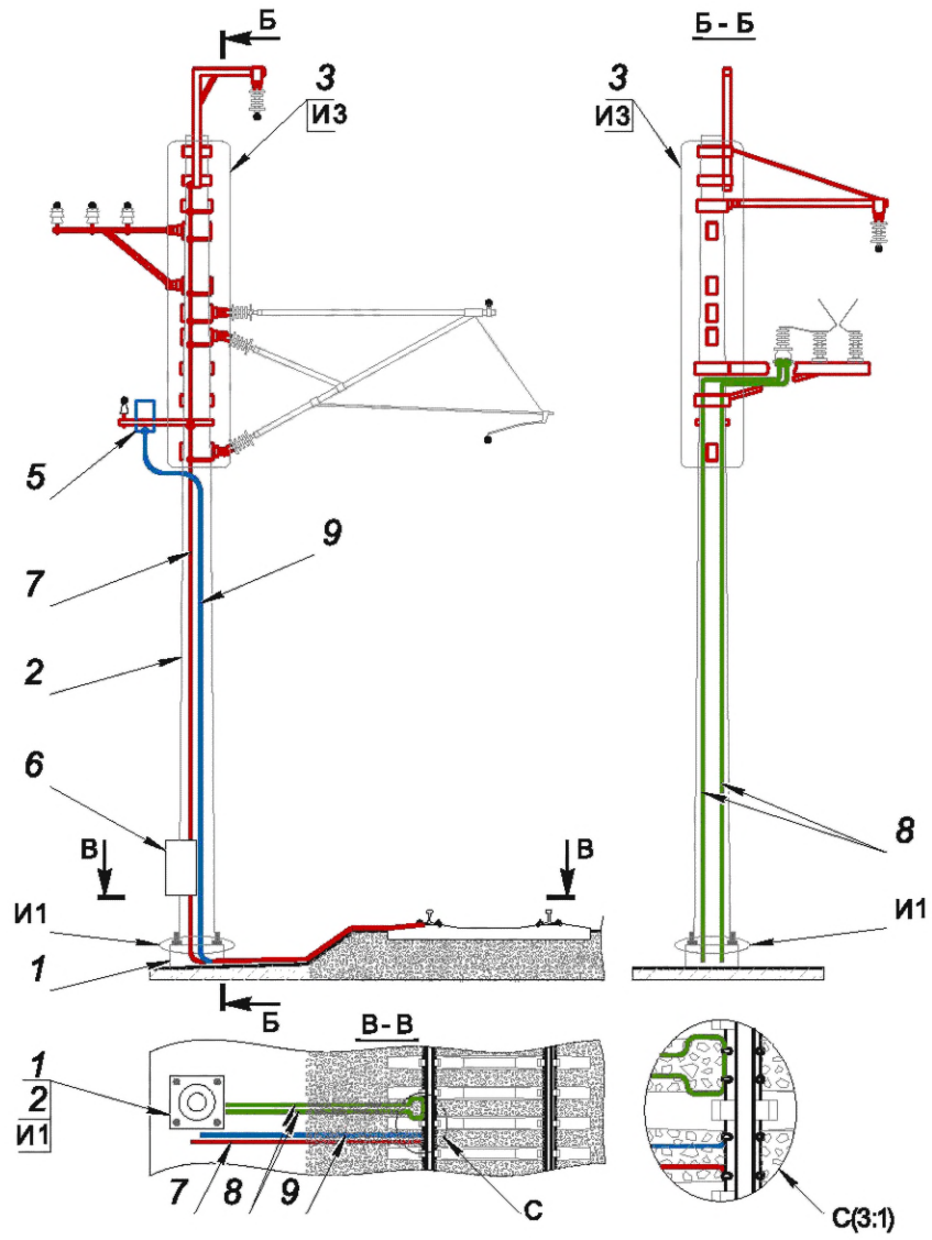
б) Железобетонная консольная опора с ограничителем перенапряжений
