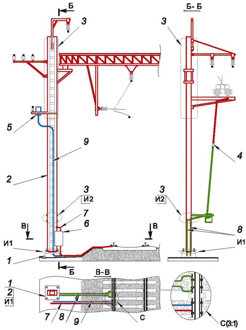
и) Металлическая опора жесткой поперечины
