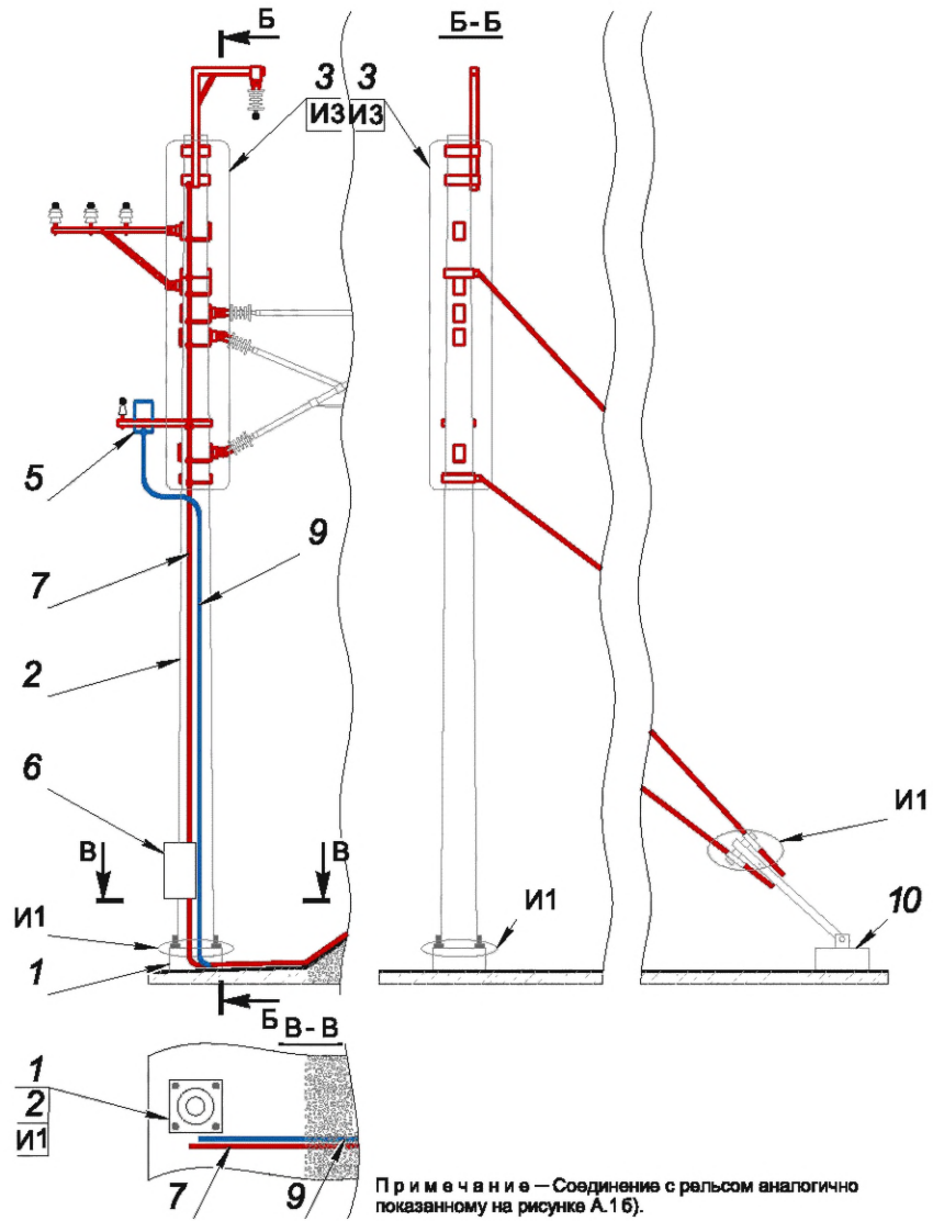
в) Железобетонная консольная опора с оттяжкой
