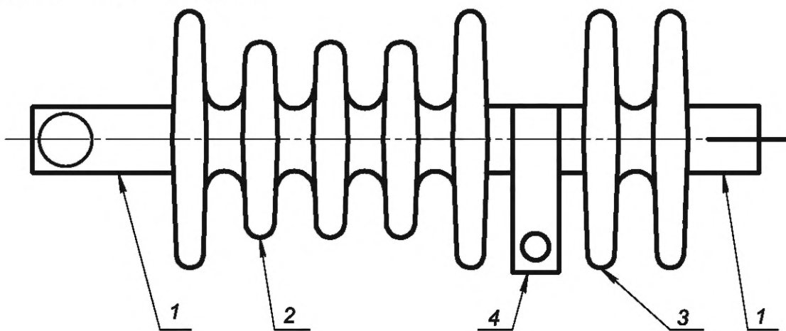
1 — арматура; 2 и 3 — изоляционные части; 4 — заземляемая вставка
