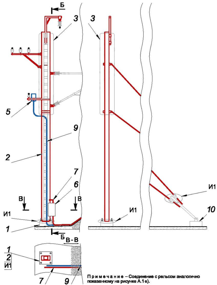
ж) Металлическая консольная опора с оттяжкой
