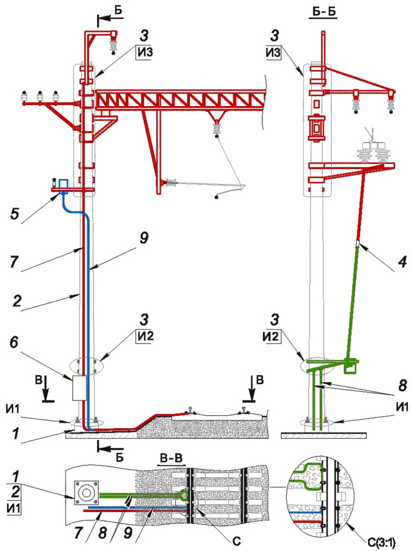
г) Железобетонная опора жесткой поперечины
