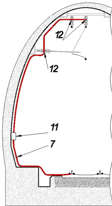
к) Контактная сеть в тоннеле
