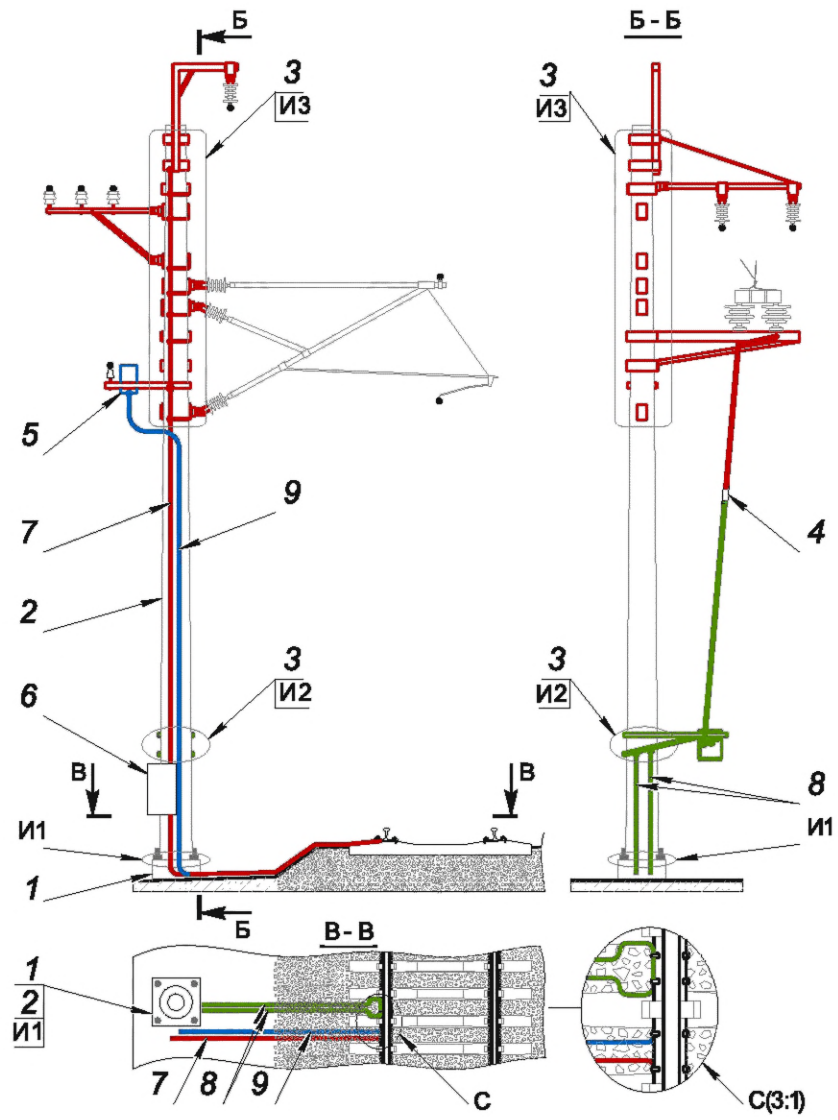
а) Железобетонная консольная опора с разъединителем
