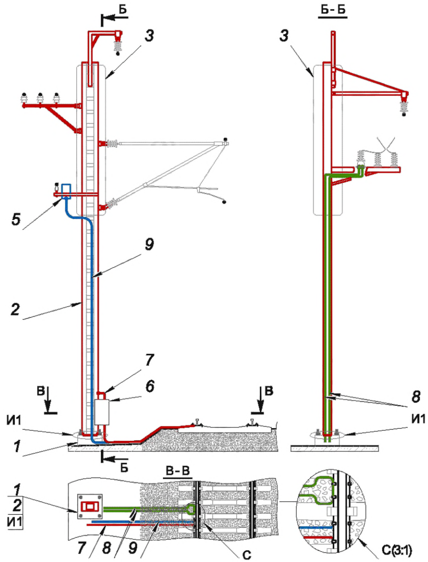
е) Металлическая консольная опора с ограничителем перенапряжений
