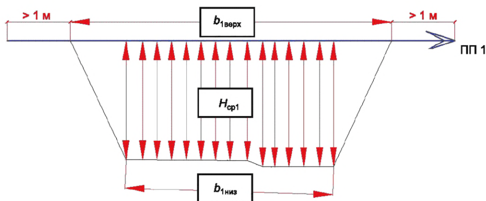
b_{1верх} — ширина выемки на поверхности по выбранному поперечному профилю; b_{1низ} — ширина выемки по дну для выбранного поперечного профиля; H_{ср1} — средняя толщина слоя обратной засыпки по выбранному поперечному профилю Рисунок В.2 — Схема выполнения поперечного георадарного профиля (вид в профиле)
