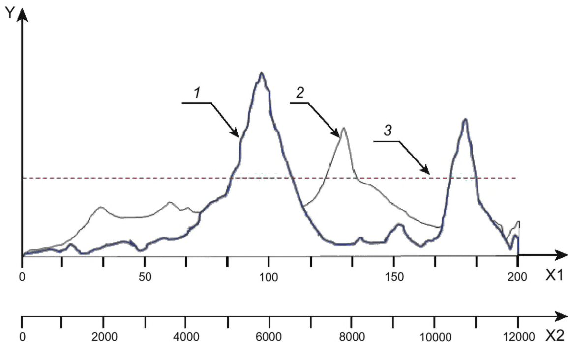
X1 — частота вращения шпинделя, Гц; X2 — частота вращения шпинделя, мин -1 ; Y — LTSC, мм/с; 1 — спектр вибрации с LTSC выше предельного значения; 2 — спектр вибрации с LTSC ниже предельного значения (после исключения области резонанса); 3 — предельное значение LTSC
