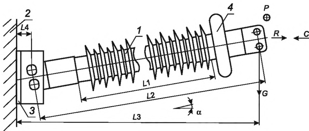
1 — изолятор консольный; 2 — стойка опоры; 3 — узел крепления консольного изолятора к стойке опоры; 4 — защитная арматура (необходимость установки определяют конструкцией); G, C, R, P — векторы механических сил, воздействующих на траверсу
