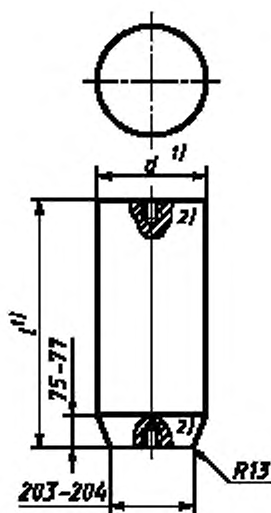
Рисунок 1 — Стандартный предмет для испытаний на удар
