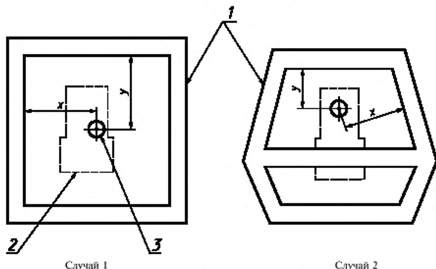
1 — главный верхний горизонтальный элемент; 2 — вертикальная проекция зоны ограничения деформации; 3 — конус стандартного предмета
