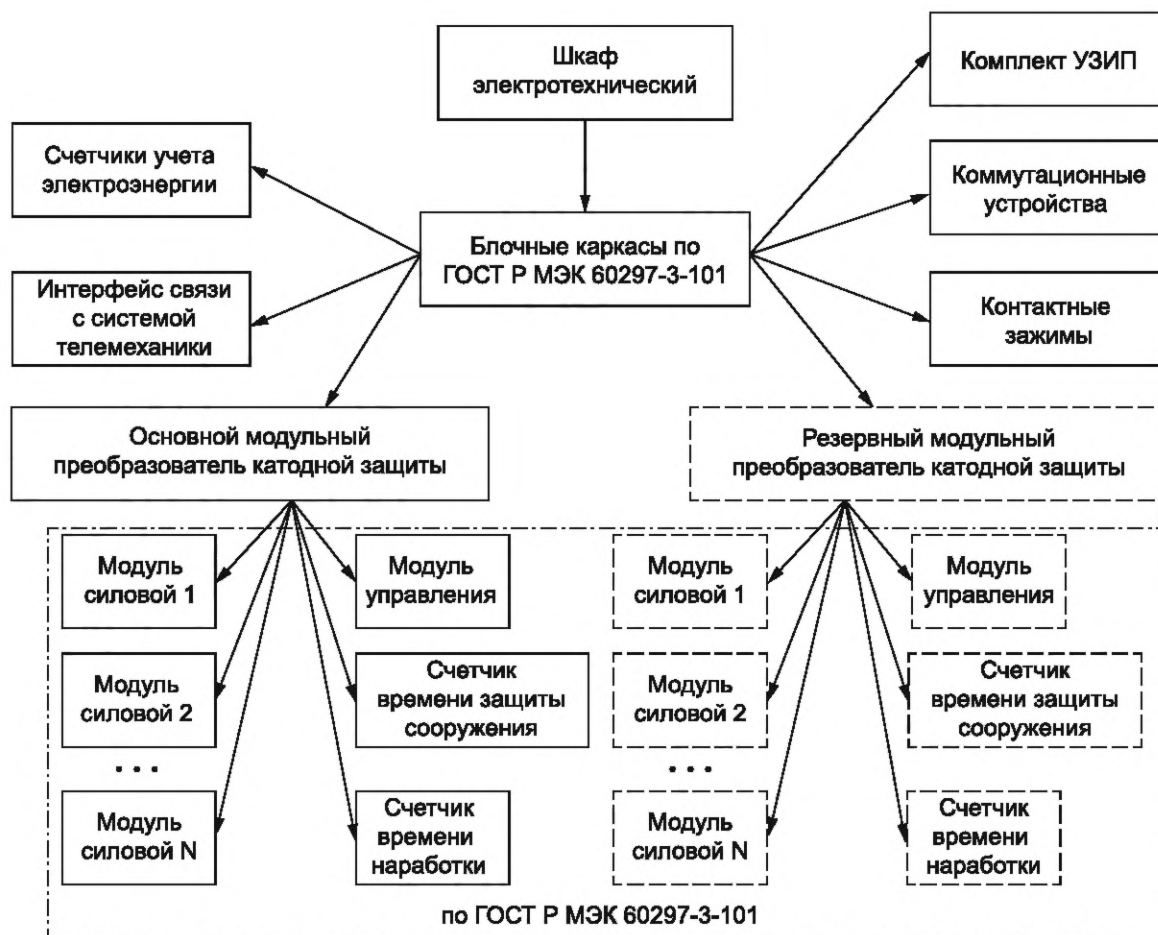
Рисунок 3 — Функциональный состав МСКЗ
