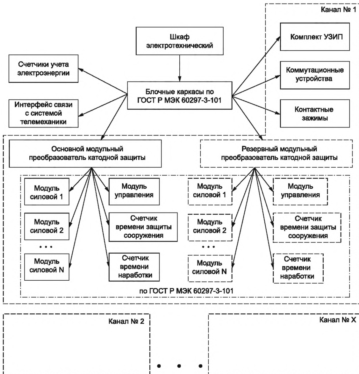
Рисунок 4 — Функциональный состав МСКЗ(Х)
