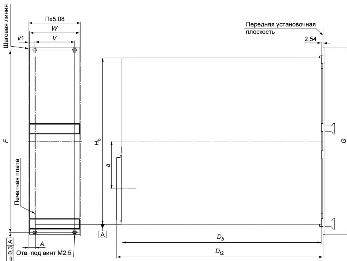
Рисунок В.1 — Основные размеры силовых модулей
