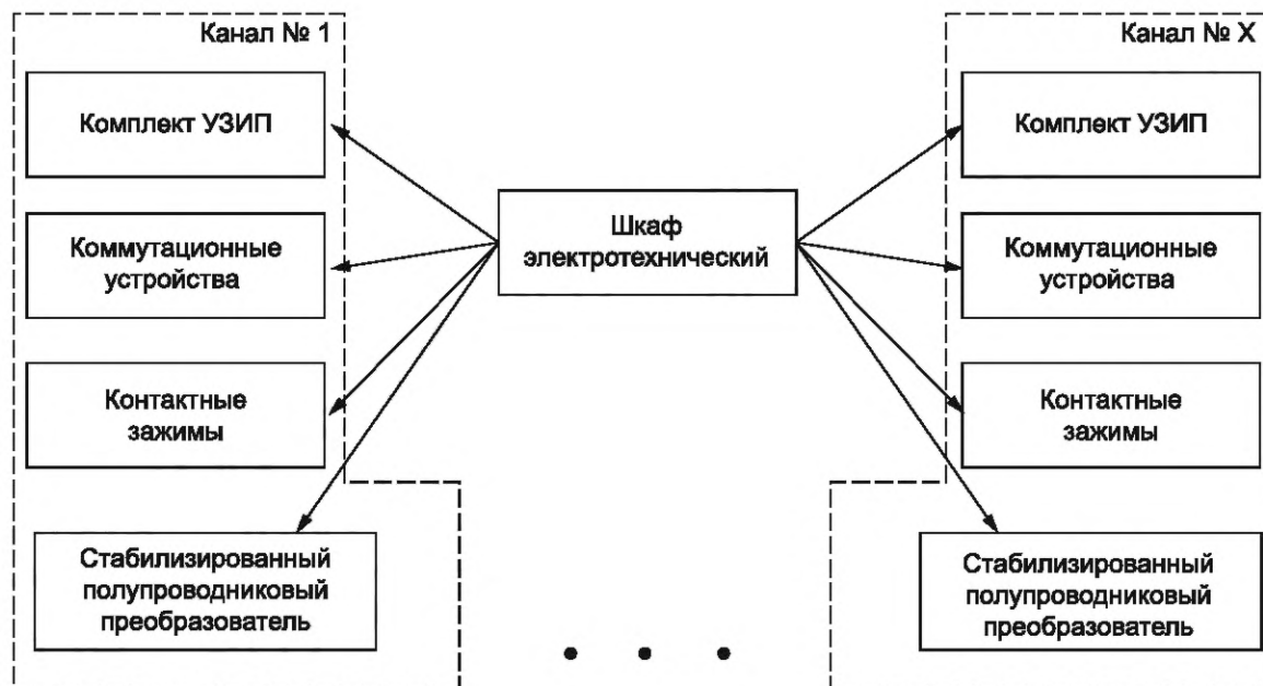
Рисунок 2 — Функциональный состав АСКЗ(Х)
