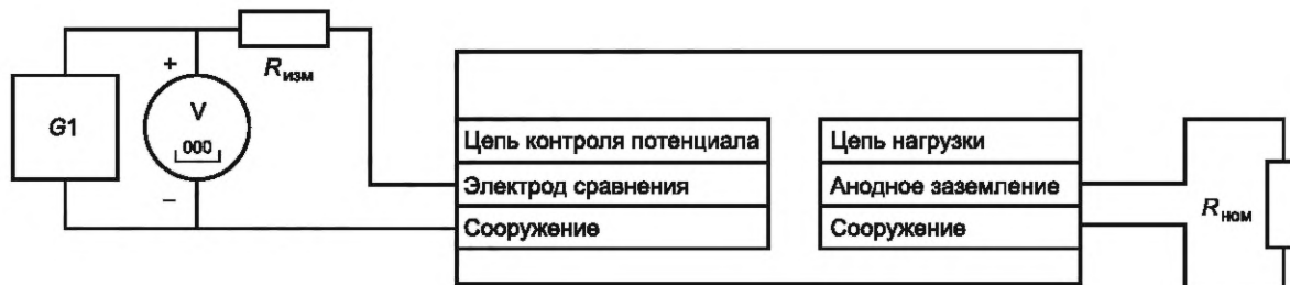
Рисунок 6 — Схема проверки входного сопротивления цепи контроля потенциала
