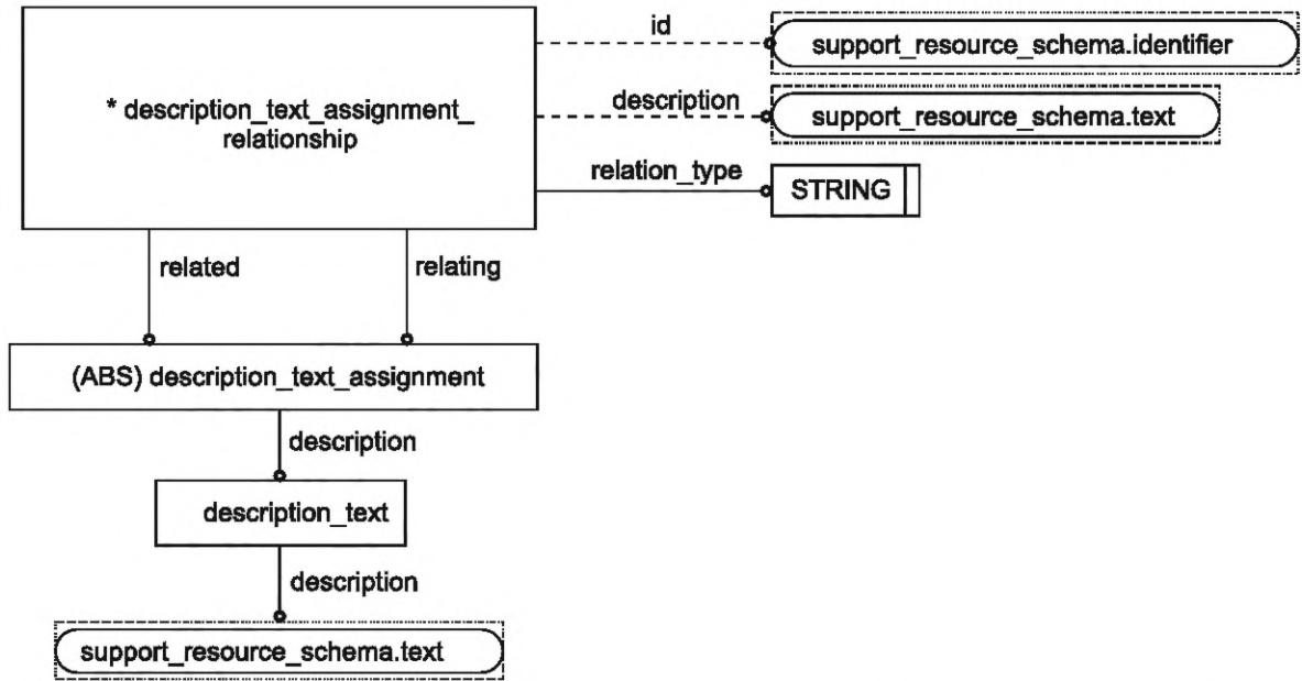
Рисунок D.6 — Представление схемы systems_engineering_representation_schema на уровне объектов в формате EXPRESS-G (6 из 8)
