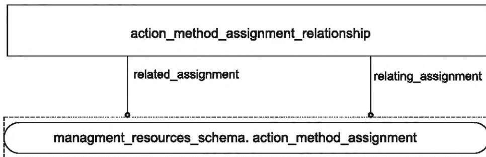
Рисунок D.8 — Представление схемы systems_engineering_representation_schema на уровне объектов в формате EXPRESS-G (8 из 8)
