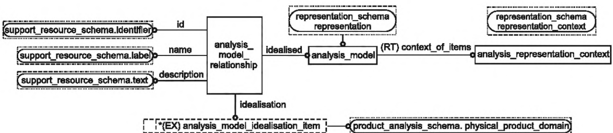
Рисунок D.5 — Представление схемы systems_engineering_representation_schema на уровне объектов в формате EXPRESS-G (5 из 8)
