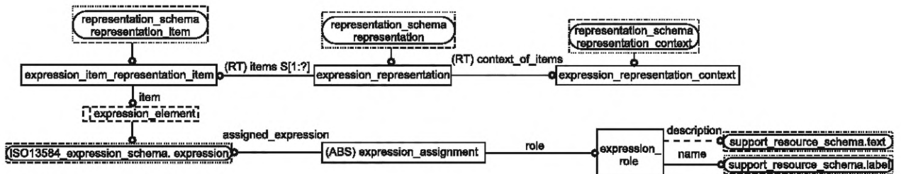
Рисунок D.7 — Представление схемы systems_engineering_representation_schema на уровне объектов в формате EXPRESS-G (7 из 8)
