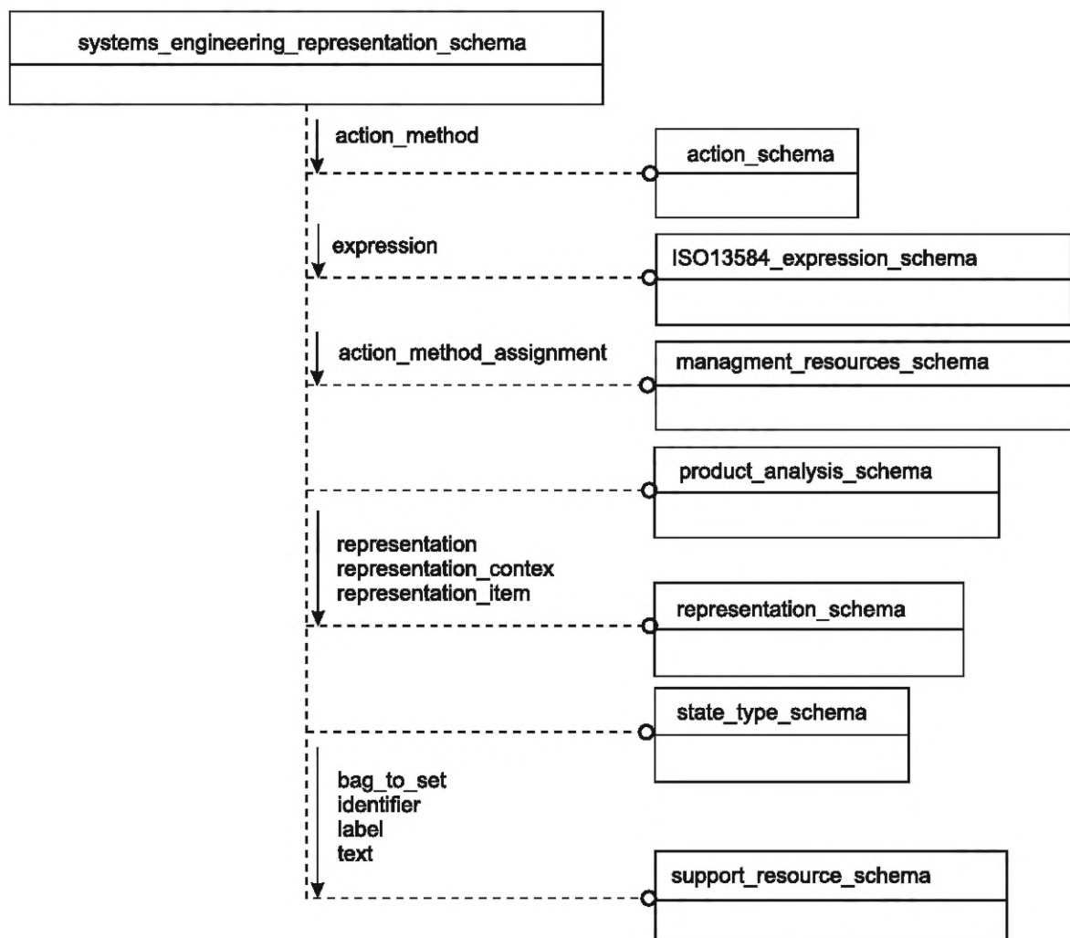
Рисунок D.1 — Представление схемы systems_engineering_representation_schema на уровне объектов в формате EXPRESS-G (1 из 8)
