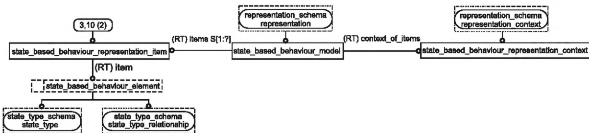
Рисунок D.3 — Представление схемы systems_engineering_representation_schema на уровне объектов в формате EXPRESS-G (3 из 8)
