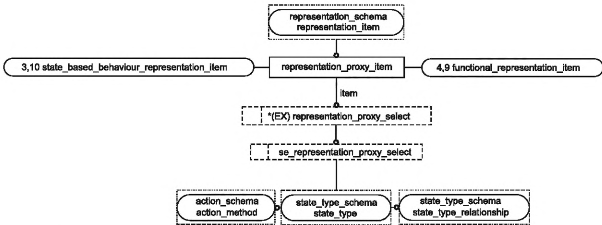
Рисунок D.2 — Представление схемы systems_engineering_representation_schema на уровне объектов в формате EXPRESS-G (2 из 8)
