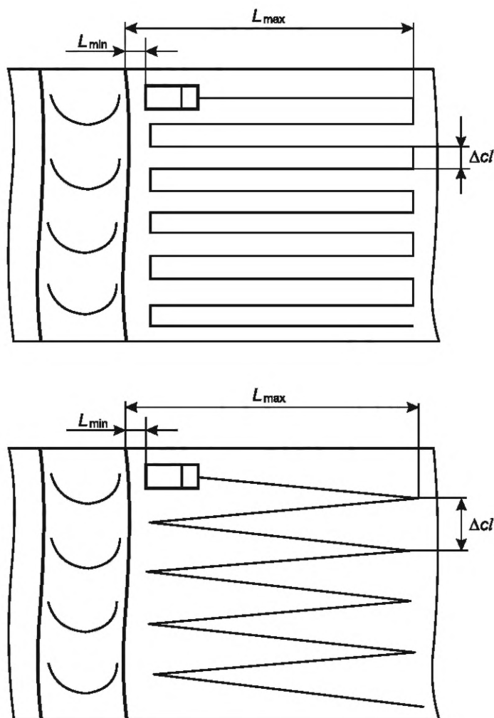
а) Варианты способа поперечно-продольного сканирования
