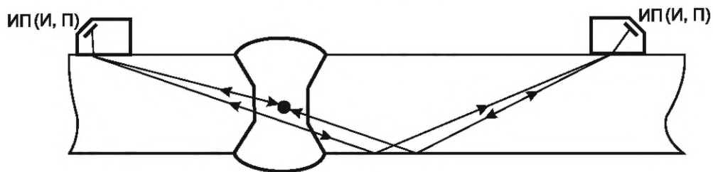
в) Эхо-теневой
