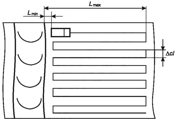
б) Способ продольно-поперечного сканирования
