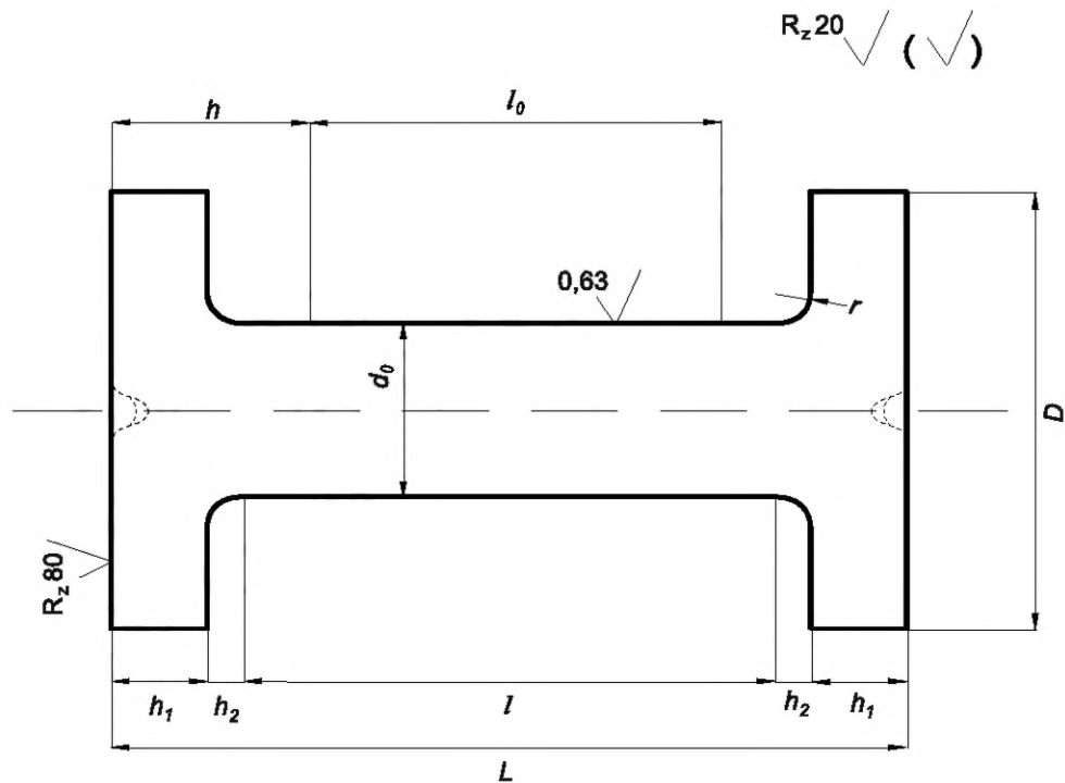
Рисунок П.1 — Образец для определения механических характеристик гидротурбинных сталей
