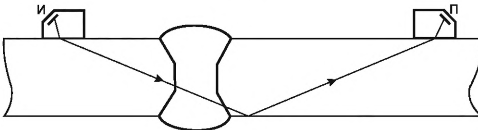
б) Зеркально-теневой
