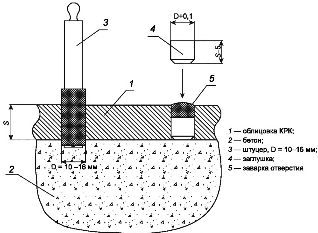
Рисунок Н.2 — Оборудование и ликвидация отверстий в облицовке КРК
