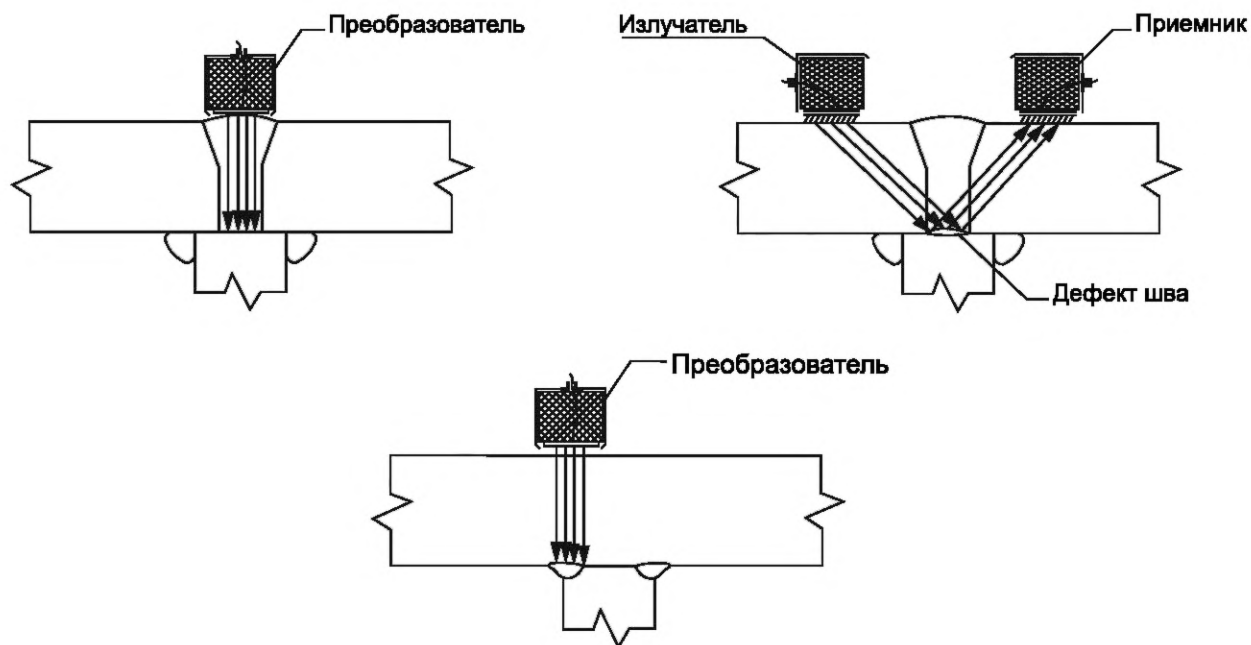
Рисунок К.3 — Схема контроля сварных стыковых соединений на ребре жесткости (контроль эхо-методом)
