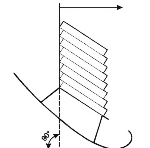
а) Метод для кресла-качалки: исходное положение
