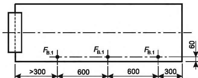
а) Шезлонг без подлокотника
