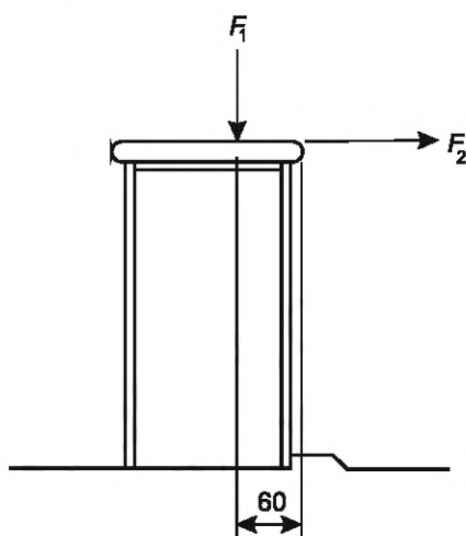
в) Мебель для сидения без спинки
