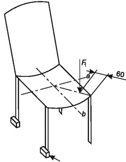
б) Все остальные виды мебели для сидения
