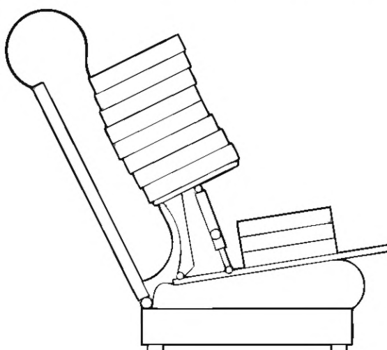
b) Практический пример метода испытания: кресла с откидывающейся спинкой без подставки для ног
