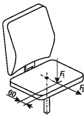
а) Поворотное изделие (кресло)
