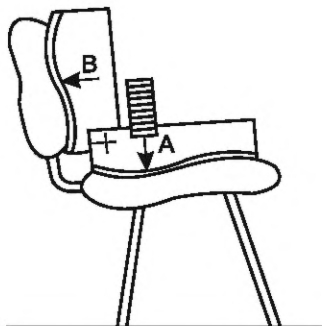
а) Мягкая/гибкая мебель для сидения со спинкой
