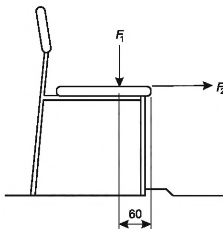
б) Мебель для сидения со спинкой
