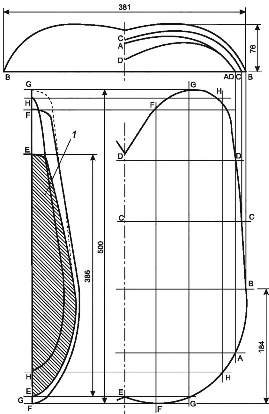
Рисунок А.2 — Конструкция нагрузочной площадки сиденья — литая конструкция
