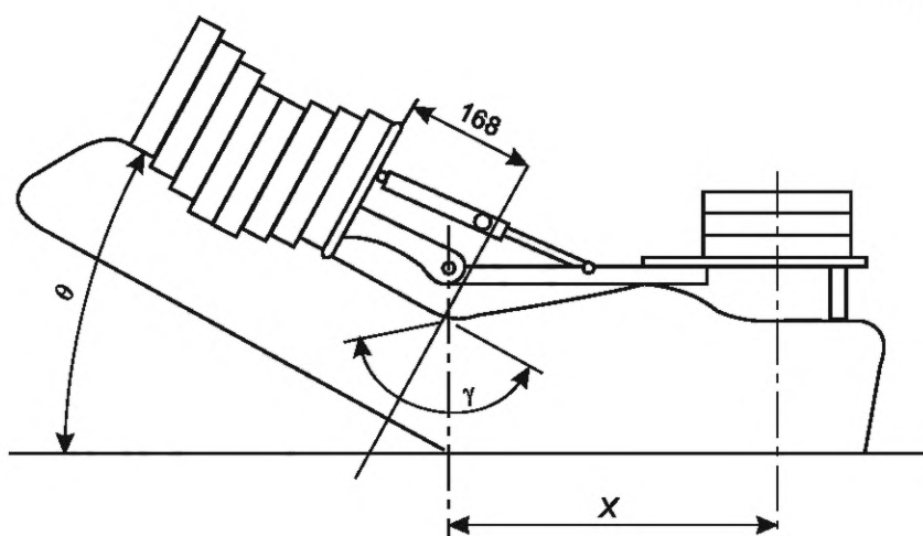
а) Испытание кресла с откидывающейся спинкой без подставки для ног
