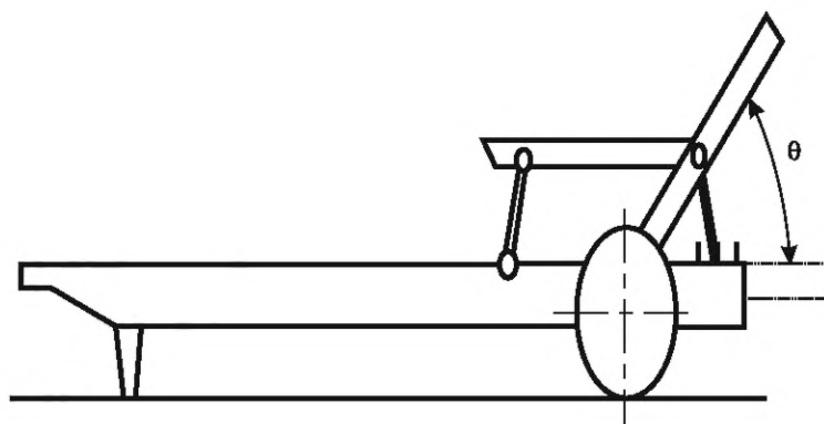
Рисунок 1 — Образец шезлонга
