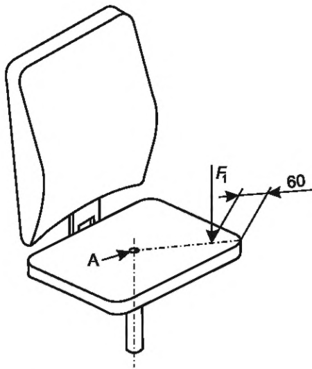
а) Поворотное изделие (кресло)
