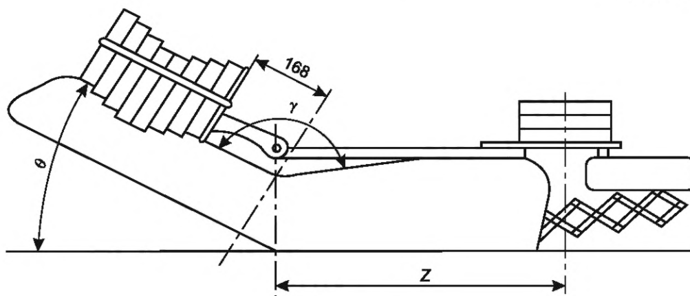
а) Испытание кресла с откидывающейся спинкой с подставкой для ног
