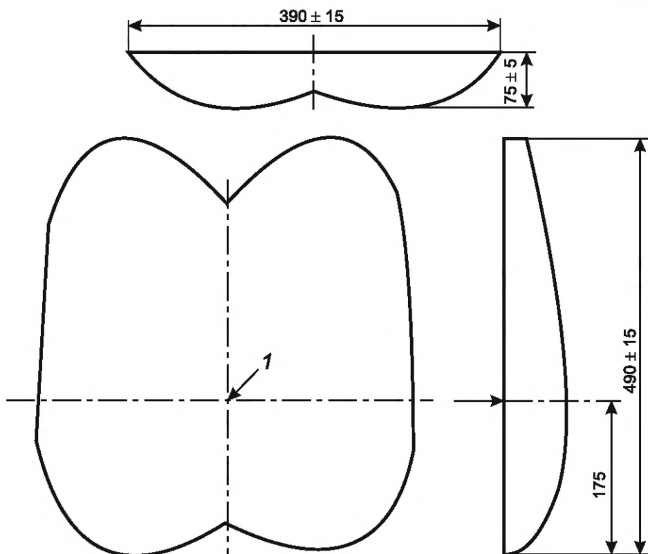
Рисунок 9 — Размеры нагрузочного штампа для сиденья
