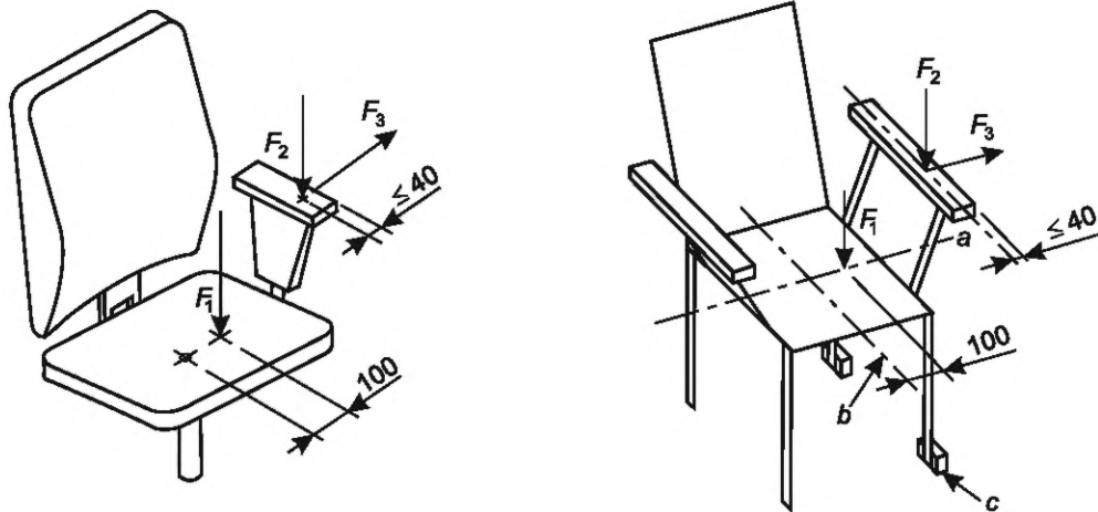
а) Поворотное изделие (кресло)
