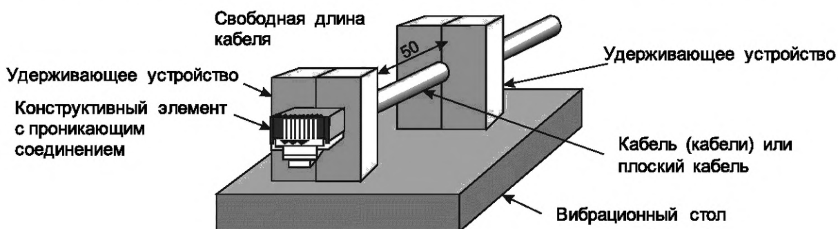
Рисунок 6 — Схема проведения испытаний, вибрация
