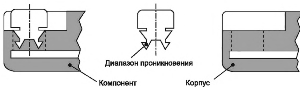
Рисунок А.1 — Пример заделки ПИ как составляющая часть соединителя
