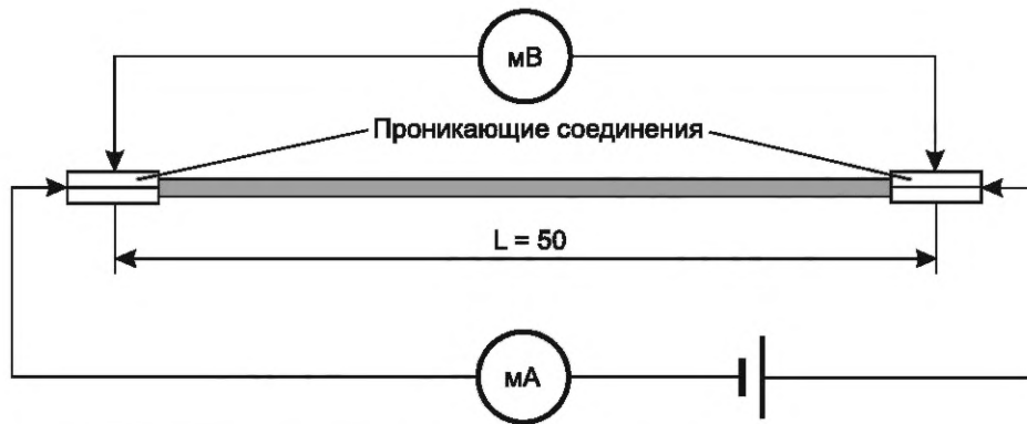
Рисунок 7 — Испытательная схема, контактное сопротивление (метод измерения для мишурного провода, плоских токопроводящих жил, плоского гибкого шлейфа)
