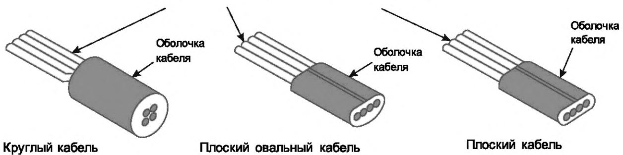
Рисунок А.4 — Примеры круглого, плоского и плоского овального кабеля в оболочке
