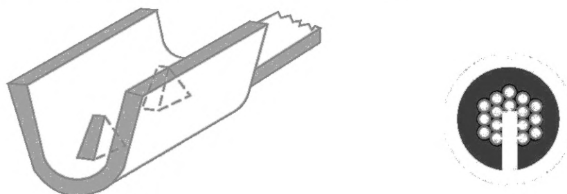
Рисунок А.3 — Пример заделки при помощи прокалывания изоляции многопроволочных токопроводящих жил
