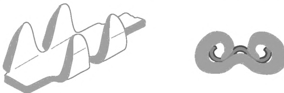
Рисунок А.2 — Пример заделки ПИ для плоской токопроводящей жилы
