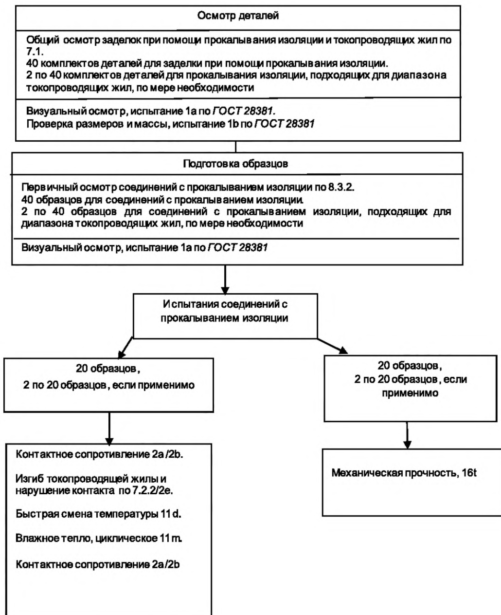
Рисунок 10 — Расширенная программа испытаний (см. 8.3)
