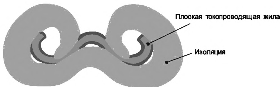
Рисунок 2 — Пример соединения с ПИ с изолированной плоской токопроводящей жилой
