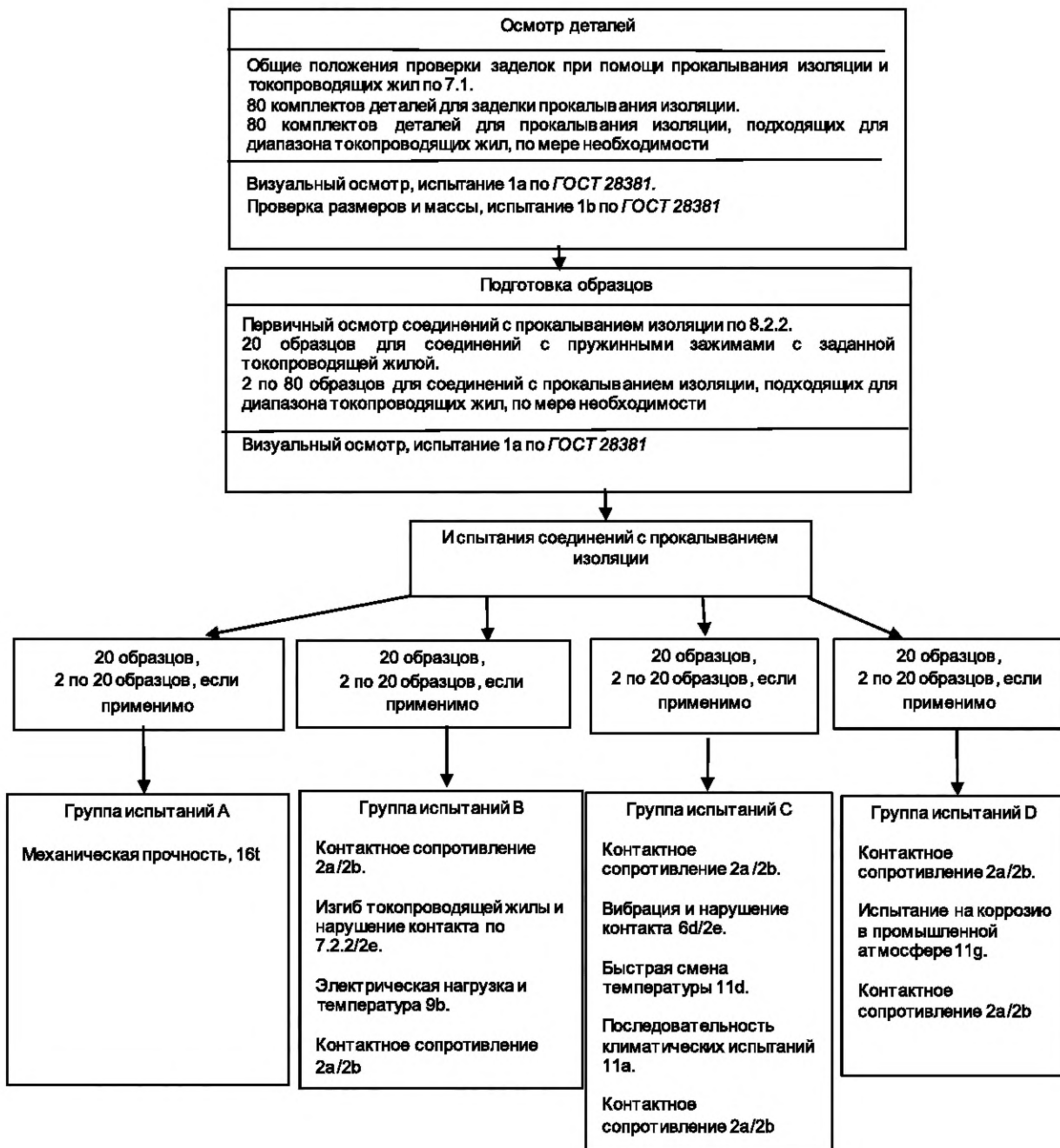
Рисунок 9 — Базовая программа испытаний (см. 8.2)
