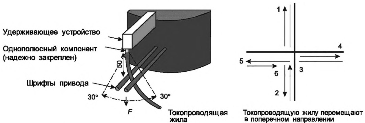
Рисунок 4 — Схема испытания на изгиб отдельной токопроводящей жилы
