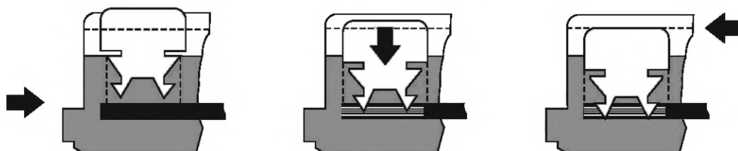
Рисунок 1 — Пример корпусного соединения с прокалыванием изоляции (показано одно соединение)
