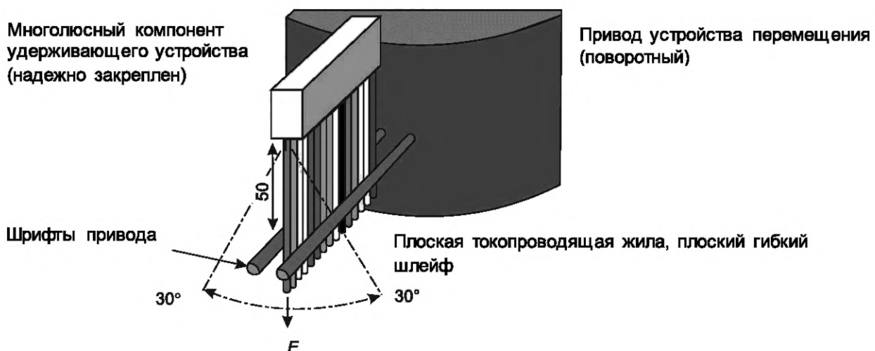
Рисунок 5 — Схема испытания на изгиб плоской токопроводящей жилы, плоского гибкого шлейфа
