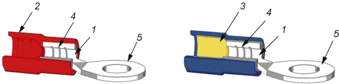
а) Исполнение с ПВХ-изоляцией
