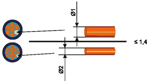
Рисунок 14 — Соотношение диаметров при обжиме токопроводящих жил с разными диаметрами отдельных жил
