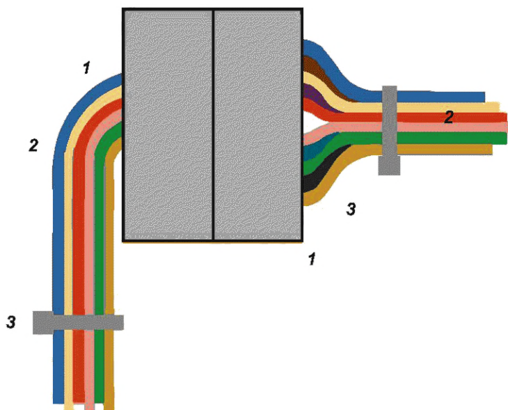
1 — соединитель; 2 — изолированный провод; 3 — хомут
