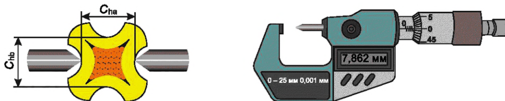
C_{ha} — высота обжима 1; C_{hb} — высота обжима 2
