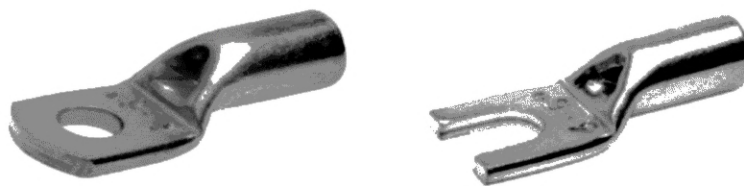
Рисунок 22 — Кабельные наконечники, изготовленные из труб, для жил класса 5
