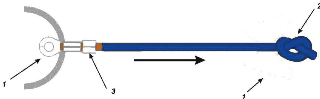
1 — точки крепления; 2 — узел; 3 — зажим для изоляции не зажимает изоляцию токопроводящей жилы
