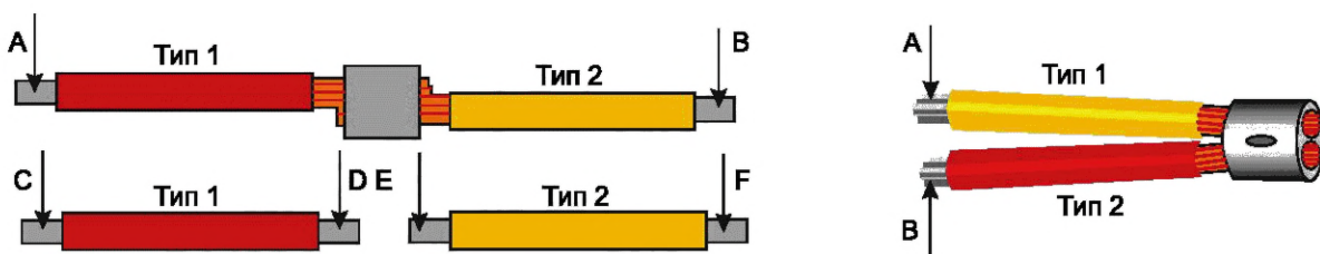
Рисунок 43 — Схема измерения сопротивления обжимного соединения, предназначенного для сращиваний или соединений с многопроволочной токопроводящей жилой
