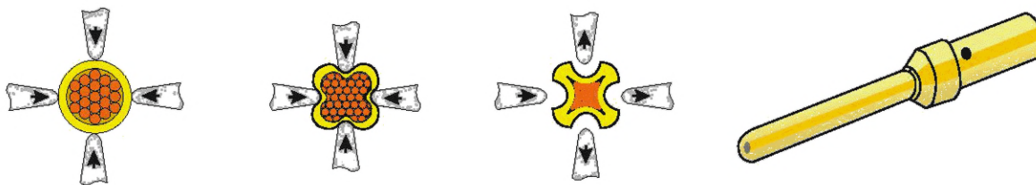
Рисунок 24 — Процесс четырехточечного обжима с помощью регулировки устройства
