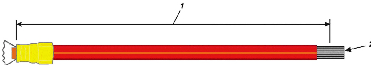
1 — минимальная длина — 200 мм; 2 — свободный конец провода зачищен и залужен погружением, обжат, припаян или сварен ультразвуком
