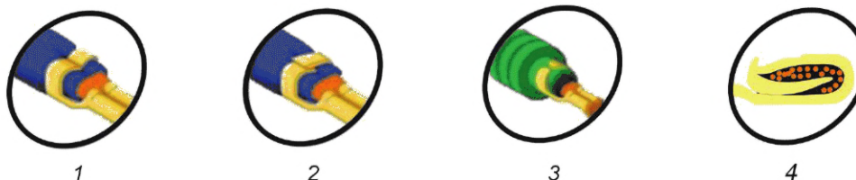
1 — В-образный обжим; 2 — обжим внахлест; 3 — О-образный обжим; 4 — угловой обжим
