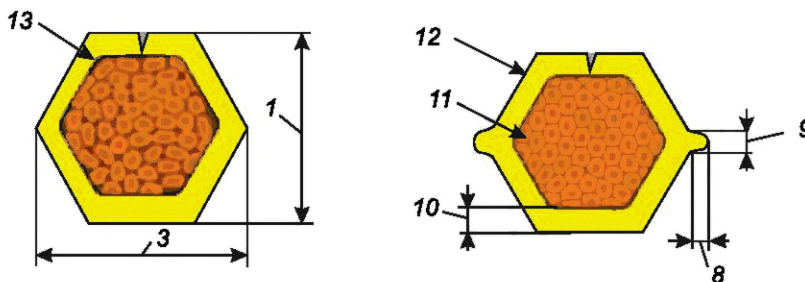
Рисунок А.24 — Размеры микросекционного размера для четырехточечного обжима хвостовика закрытого типа
