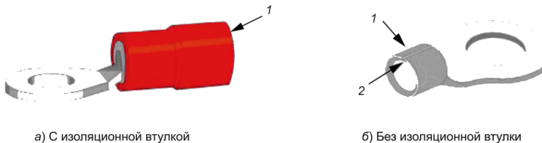
Рисунок А.2 — Хвостовики закрытого типа
