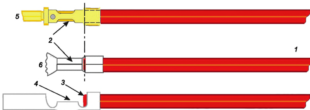
1 — многопроволочная токопроводящая жила; 2 — область зажима токопроводящей жилы; 3 — конец токопроводящей жилы; 4 — проволоки не видны; 5 — обработанный контакт; 6 — контакт В-обжима
