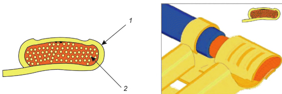
Рисунок А.3 — Форма обжимного соединения по оси токопроводящей жилы
