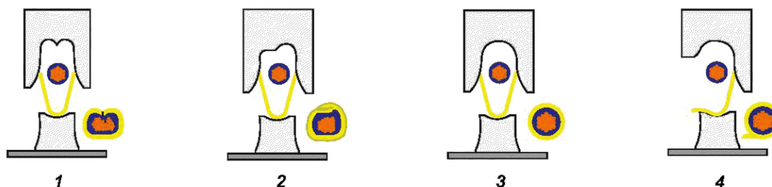
1 — В-образный обжим; 2 — обжим внахлест; 3 — О-образный обжим; 4 — угловой обжим
