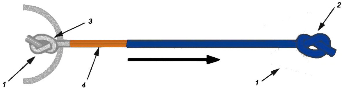
Рисунок А.16 — Определение внутренней прочности токопроводящей жилы на растяжение (50 мм/мин)
