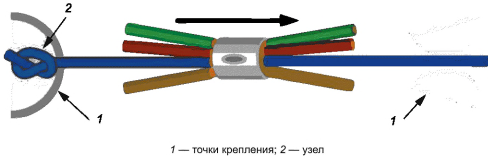
Рисунок А.18 — Испытание на растягивающее усилие сращиваний (50 мм/мин)
