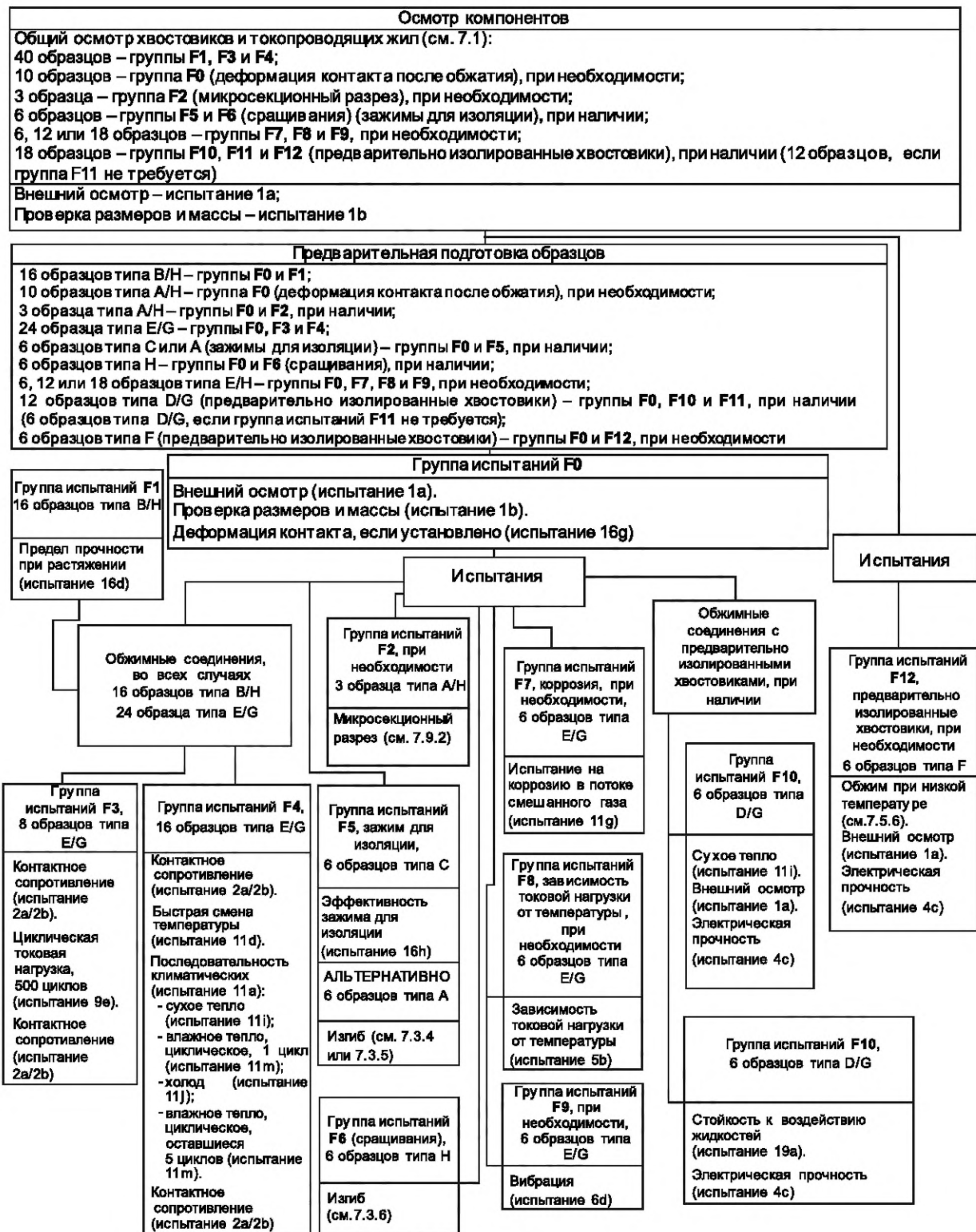
Рисунок 58 — Расширенная программа испытаний (см. 8.3)
