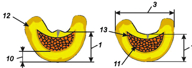
Рисунок А.22 — Размеры микросекционного разреза для В-обжима
