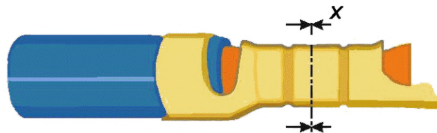
X — центр зоны обжима
