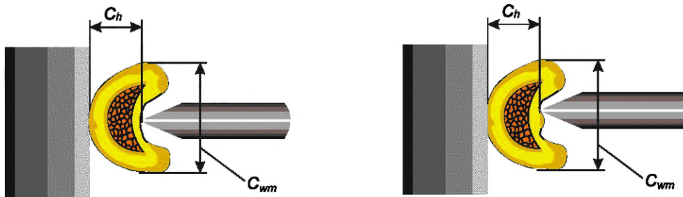
C_h — высота обжима; C_{wm} — измеряемая ширина обжима
