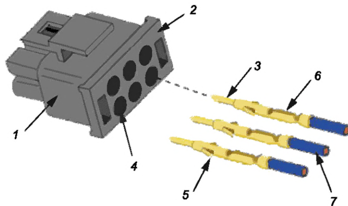
1 — соединительная вставка; 2 — задняя стенка; 3 — контакт; 4 — контактная полость; 5 — удерживающая пружина; 6 — обжатое соединение; 7 — изолированные токопроводящие жилы
