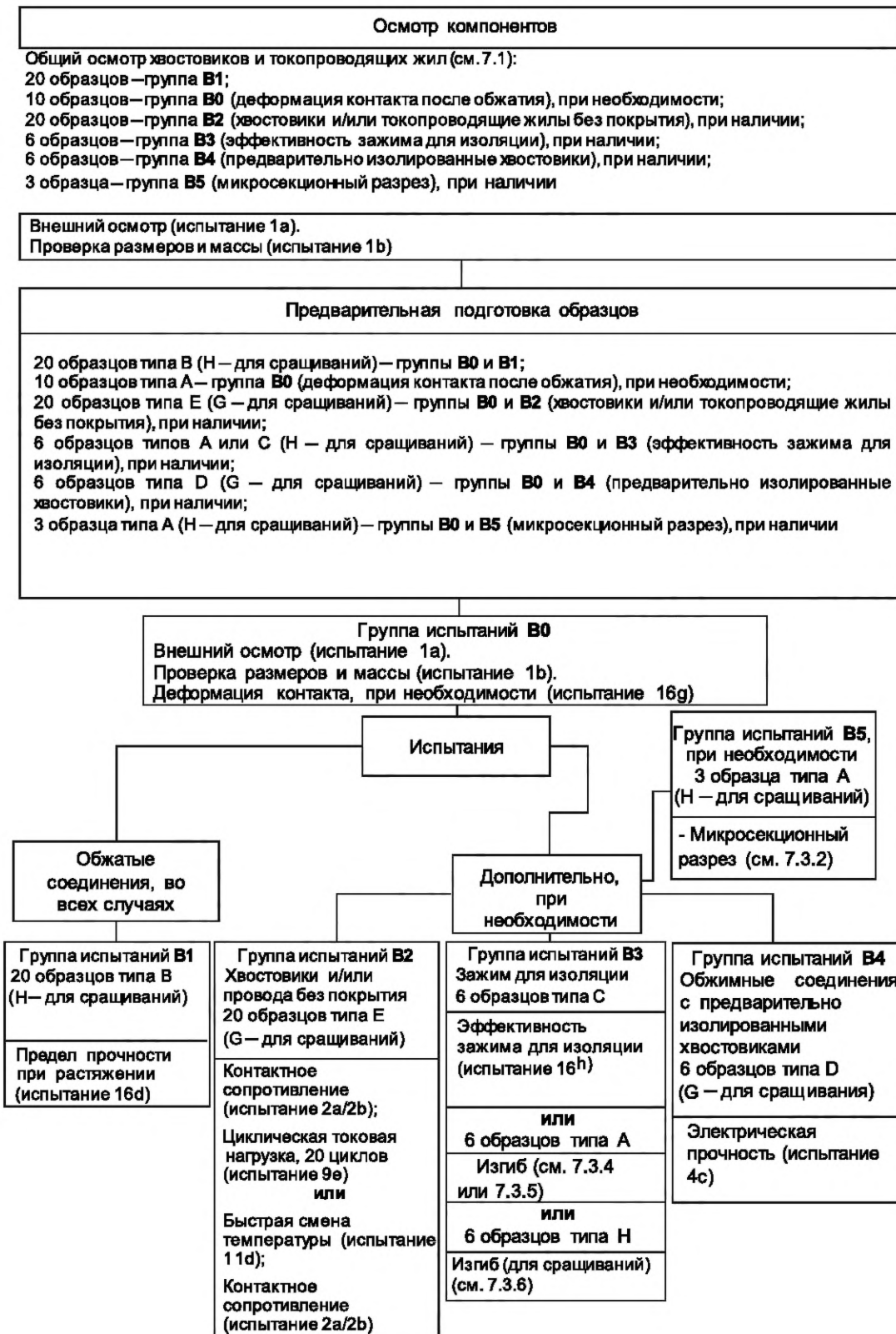
Рисунок 57 — Базовая программа испытаний (см. 8.2)
