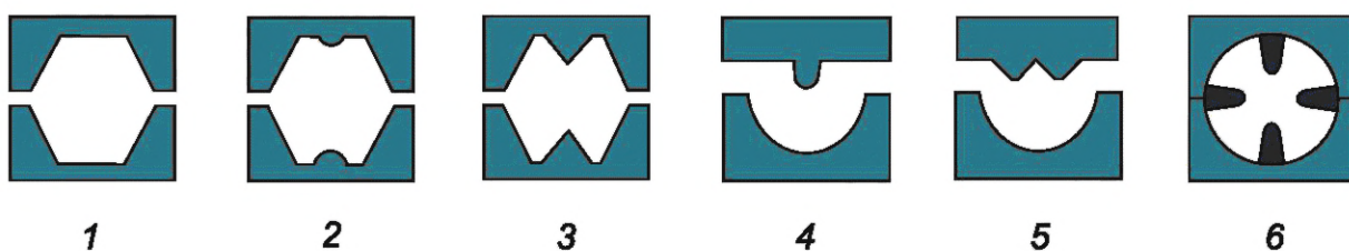
1 — гексагональная; 2 — гексагональная с вдавливанием; 3 — WM; 4 — трапециевидная; 5 — двухконтурная; 6 — четырехточечная
