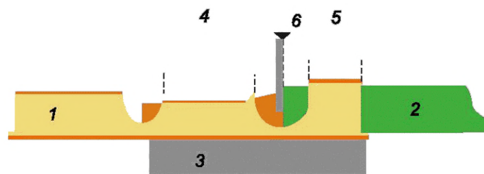
Рисунок 6 — Пример расположения позиционера для хвостовика
