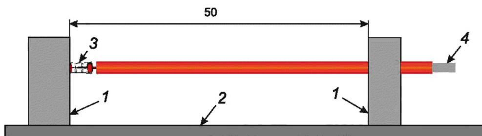
Рисунок 41 — Установка для вибрационного испытания
