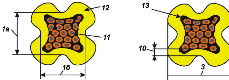
Рисунок А.23 — Размеры микросекционного разреза для гильз закрытого типа и кабельных наконечников
