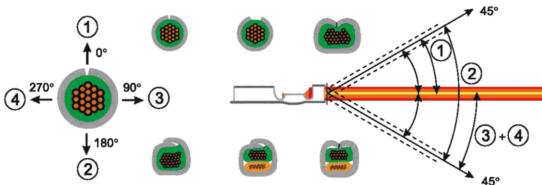
Рисунок 38 — Испытание на изгиб для наконечников с неизолированным хвостовиком
