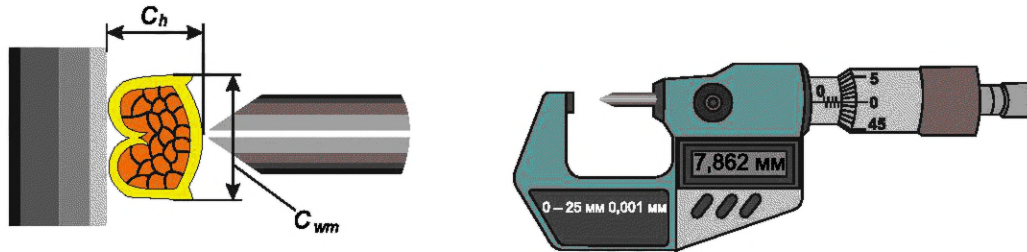
C_h — высота обжима; C_{wm} — измеряемая ширина обжима
