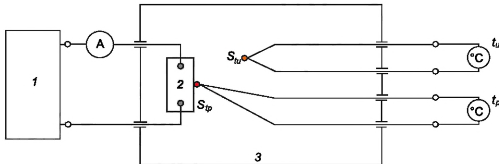
Рисунок 45 — Испытательная установка для измерения превышения температуры под нагрузкой
