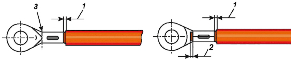
1 — расстояние до изоляции; 2 — выступ жил; 3 — торец хвостовика
