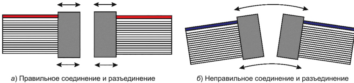
Рисунок А.40 — Соединение и разъединение многополюсных разъемов
