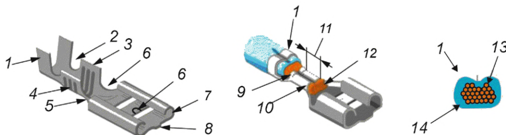
1 — лапки зажима для изоляции; 2 — окно для проверки изоляции; 3 — лапки зажима для токопроводящей жилы; 4 — канавки штамповки; 5 — переходный элемент; 6 — блокировка контакта; 7 — площадь контакта; 8 — упор; 9 — входная воронка; 10 — выходная воронка; 11 — зона обжатия; 12 — выступ жил; 13 — проволоки жил; 14 — изоляция токопроводящей жилы
