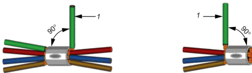
Рисунок 40 — Испытание на изгиб сращиваний
