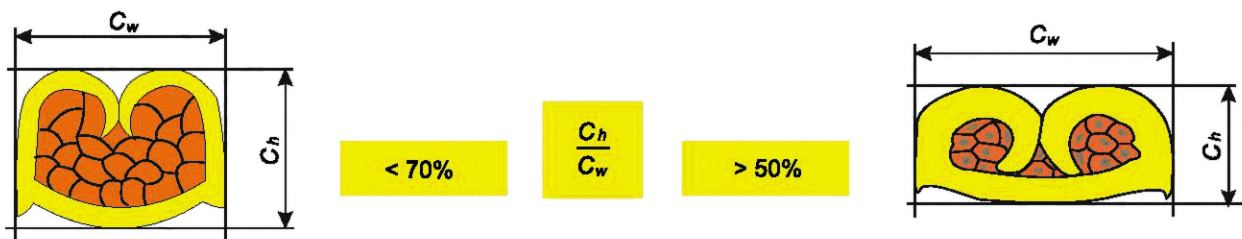
Рисунок А.28 — Отношение высоты обжима к ширине обжима
