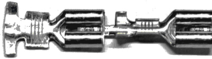
Рисунок А.20 — Пример разъемов с хвостовиком открытого типа для продольной подачи
