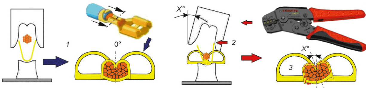
а) Прямолинейное параллельное обжатие
