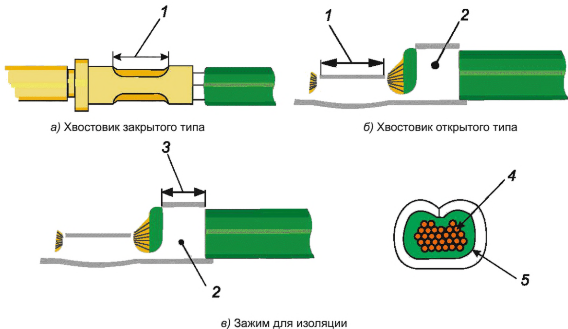
Рисунок 11 — Зоны обжатия
