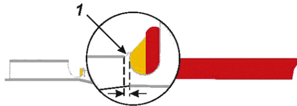
1 — обжимная воронка
