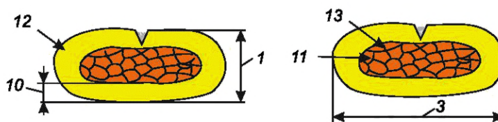
1 — высота обжима C_h ; 3 — измеряемая ширина обжима C_{wm} ; 10 — толщина дна S_b ; 11 — внутренняя поверхность A_{ci} ; 12 — внешняя поверхность A_{ca} ; 13 — пористость A_{pr}
