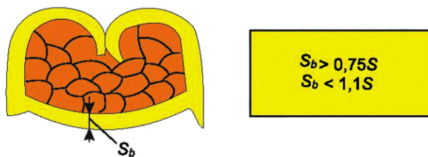
Рисунок А.32 — Расстояние от кромки обжима до дна
