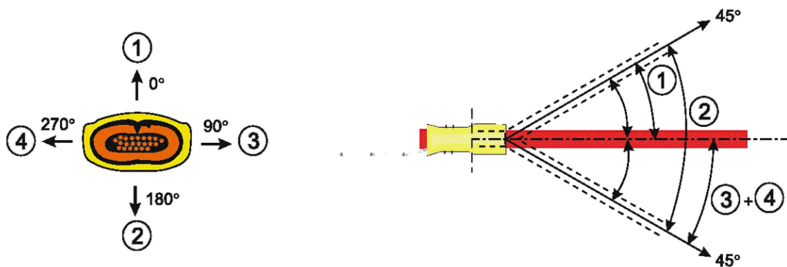
Рисунок 39 — Испытание на изгиб для соединений при помощи обжима с предварительно изолированными наконечниками
