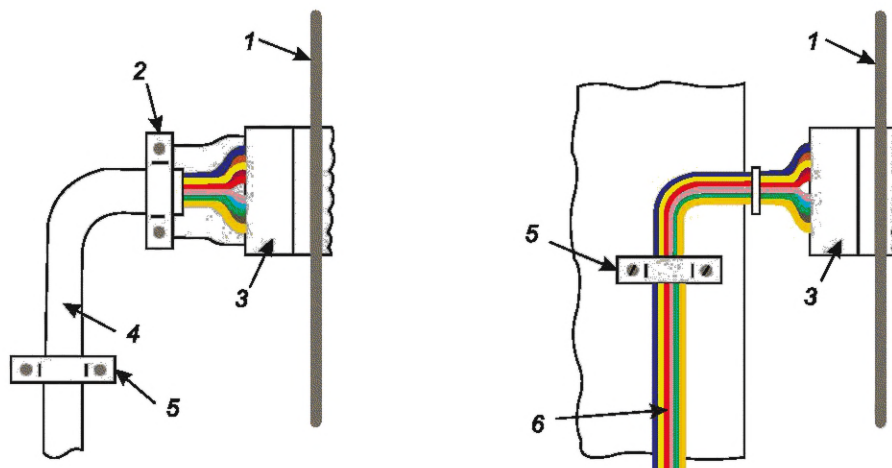
1 — корпус; 2 — кабельный зажим; 3 — соединитель; 4 — кабель; 5 — монтажный зажим; 6 — жгут проводов
