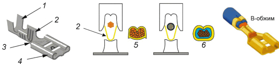
1 — лапки зажима для изоляции; 2 — лапки зажима для токопроводящей жилы; 3 — переходный элемент; 4 — площадь контакта; 5 — обжатие токопроводящей жилы; 6 — зажим для изоляции
