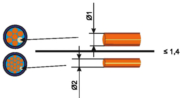
Рисунок 29 — Соотношение диаметров при обжиме токопроводящих жил с разными диаметрами отдельных жил в сращивании
