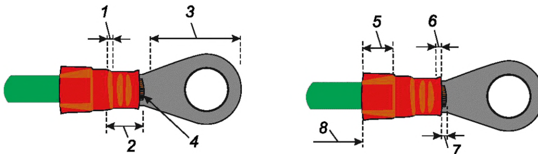
1 — входная воронка зажима провода (не видна); 2 — зона обжима; 3 — площадь контакта; 4 — выступ жил; 5 — изоляция наконечника; 6 — выходная зона обжима (не видна); 7 — выступ жил; 8 — изолированная токопроводящая жила
