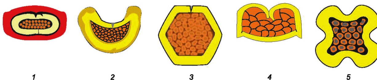
1 — предварительно изолированный обжим; 2 — трапециевидный обжим; 3 — гексагональный обжим; 4 — V-обжим; 5 — четырехточечный обжим
