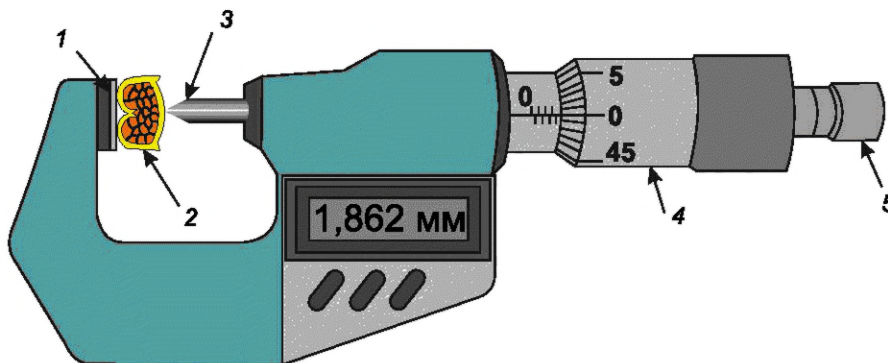
1 — неподвижная пятка; 2 — соединение; 3 — подвижная пятка; 4 — микрометр; 5 — трещотка
