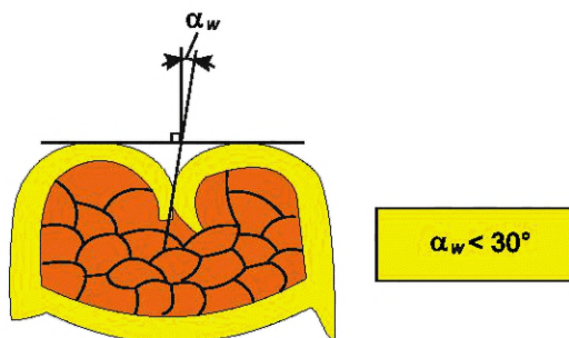
Рисунок А.30 — Угол опоры лапок обжима
