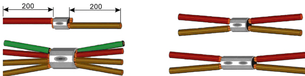
Рисунок 56 — Пример образца типа H (сращивание)
