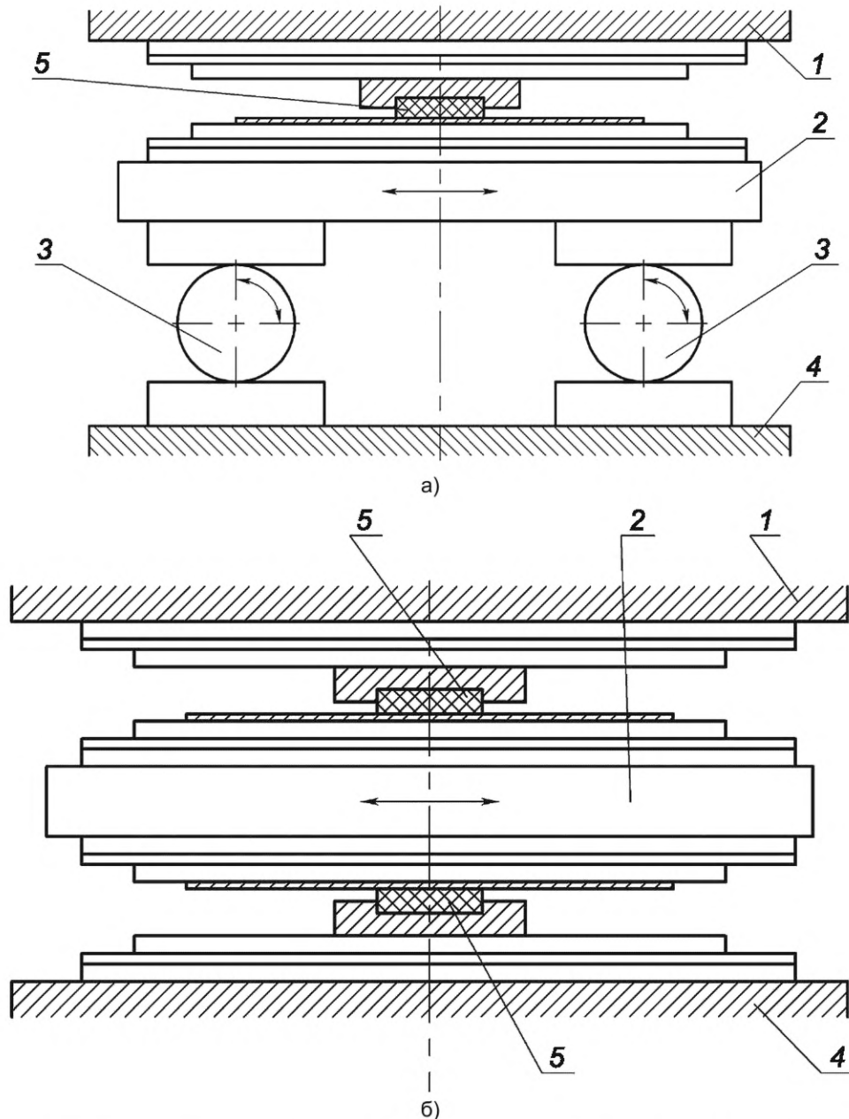
Рисунок Б.1 — Принципиальная схема испытательного стэнда
