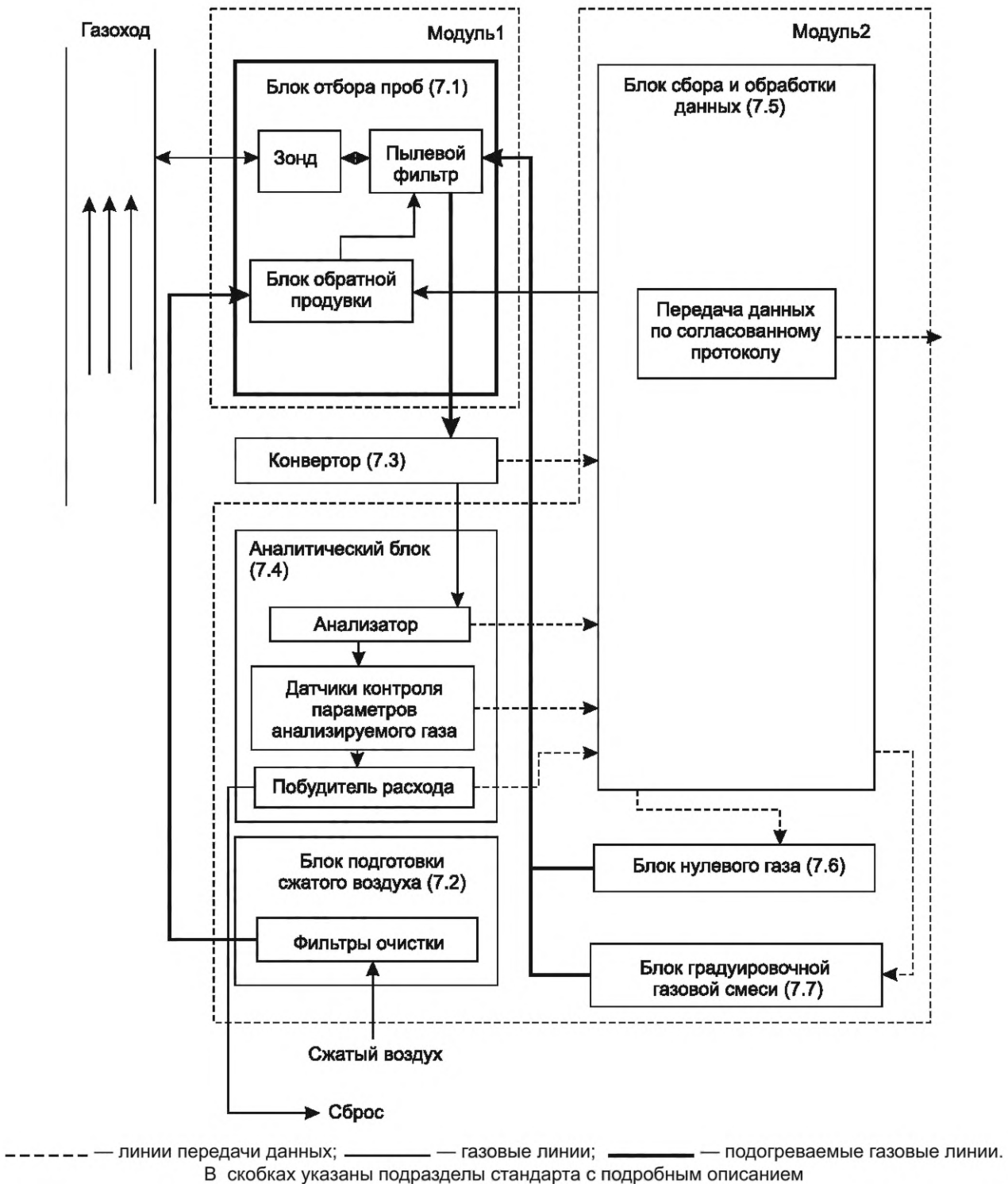
Рисунок 1 — Блок-схема системы при отборе проб без разбавления дымового газа
