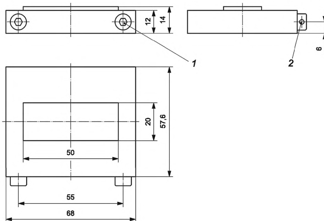
Рисунок В.1 — Плита
