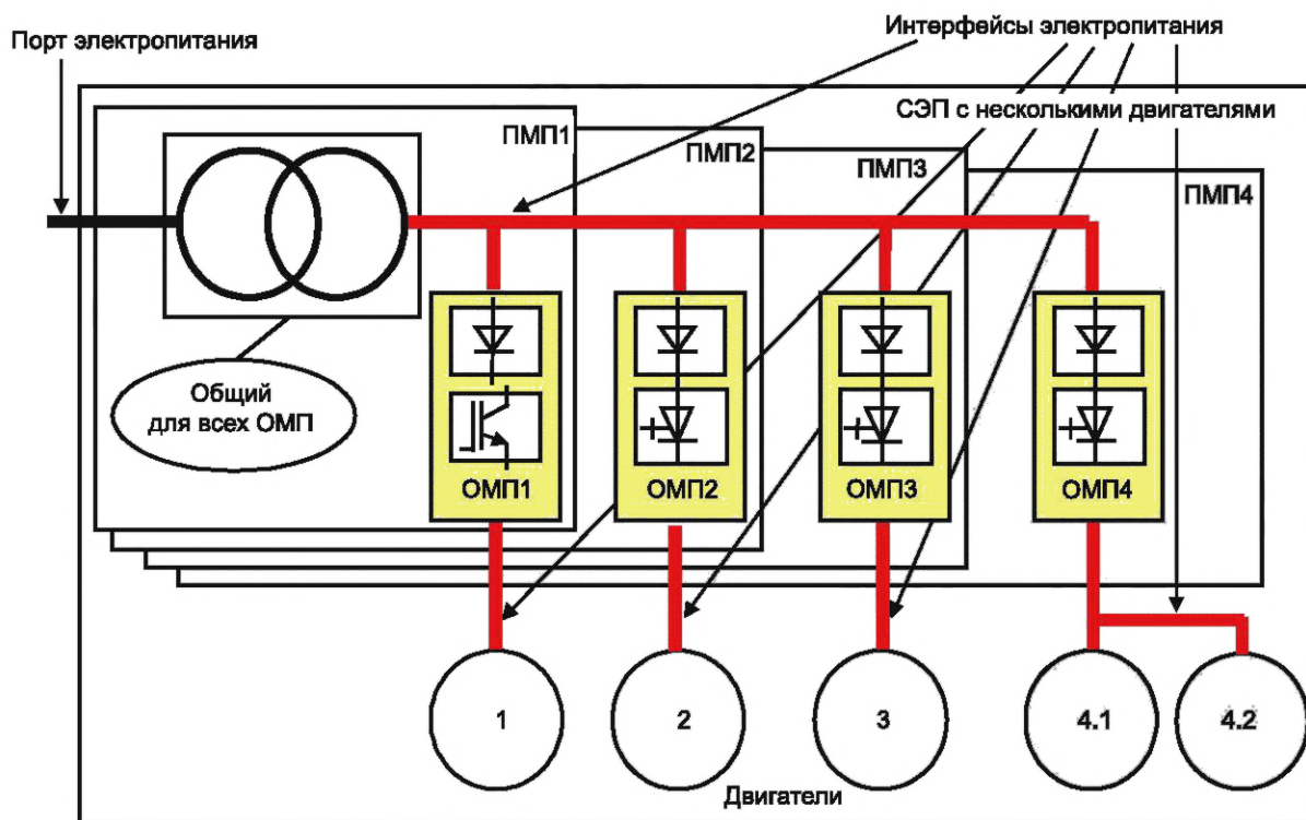
Рисунок 4 — Интерфейсы электропитания с общим входным трансформатором
