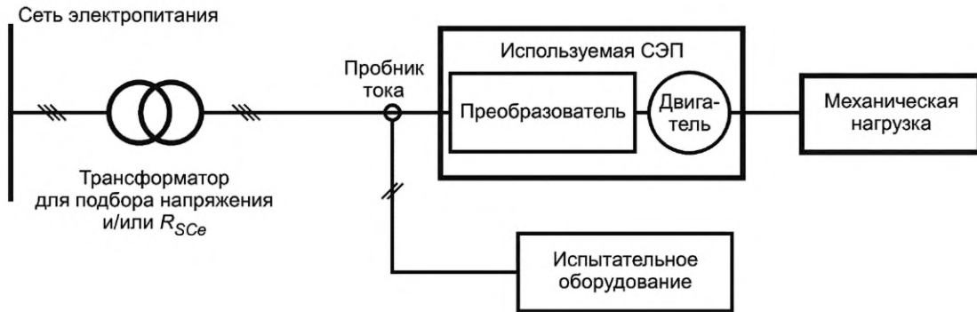
Рисунок В.5 — Испытательная установка с механической нагрузкой
