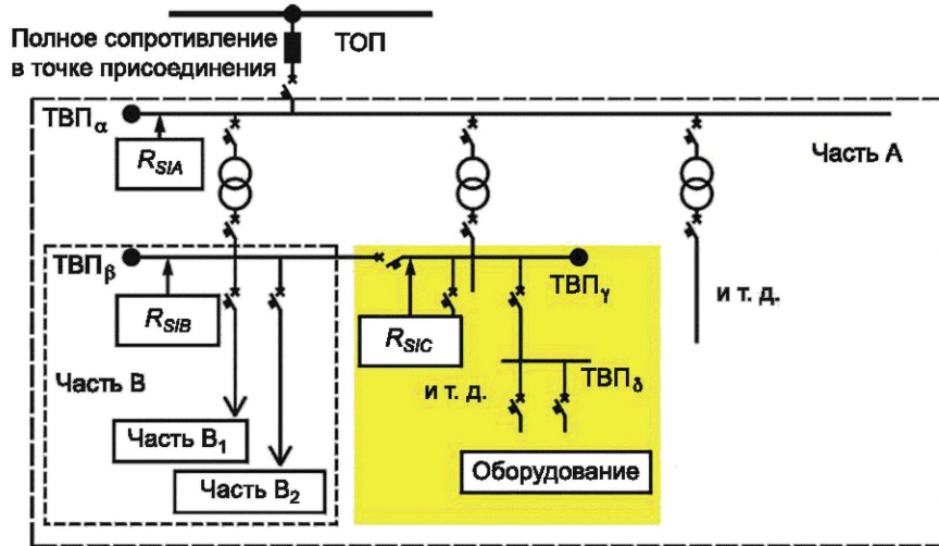
Рисунок В.2 — ТОП, ТВП, отношение тока установки и R_{SI}
