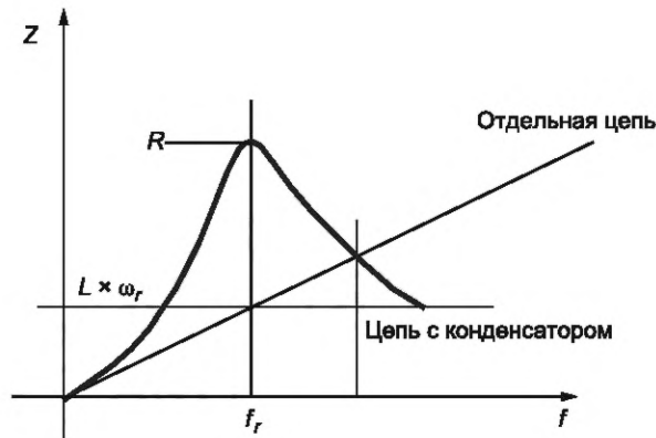
Рисунок С.3 — Полное сопротивление в зависимости от частоты при упрощенной схеме сети
