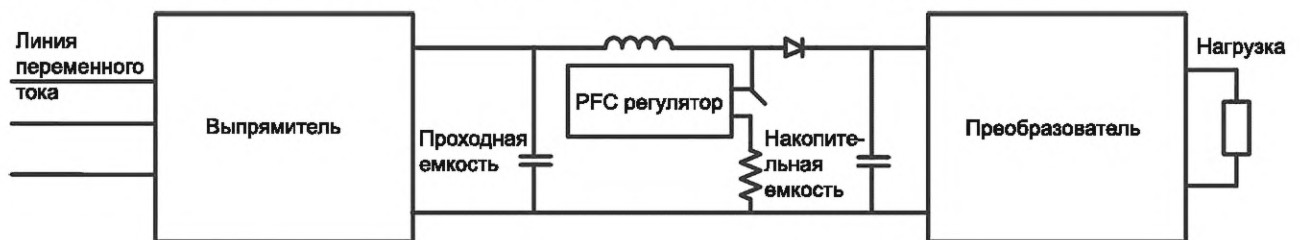
Рисунок С.7 — Повышающий преобразователь
