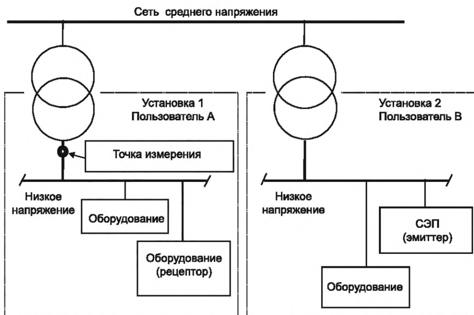
Рисунок 8 — Распространение помех
