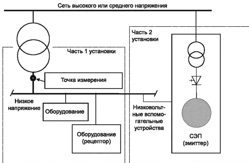
Рисунок 9 — Распространение помех в установке, включающей в себя СЭП номинальным напряжением свыше 1000 В
