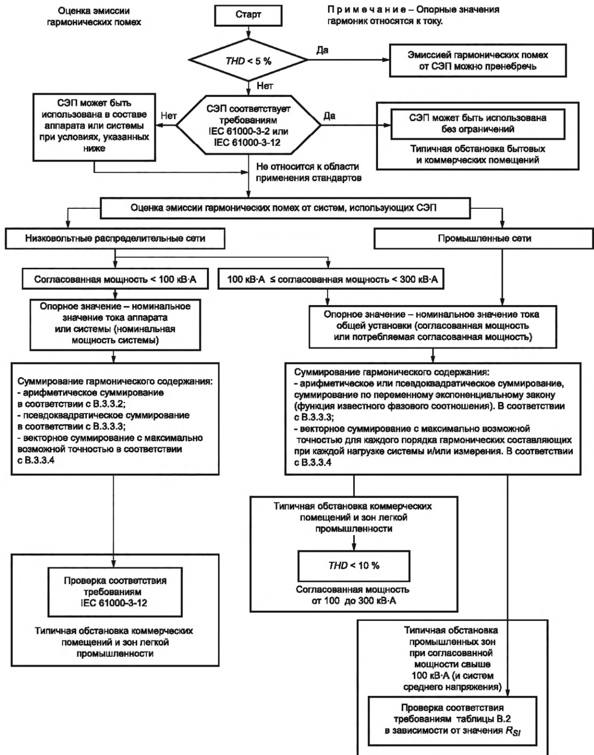
Рисунок В.8 — Оценка эмиссии гармонических помех при использовании СЭП (аппаратов, систем или установок)
