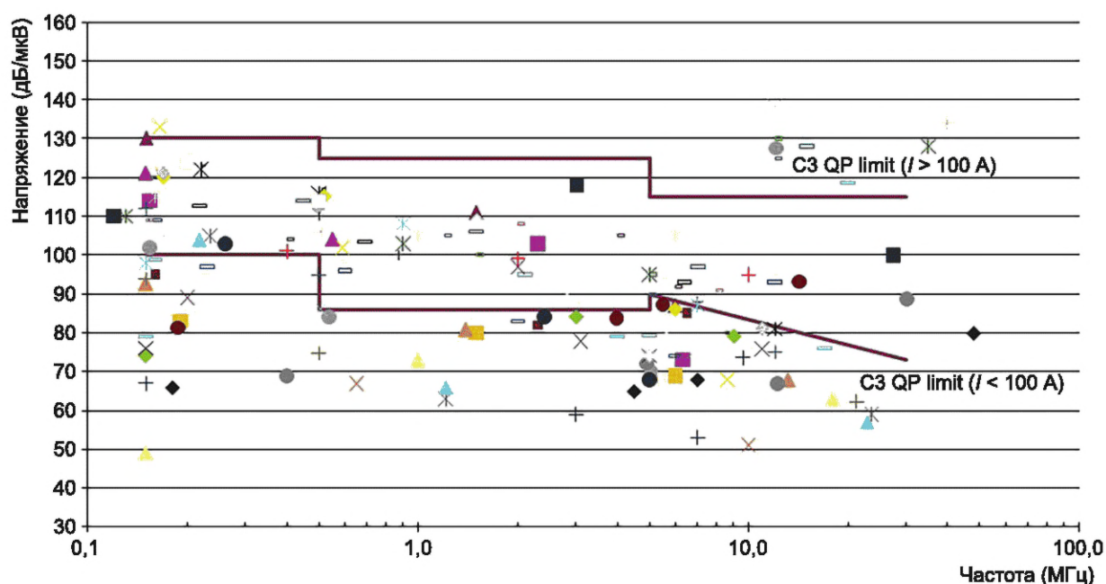
Рисунок D.1 — Кондуктивные помехи, создаваемые различными СЭП, не оборудованными фильтрами
