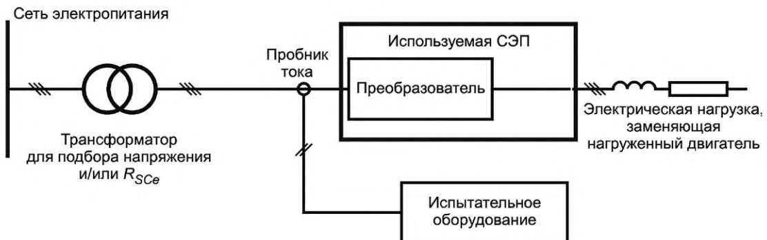
Рисунок В.6 — Испытательная установка с электрической нагрузкой, заменяющей нагруженный двигатель
