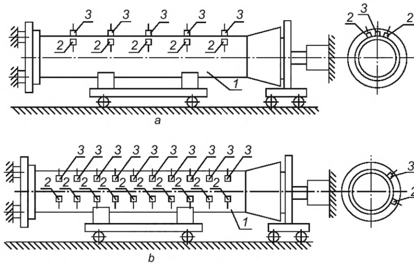
Рисунок 1 — Испытательный стенд
