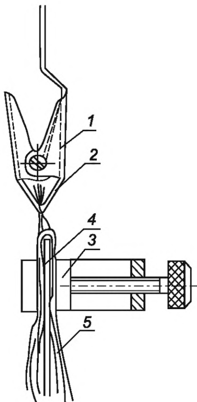
1 — верхний зажим; 2 — губки верхнего зажима; 3 — нижний зажим; 4 — планка; 5 — испытываемая проба
