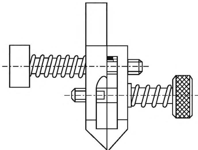
Рисунок А.1 — Верхний зажим для закрепления пучка волокон
