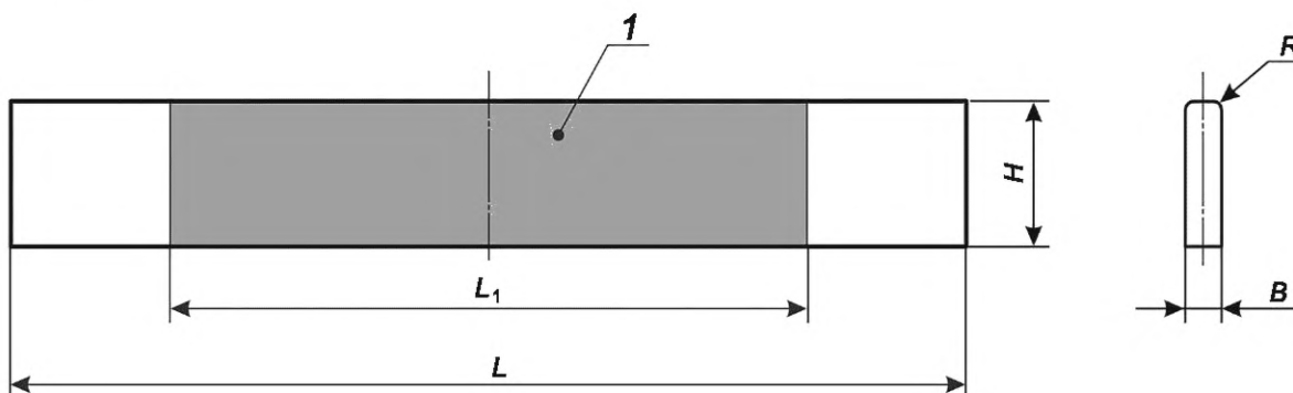
1 — центральная зона доски упора; L — длина внутренней части тэбилик между опорами; L_1 — длина центральной зоны доски упора; H — высота тэбилик; B — ширина доски упора; R — радиус закругления доски упора
