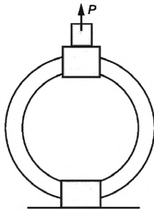
Рисунок 7 — Схема определения прочности тогурук мас
