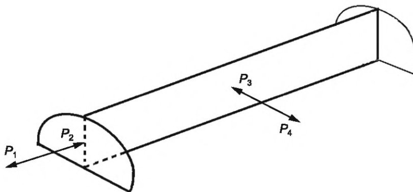
Рисунок 9 — Схема определения прочности крепления боковых опор тэбилик
