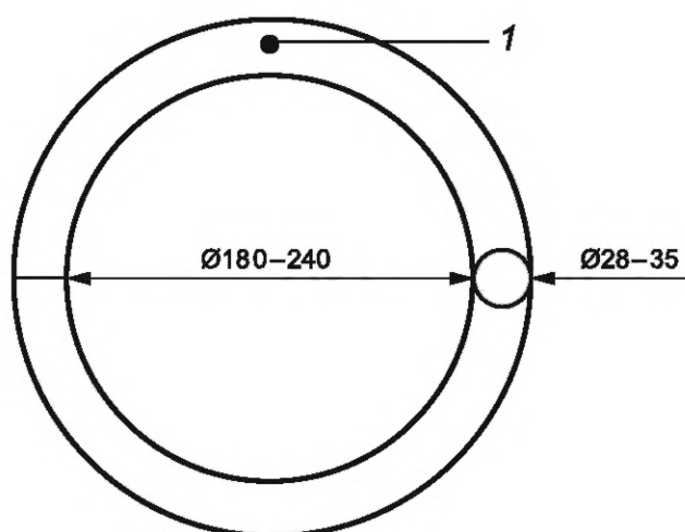
Рисунок 2 — Схема тогурук мас
