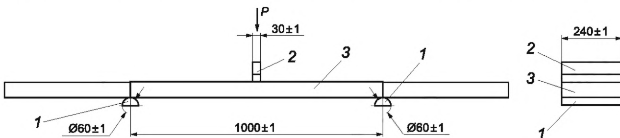
Рисунок 8 — Схема определения прочности доски упора
