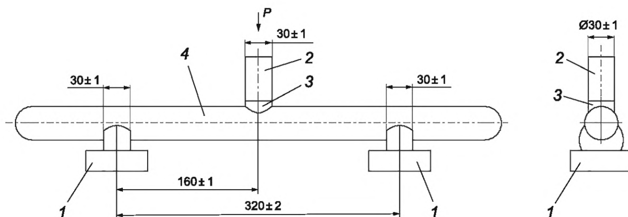
1 — шаровая опора; 2 — шток; 3 — резиновая проставка; 4 — мас; P — прикладываемая нагрузка
