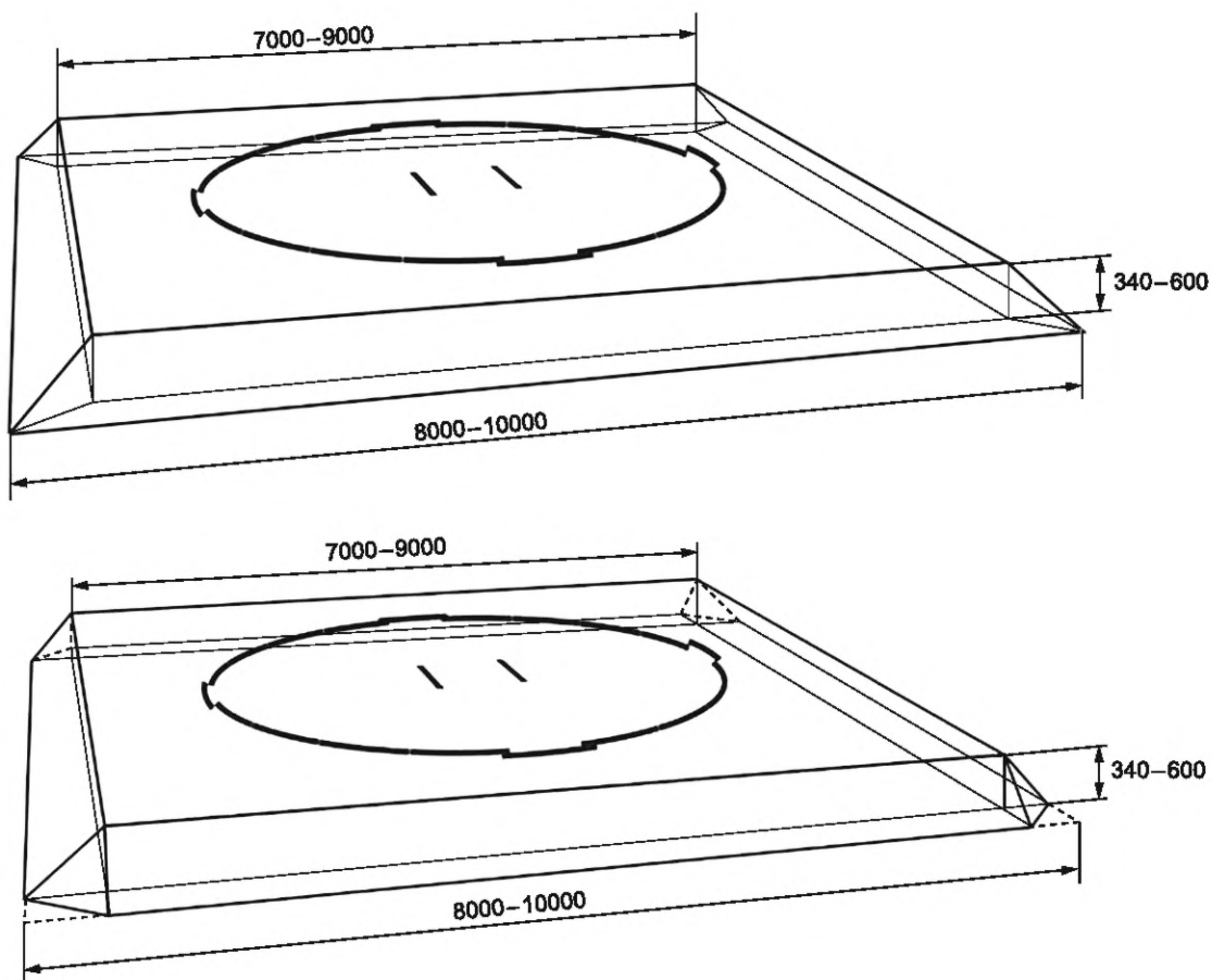
Рисунок 2 — Схема мори-дохё с двумя видами исполнения
