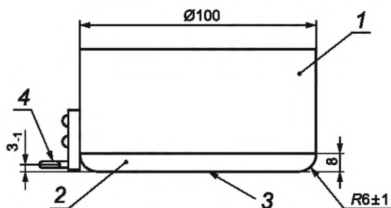
1 — цилиндр; 2 — каучуковый диск; 3 — трущаяся поверхность; 4 — проушина
