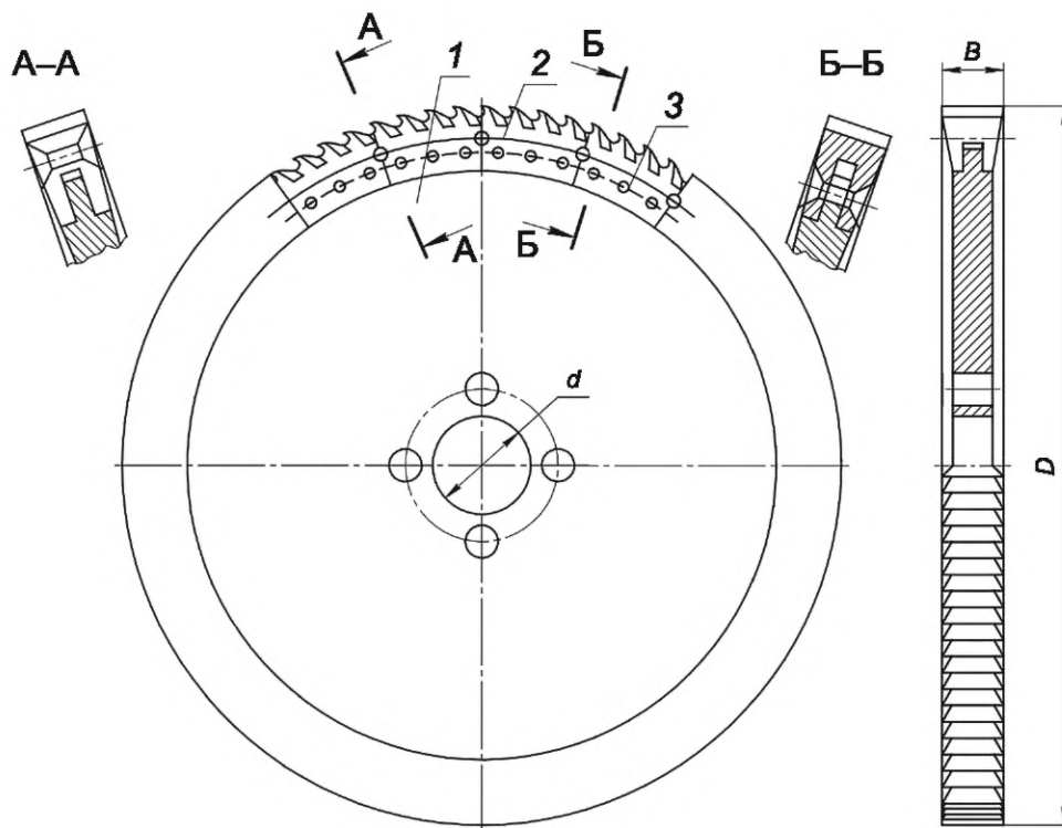
1 — диск; 2 — сегмент; 3 — заклепка
