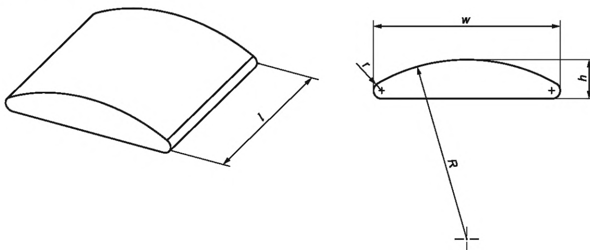
Рисунок Е.1 — Нагрузочная подушка таза
