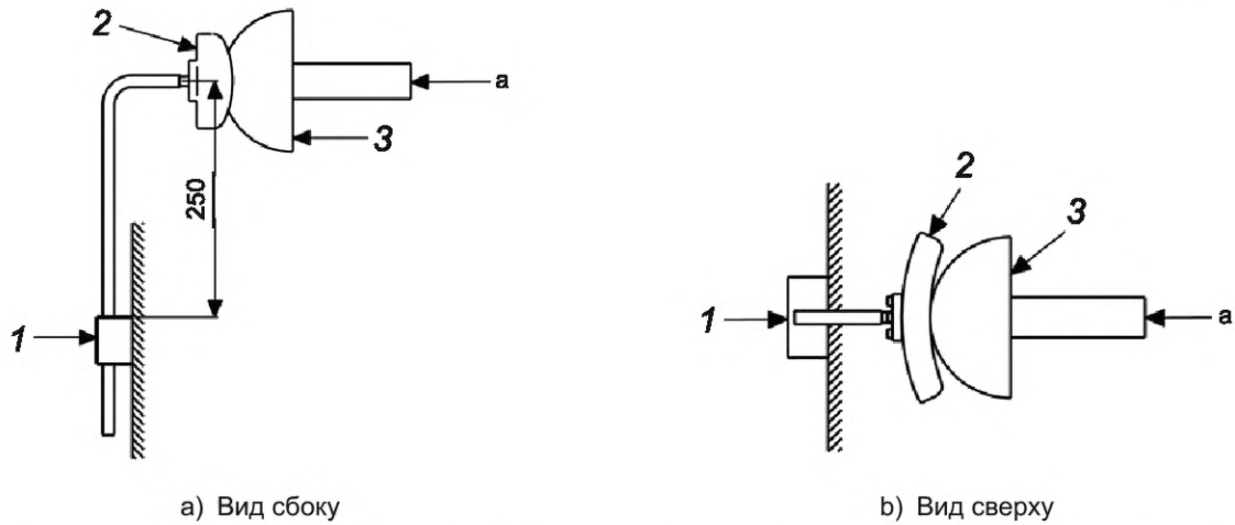
Рисунок В.4 — Пример приложения силы сзади к опоре головы
