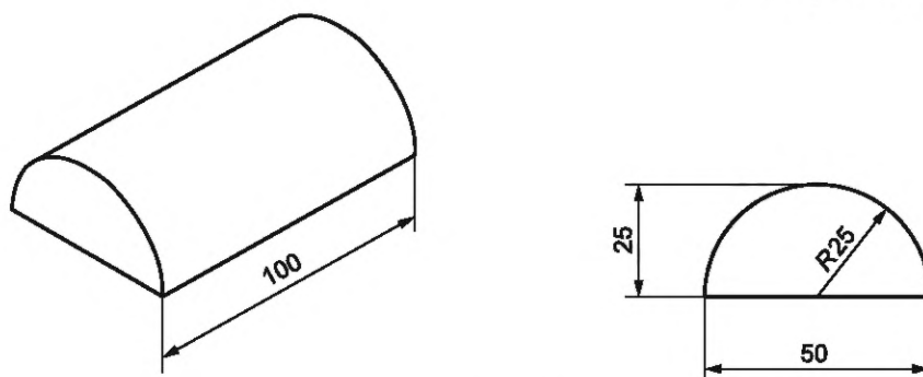
Рисунок Е.3 — Пример выпуклой нагрузочной подушки
