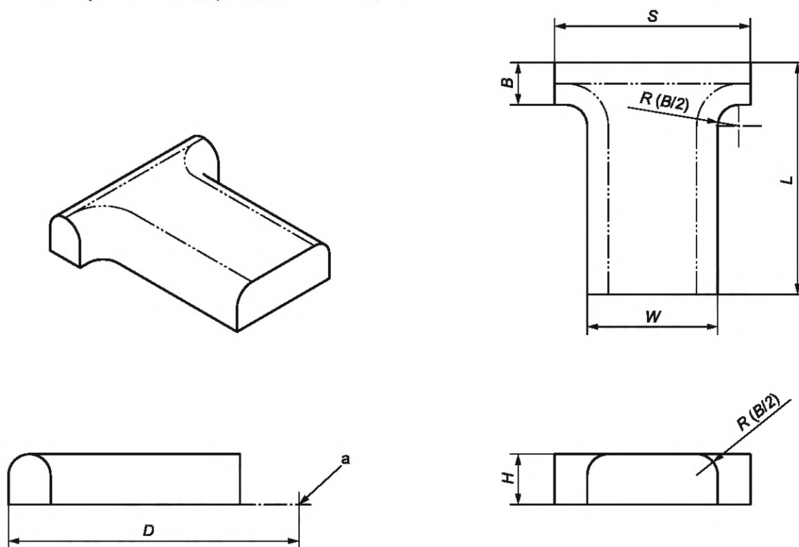
Рисунок Е.2 — Нагрузочная подушка туловища (размеры приведены в таблице Е.2)
