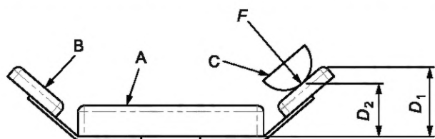
Рисунок В.2 — Пример приложения силы к невстроенной боковой опоре туловища
