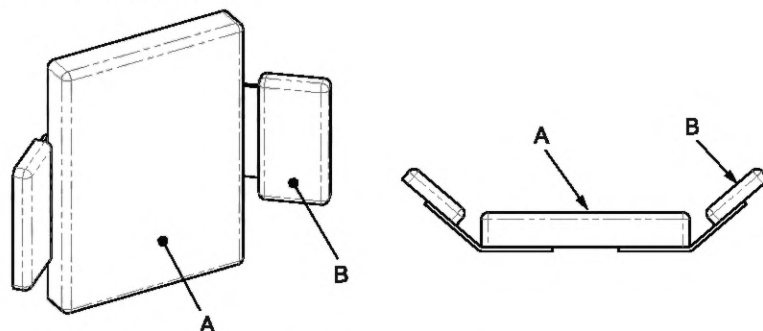
А — опора для спины; В — невстроенная боковая опора туловища
