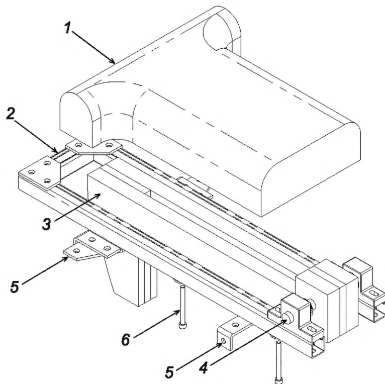
Рисунок D.2 — Поворотная испытательная рама и нагрузочная подушка для туловища
