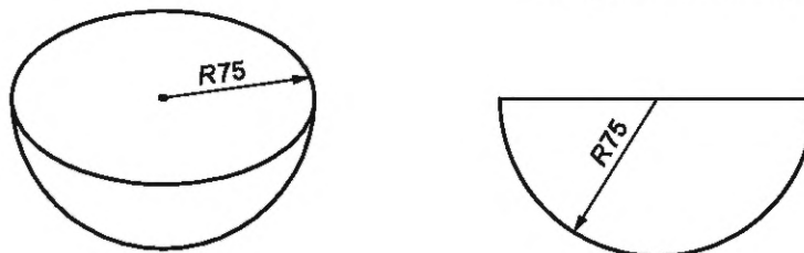
Рисунок Е.5 — Пример выпуклой полусферической нагрузочной подушки
