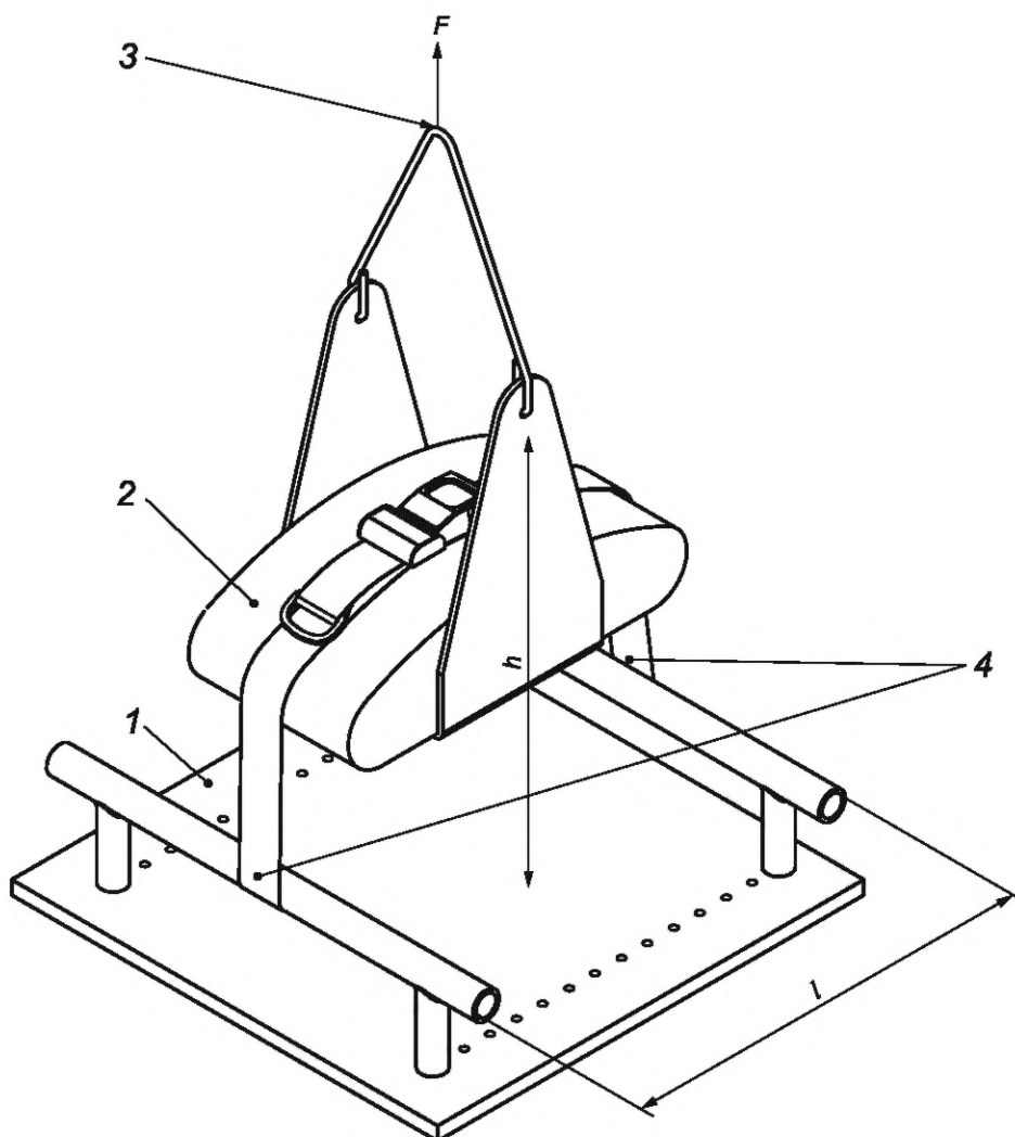
1 — регулируемая жесткая испытательная рама; 2 — выпуклая нагрузочная подушка таза; 3 — средняя точка нагрузочной подушки; 4 — точки крепления; F — испытательная нагрузка; l — расстояние между точками крепления; h — измерение положения нагрузочной подушки
