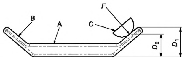
Рисунок В.1 — Пример приложения силы к встроенной боковой опоре туловища на опоре спинки
