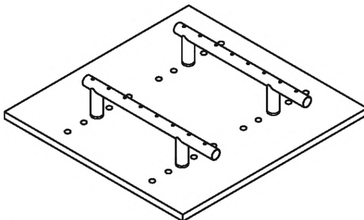
Рисунок D.1 — Пример регулируемой жесткой испытательной рамы с монтажными стержнями, прикрепленными параллельно основанию
