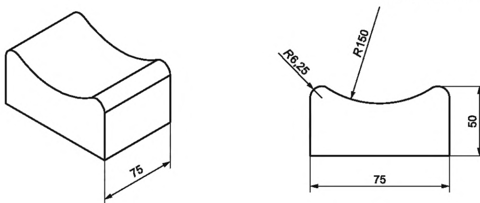
Рисунок Е.4 — Пример вогнутой нагрузочной подушки
