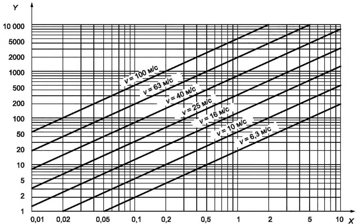
Рисунок А.4 — Зависимость абсолютной энергии от массы и скорости поступательного движения частицы
