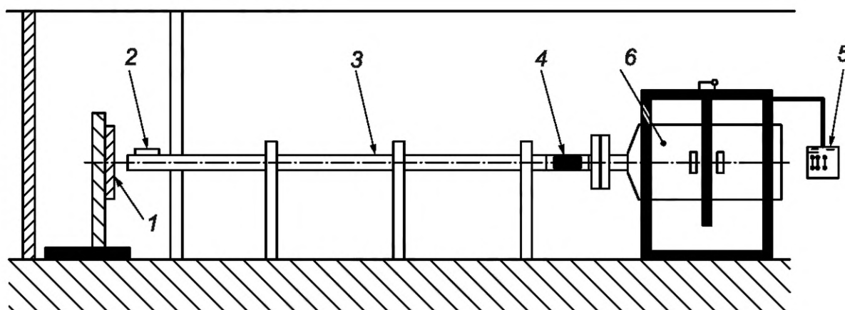
1 — объект испытаний; 2 — датчик скорости; 3 — ствол пушки; 4 — ударник; 5 — панель управления; 6 — баллон сжатого воздуха
