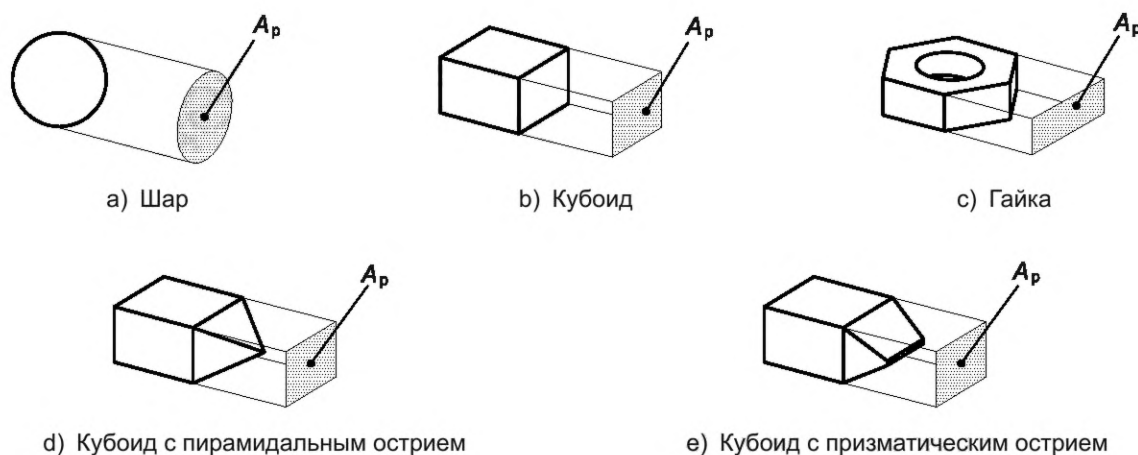
Рисунок А.2 — Минимальная площадь проекции для тел разной формы
