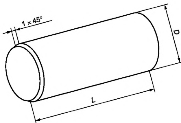
Рисунок А.3 — Стандартный ударник тупоголовой формы (изготовлен из стали твердостью 40—50 единиц по шкале Роквелла)
