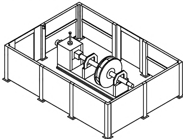
Рисунок С.1 — Ограждение для горизонтального балансирующего станка (класс защиты В)
