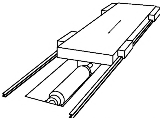
Рисунок С.5 — Прямо́к с кры́шкой для высо́коскоростного баланси́ровочного станка (класс защиты D, взрывозащищенный)
