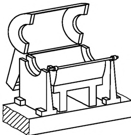
Рисунок С.2 — Кожух ротора для горизонтального балансирующего станка (класс защиты В или С)
