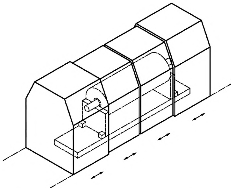
Рисунок С.3 — Телескопический кожух, полностью охватывающий балансировочный станок (класс защиты С)
