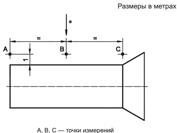
Рисунок 1 — Точки измерений согласно перечислению е)
