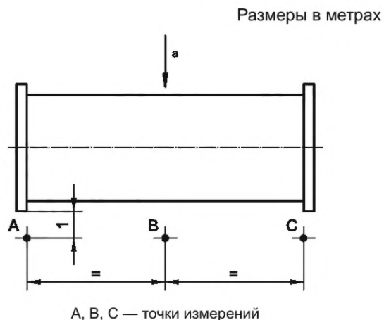
Рисунок 2 — Точки измерений согласно перечислению e)
