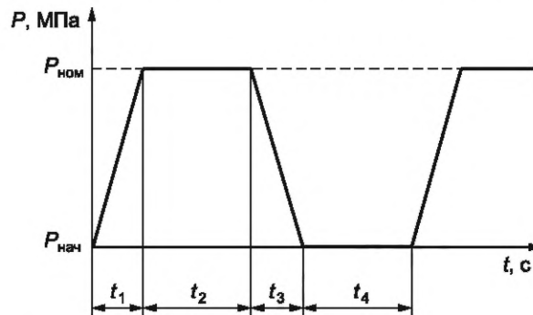
t_1 — время нарастания давления; t_2 — время выдержки фильтра под давлением; t_3 — время падения давления; t_4 — время выдержки фильтра под начальным давлением; P_{ном} — номинальное давление; P_{нач} — начальное давление
