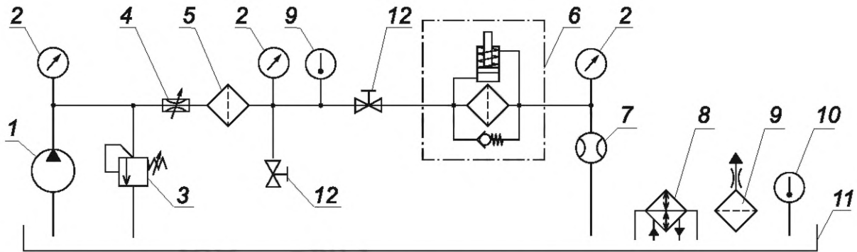
1 — насос; 2 — манометр; 3 — предохранительный гидроклапан; 4 — регулируемый гидродроссель; 5 — технологический фильтр; 6 — испытуемый фильтр; 7 — расходомер; 8 — теплообменный аппарат; 9 — сапун; 10 — термометр; 11 — гидробак; 12 — кран
