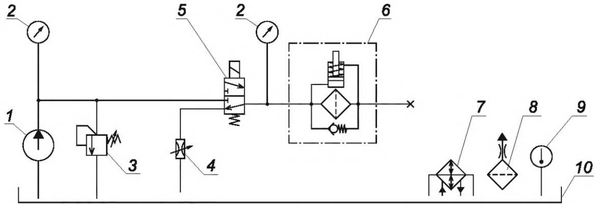
1 — насос; 2 — манометр; 3 — предохранительный гидроклапан; 4 — регулируемый гидродроссель; 5 — гидрораспределитель; 6 — испытуемый фильтр; 7 — теплообменный аппарат; 8 — салун; 9 — термометр; 10 — гидробак
