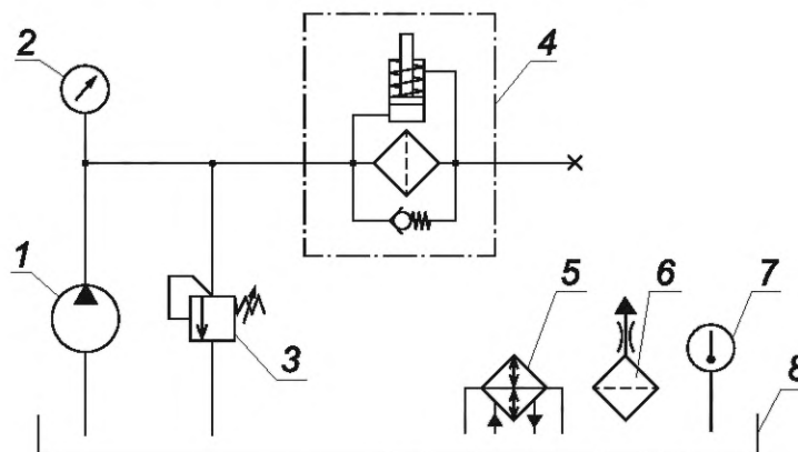
1 — насос; 2 — манометр; 3 — предохранительный гидроклапан; 4 — испытуемый фильтр; 5 — термометр; 6 — сапун; 7 — теплообменный аппарат; 8 — гидробак
