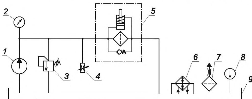
1 — насос; 2 — манометр; 3 — предохранительный гидроклапан; 4 — регулируемый гидродроссель; 5 — испытуемый фильтр; 6 — теплообменный аппарат; 7 — сапун; 8 — термометр; 9 — гидробак
