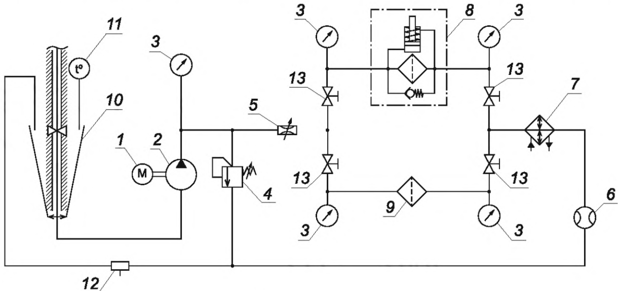
1 — электродвигатель; 2 — насос; 3 — манометр; 4 — предохранительный гидроклапан; 5 — регулируемый гидродроссель; 6 — расходомер; 7 — теплообменный аппарат; 8 — испытуемый фильтр; 9 — технологический фильтр; 10 — бак; 11 — термометр; 12 — пробоотборник; 13 — кран
