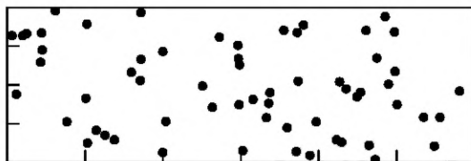
Рисунок А.6 — 4 % поверхности, 61 пора, d = 1 мм
