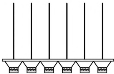
а) вариант 3: отсутствие интерференции максимумов звукового поля в дальней зоне
