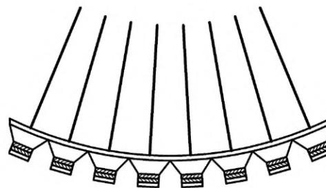
б) вариант 4: аддитивное наложение максимумов звукового поля в дальней зоне
