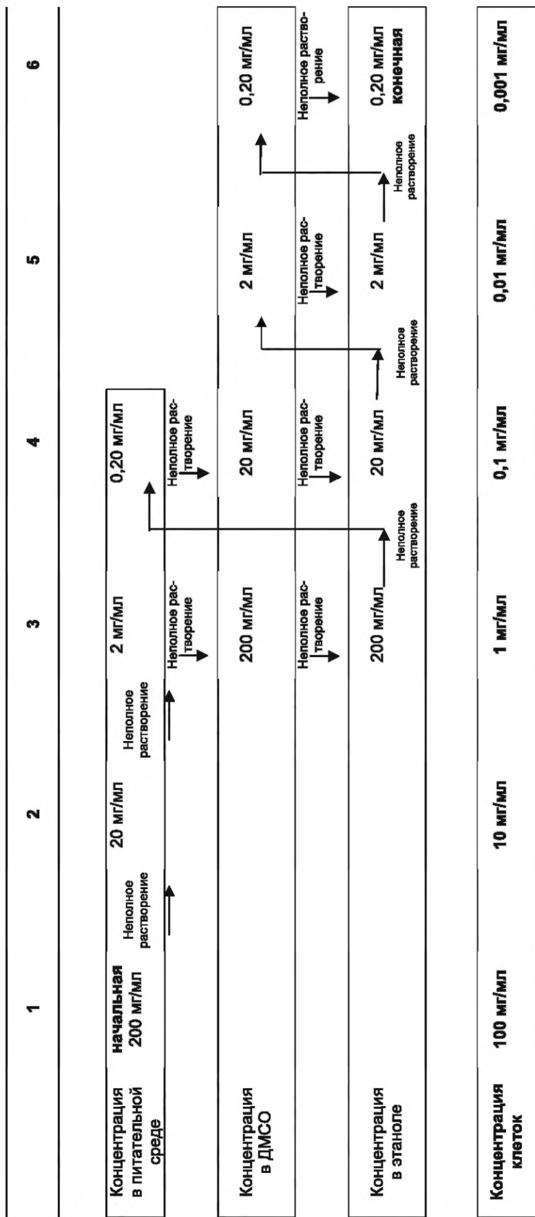
Рисунок Г.1 — Блок-схема для определения растворимости исследуемого вещества в питательной среде, диметилсульфоксиде (ДМСО) или этаноле
