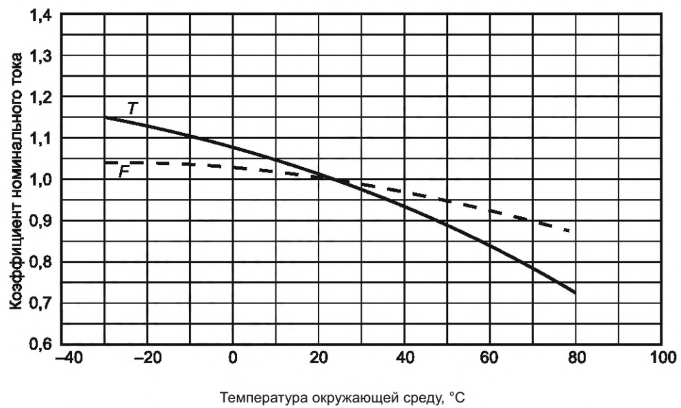
Рисунок С.2 — Пример повторного определения номинального тока плавкой вставки
