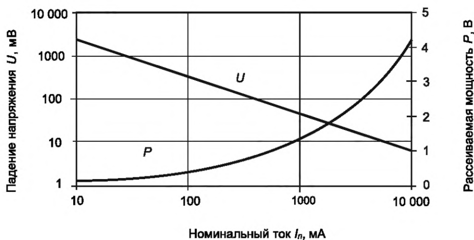
Рисунок С.1 — Пример рассеиваемой мощности и падения напряжения в зависимости от номинального тока
